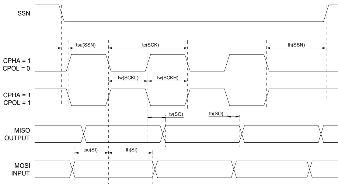
图 7-6 SPI 时序图 (从机模式 cpha=1)
