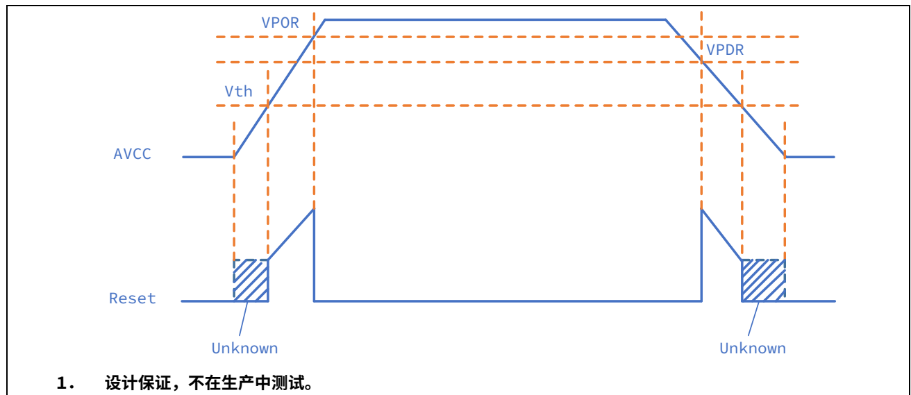
图 7-1 POR/PDR 示意图
