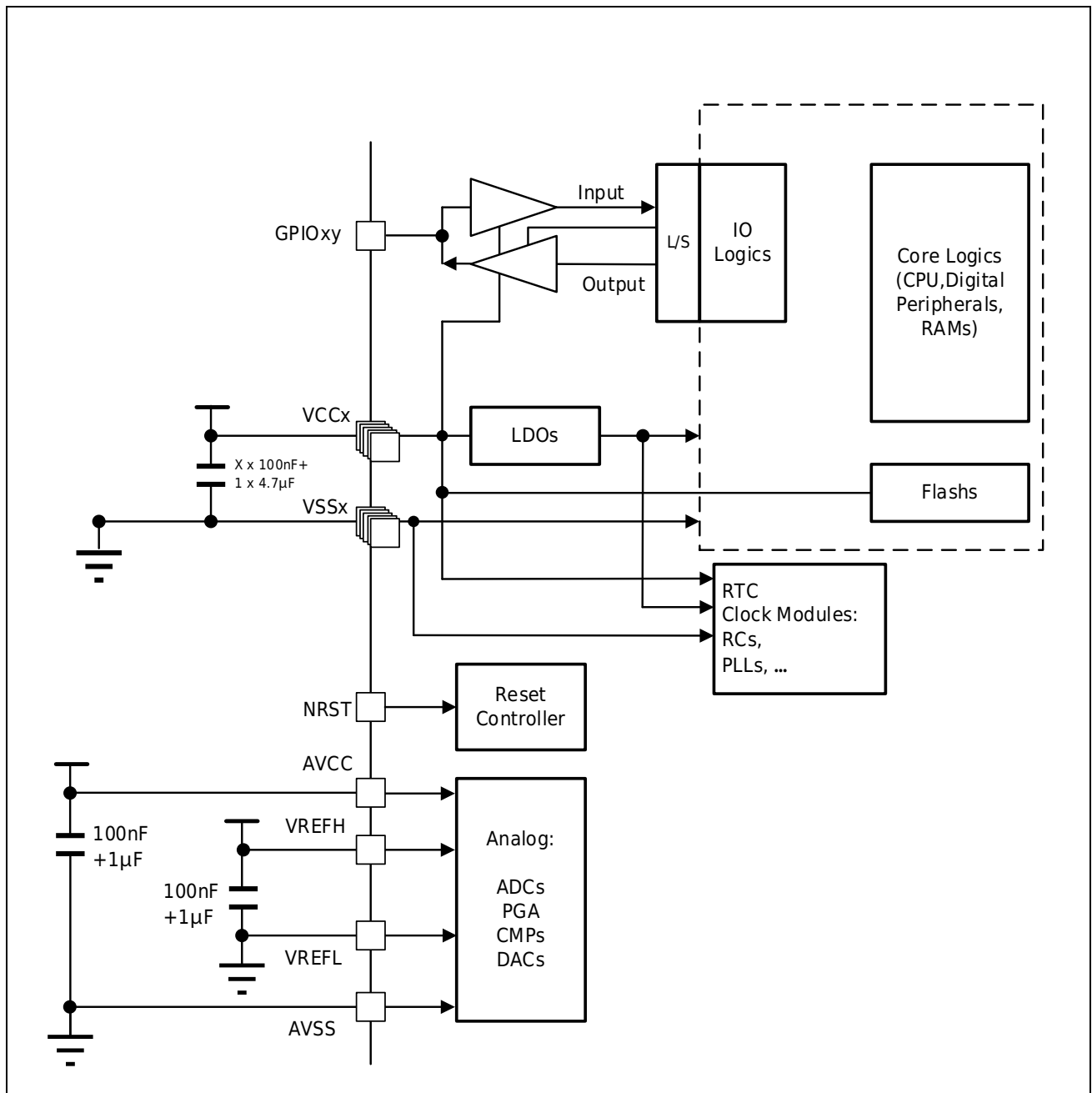
图 3-2 电源方案
