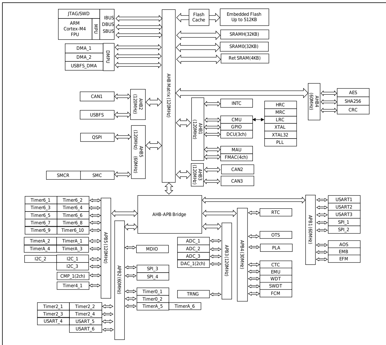
图 1-2 功能框图
