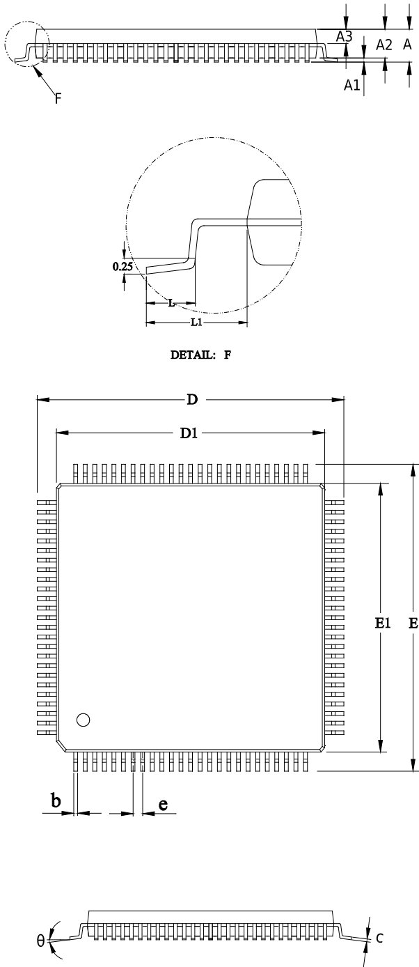
LQFP100 封装
