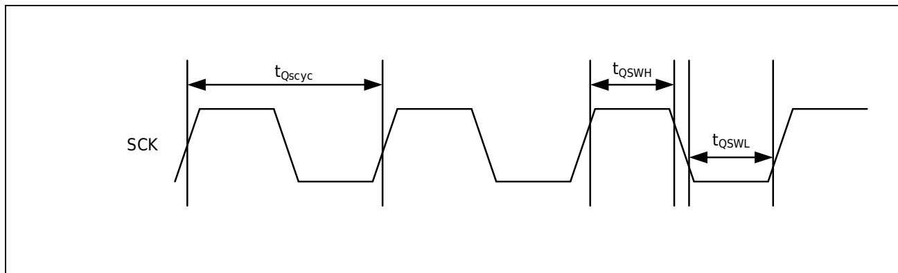
图 3-12 QSPI 时钟时序
