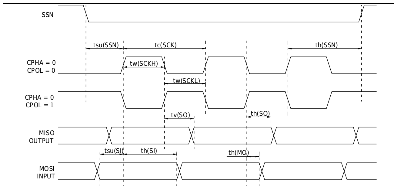
图 7-5 SPI 时序图（从机模式 cpha=0）
