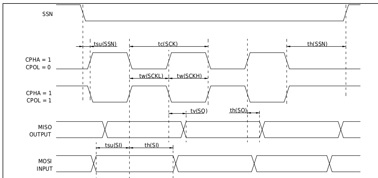
图 7-6 SPI 时序图 (从机模式 cpha=1)
