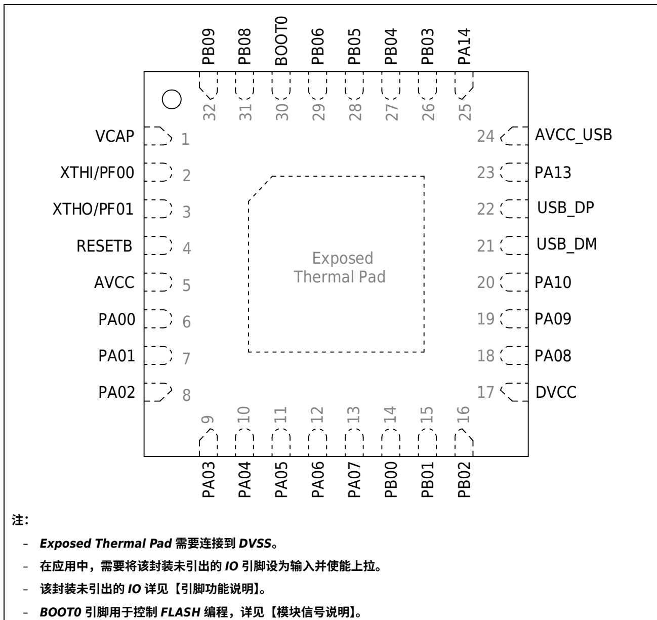
图 3-1 引脚配置图
