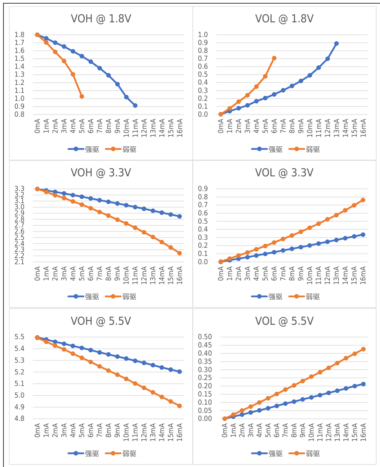
图 7-2 输出端口 VOH/ VOL 实测曲线
