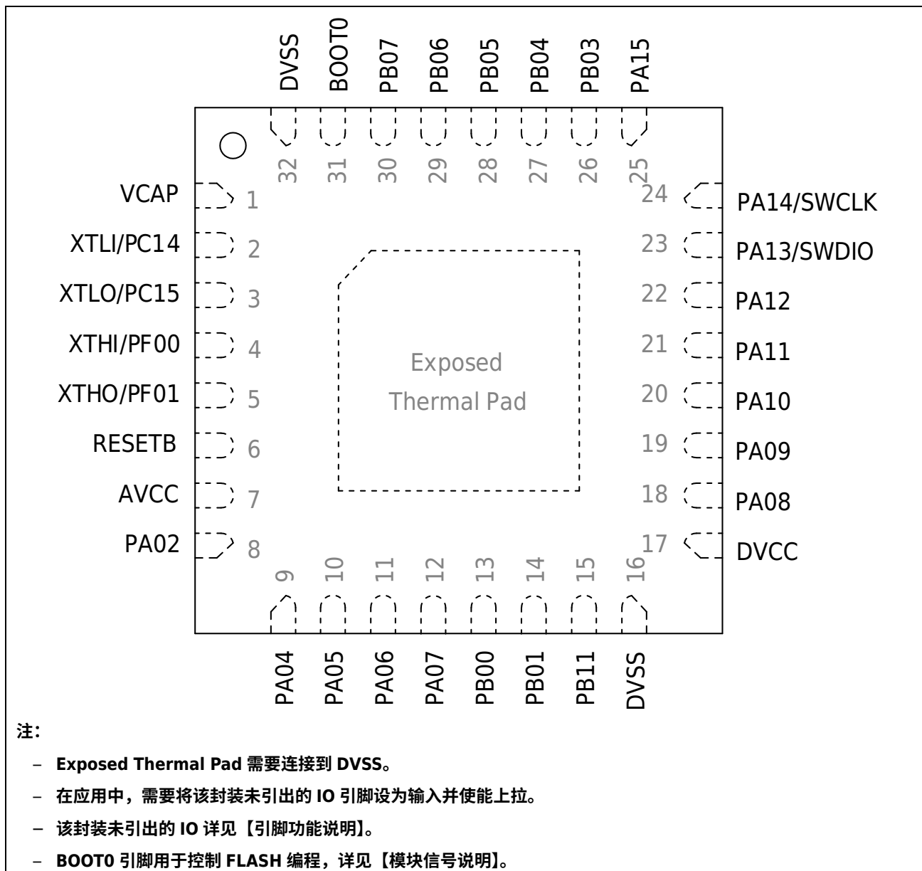
图 3-1 引脚配置图
