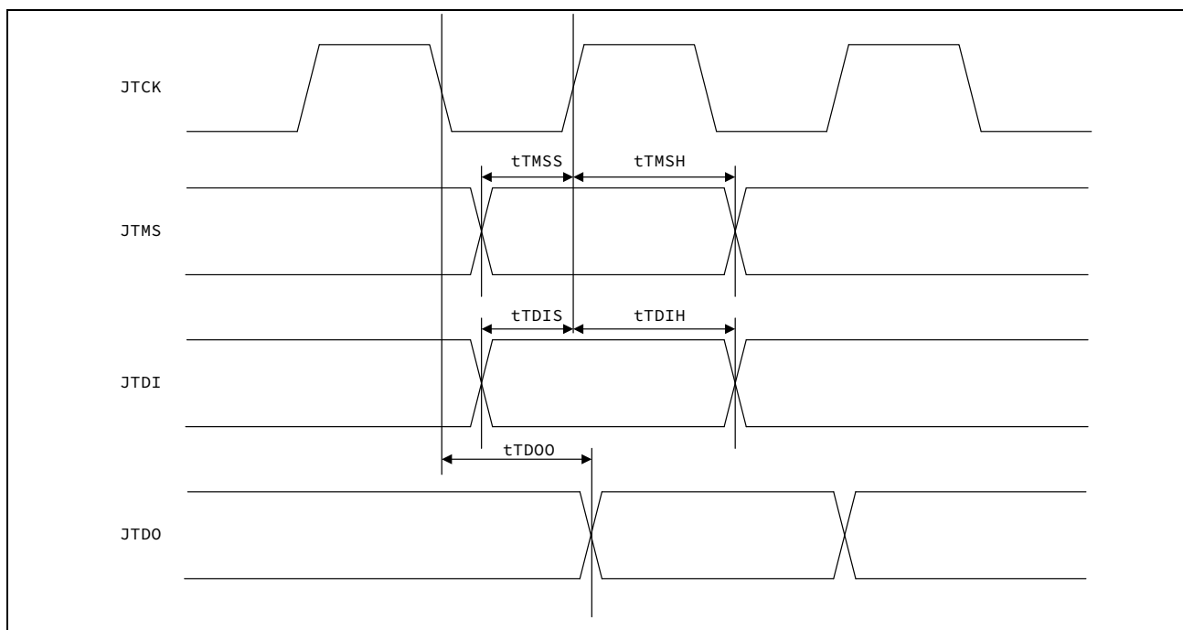
图 3-25 JTAG TCK 时钟
