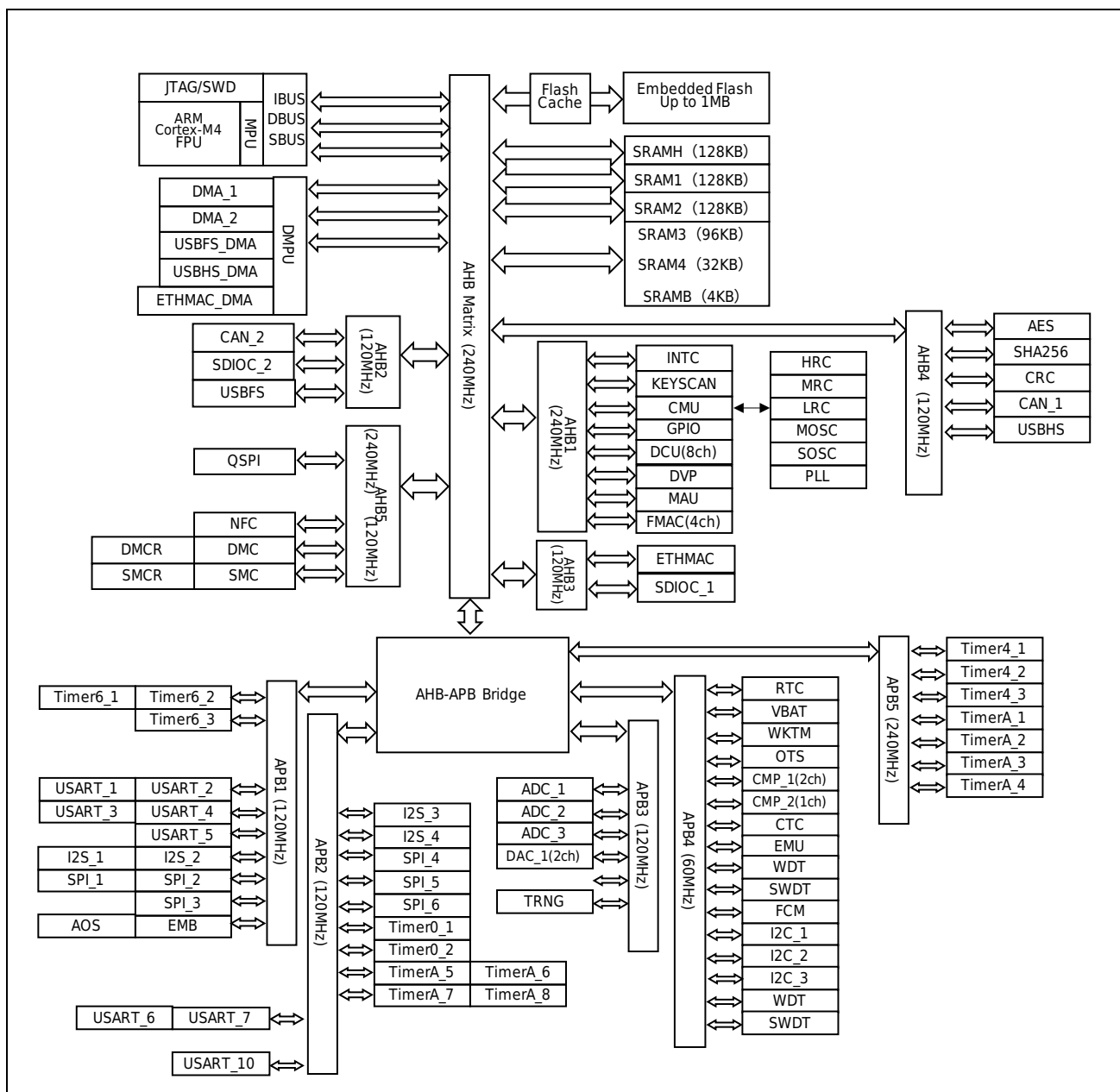
图 1-1 功能框图
