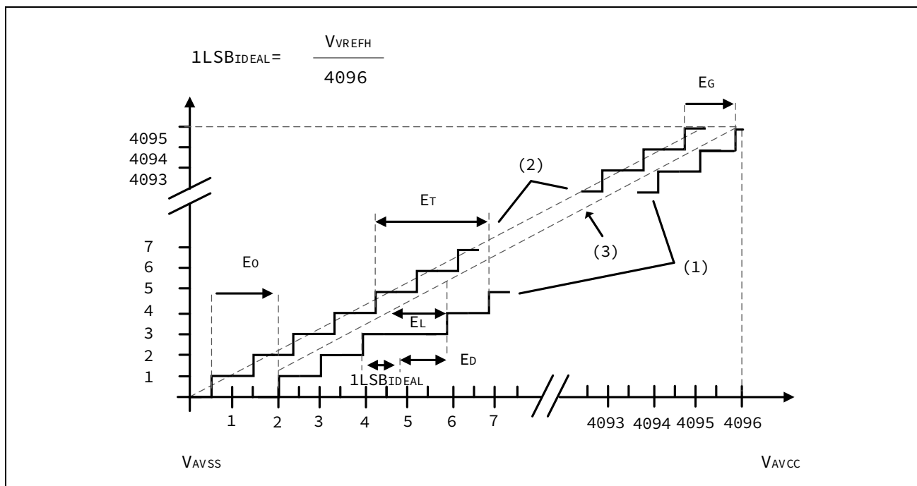
图 3-31 ADC 精度特性
