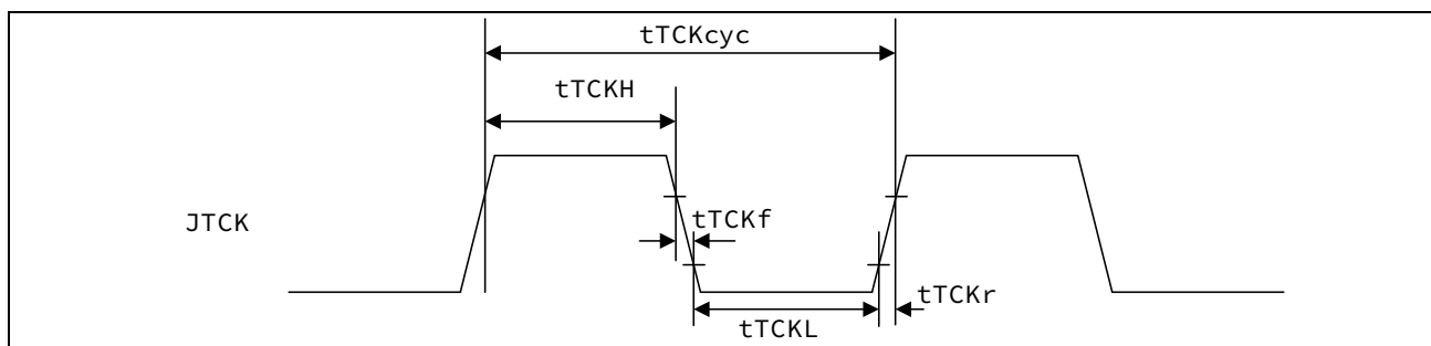
图 3-25 JTAG TCK 时钟
