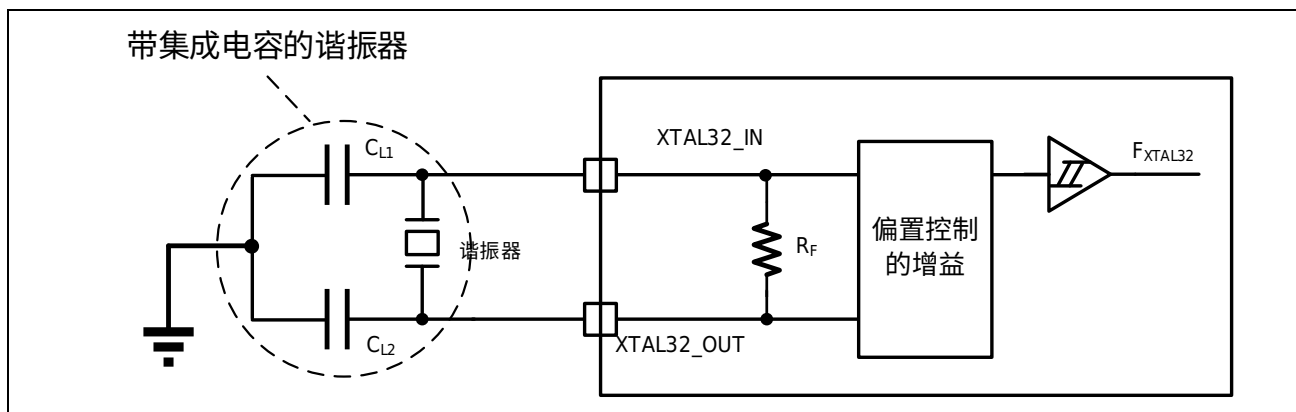
图 3-5 采用 32.768kHz 晶振的典型应用
