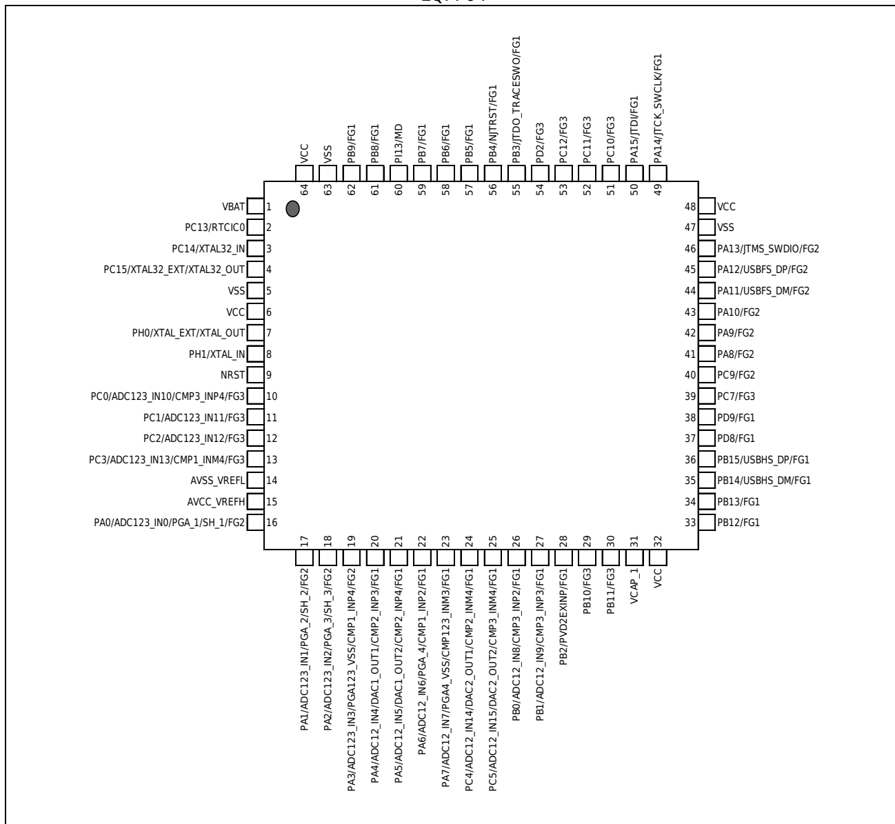
图 2-1 引脚配置图
