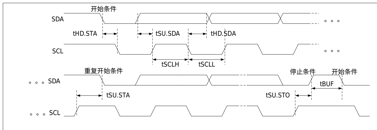
图 7-3 I2C 接口时序
