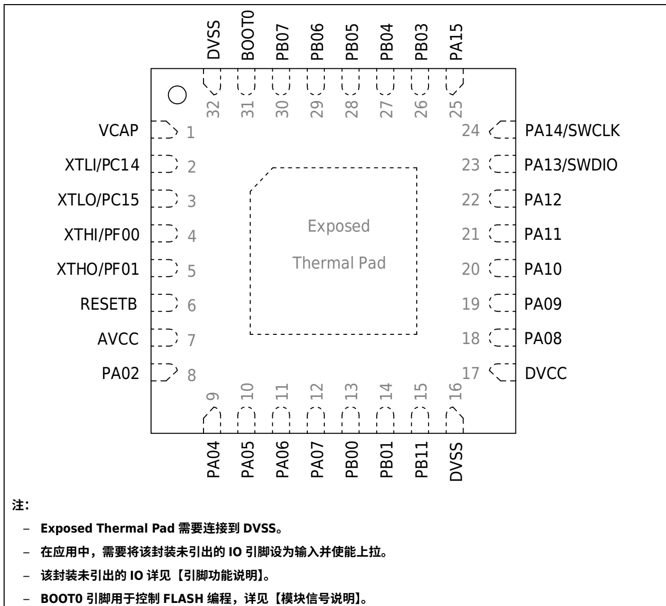
图 3-1 引脚配置图
