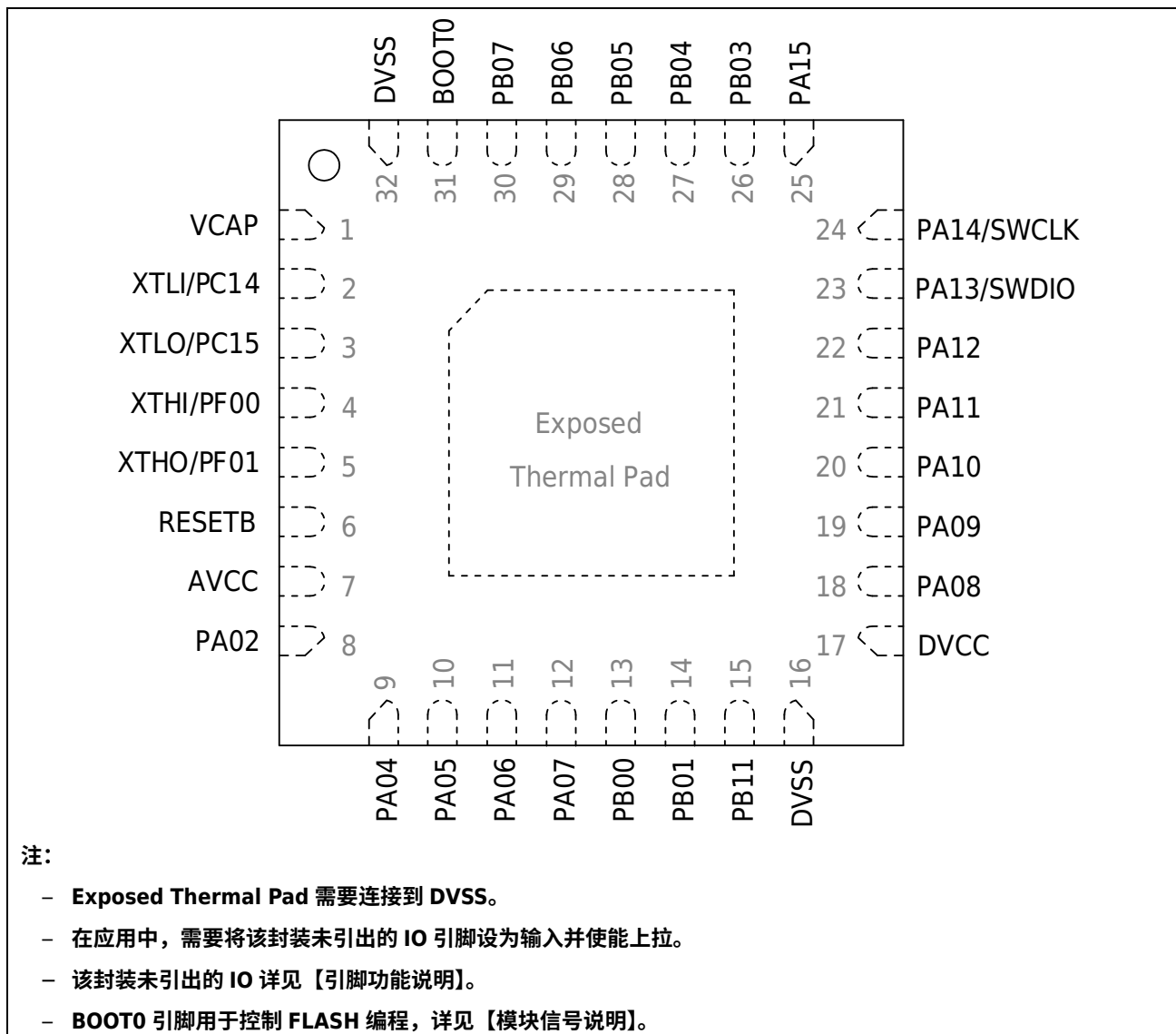
图 3-1 引脚配置图
