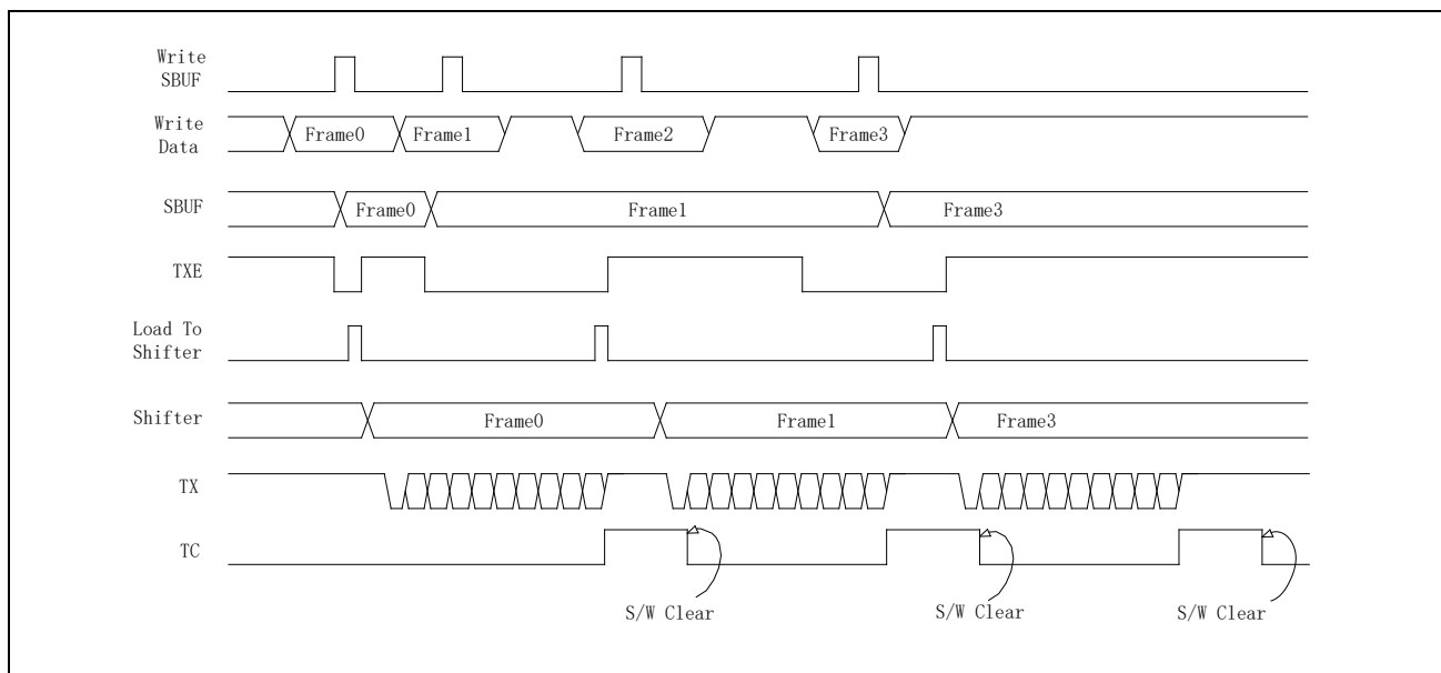
图 22-14 发送缓存
