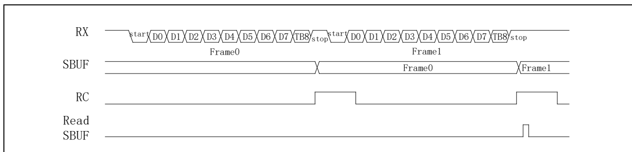
图 22-13 接收缓存
