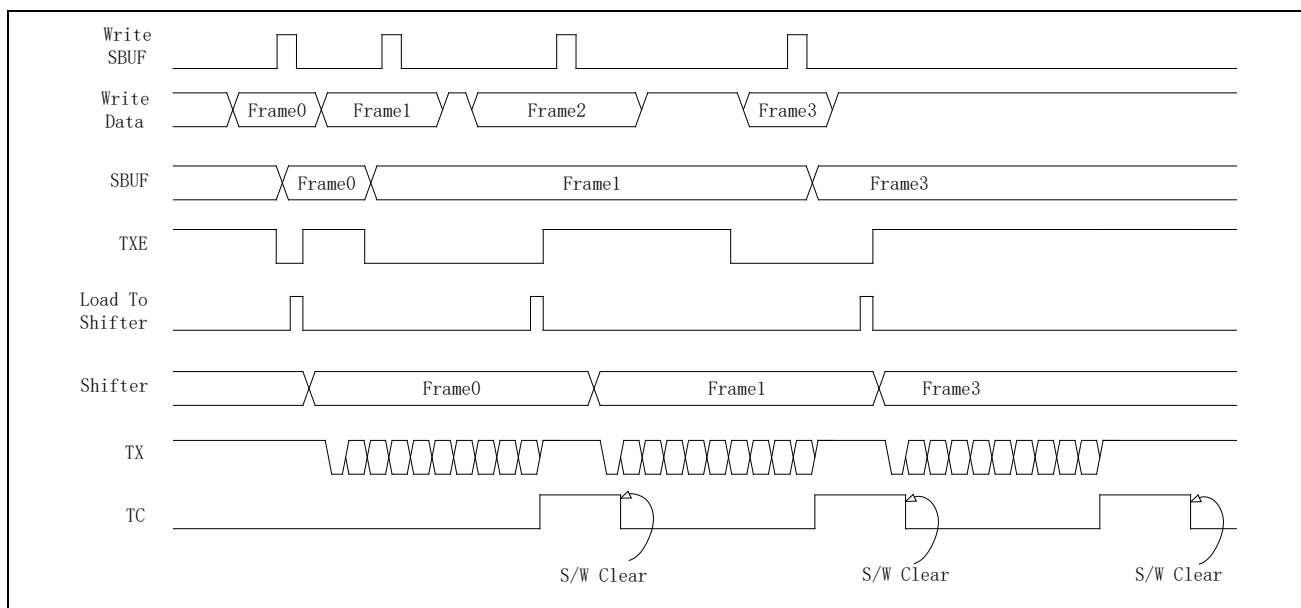
图 21-14 发送缓存
