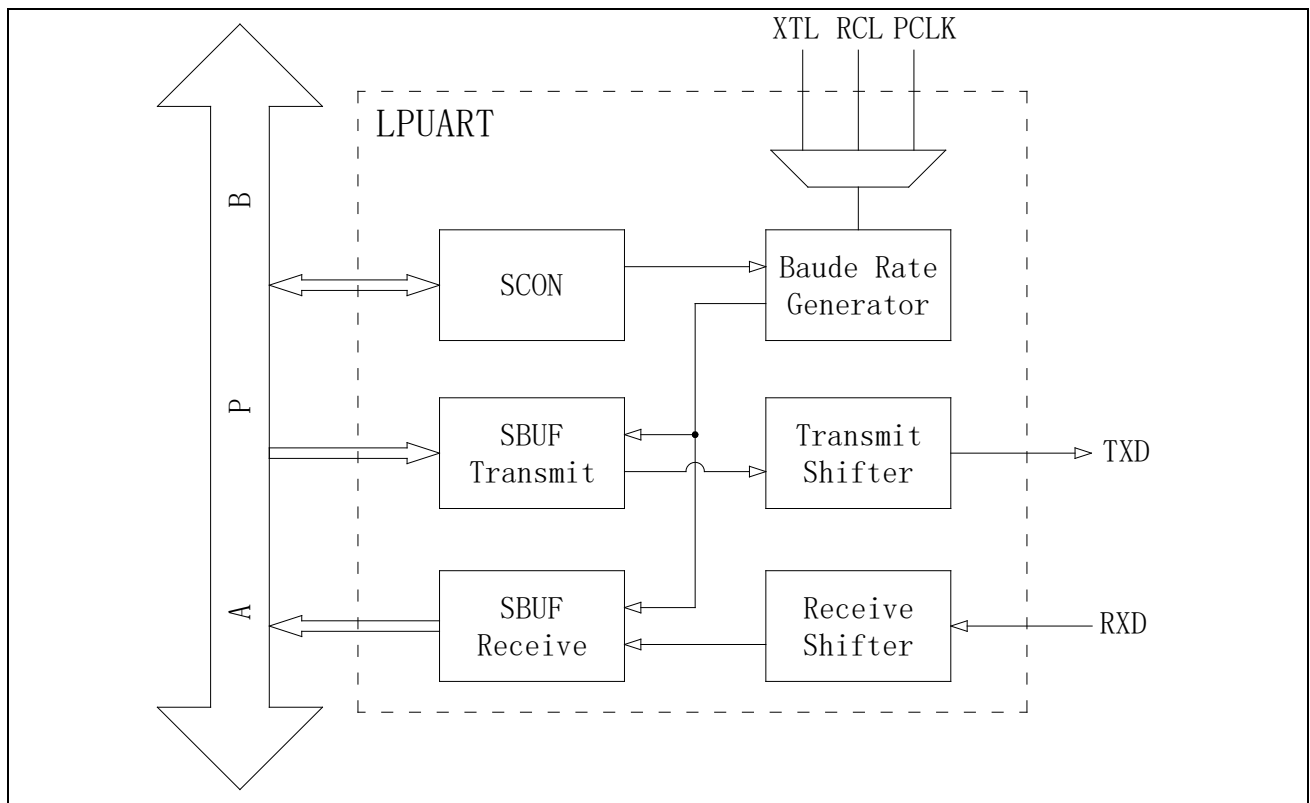
图 22-1 结构框图
