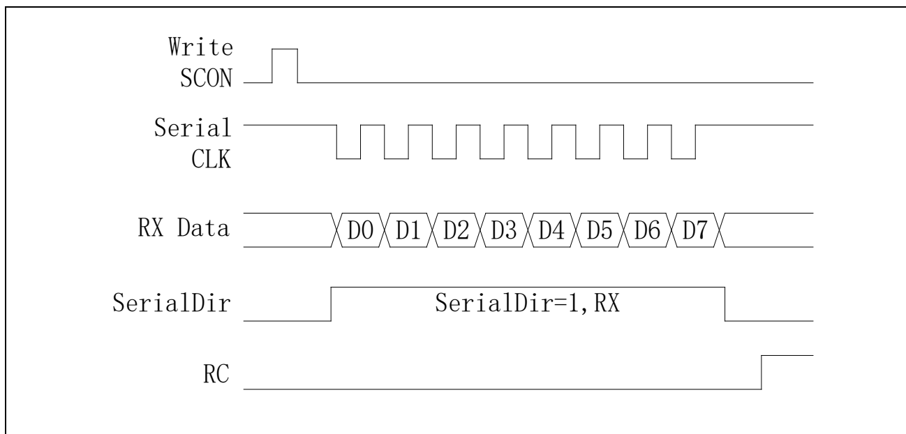
图 21-3 Mode0 接收数据
