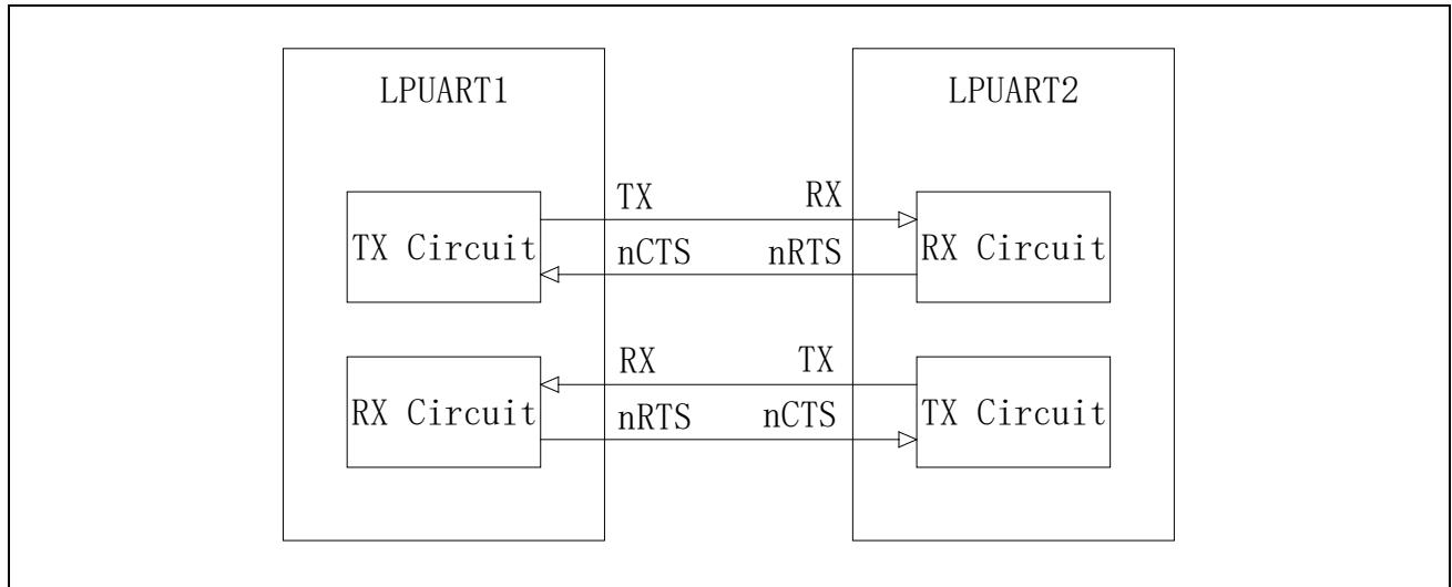
图 22-10 LPUART 硬件流控
