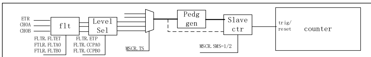
图 14-53 触发和复位功能
