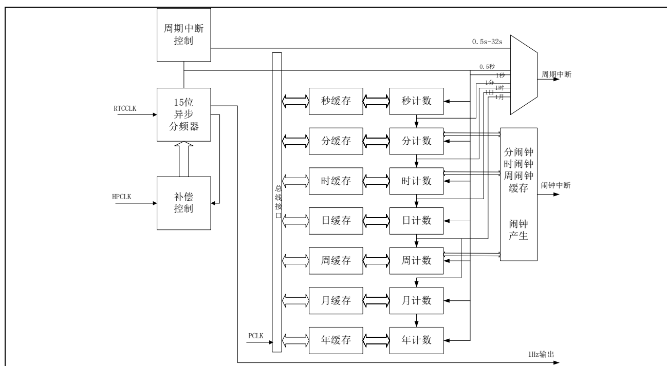
图 18-1 RTC 框图
