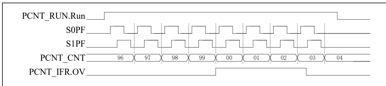
图 20-6 双通道正交脉冲计数模式加计数波形
