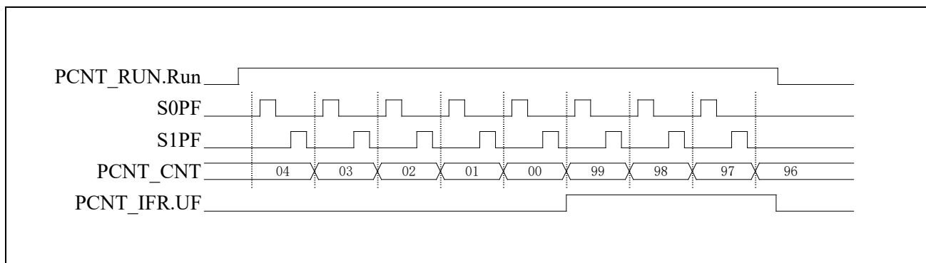
图 20-5 双通道非交脉冲计数模式减计数波形
