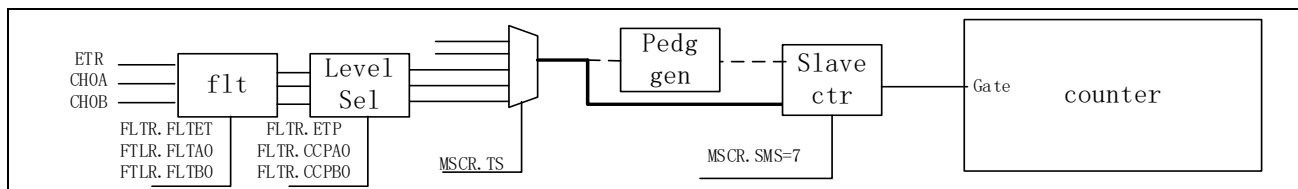
图 14-52 门控功能
