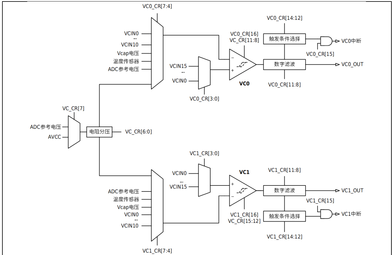
图 28-1 VC 框架图
