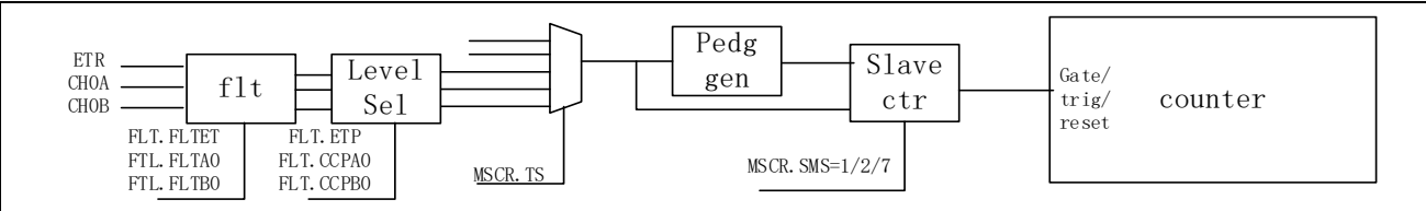
图 14-51 从模式示意图
