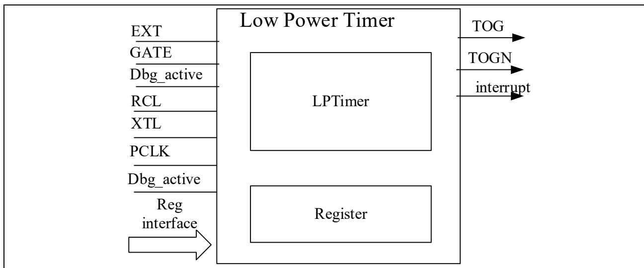
图 15-1 LPTimer 框图
