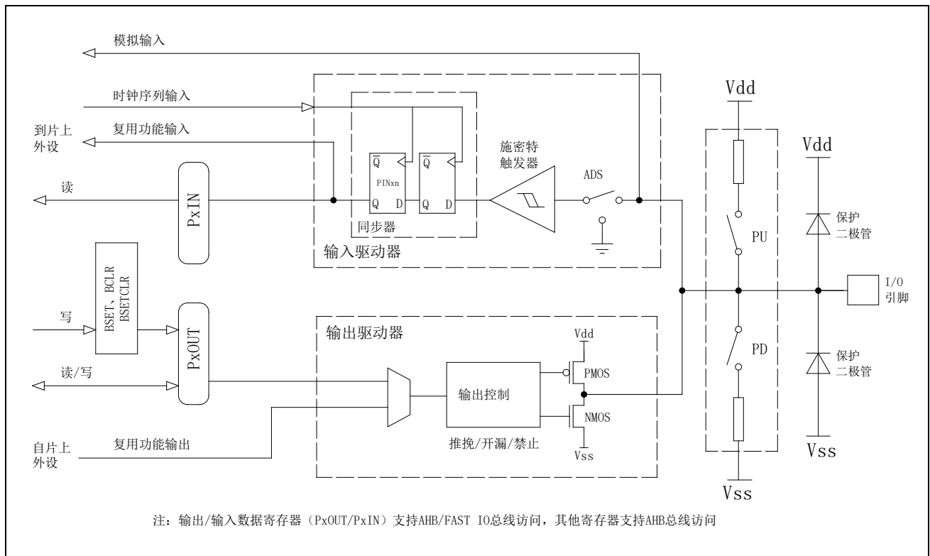
图 6-1 端口电路图
