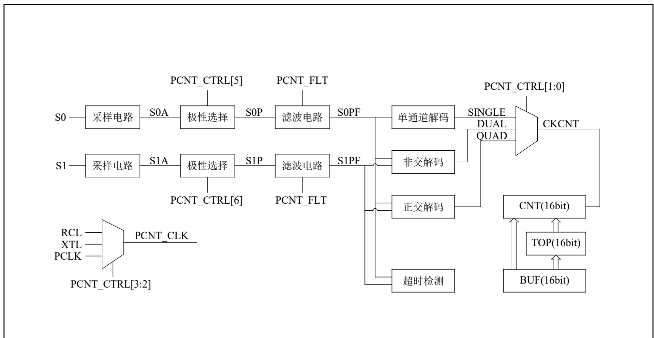
图 20-1 整体框图
