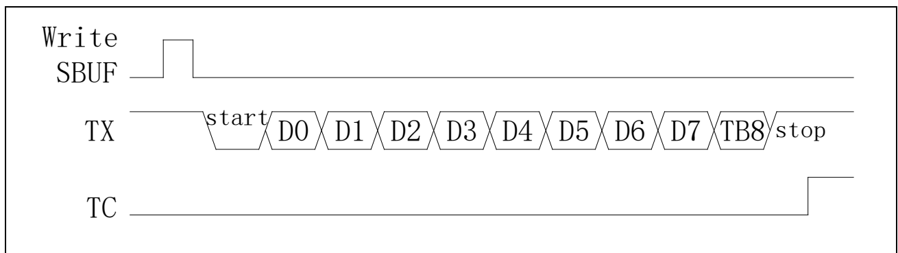
图 21-6 Mode2 发送数据
