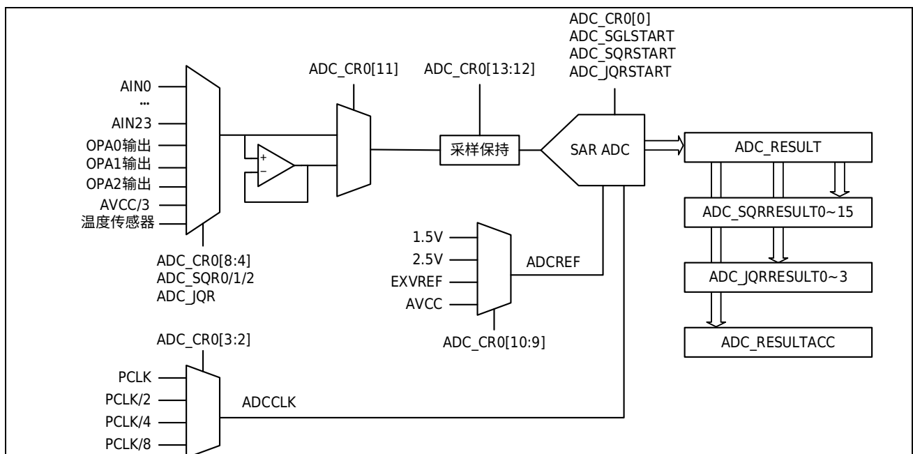
图 27-1 ADC 示意图
