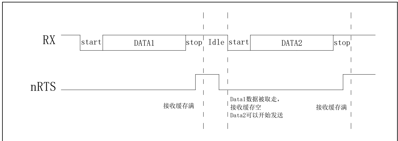
图 21-11 nRTS 硬件流控信号
