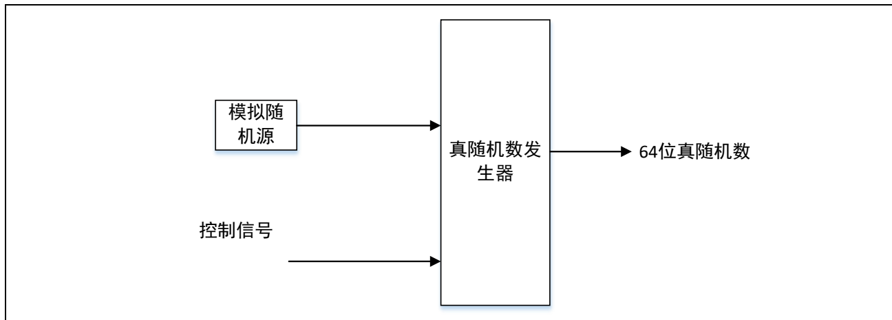
图 24-1 TRNG 数据流
