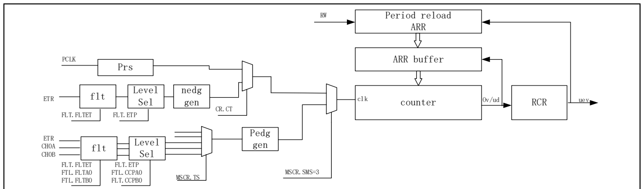
图 14-14 计数器框图
