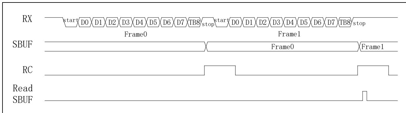
图 21-13 接收缓存
