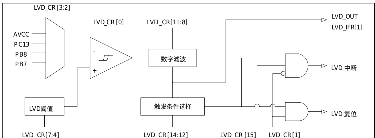
图 25-1 LVD 框图
