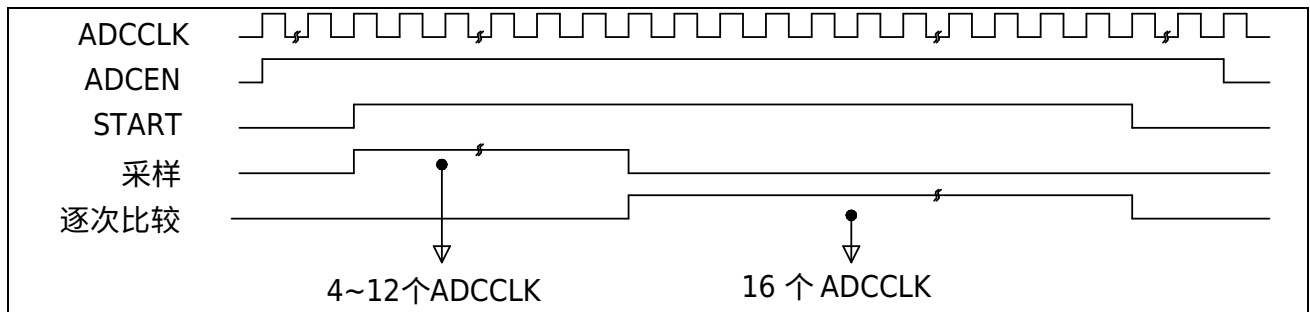
图 22-2 ADC 转换时序图
