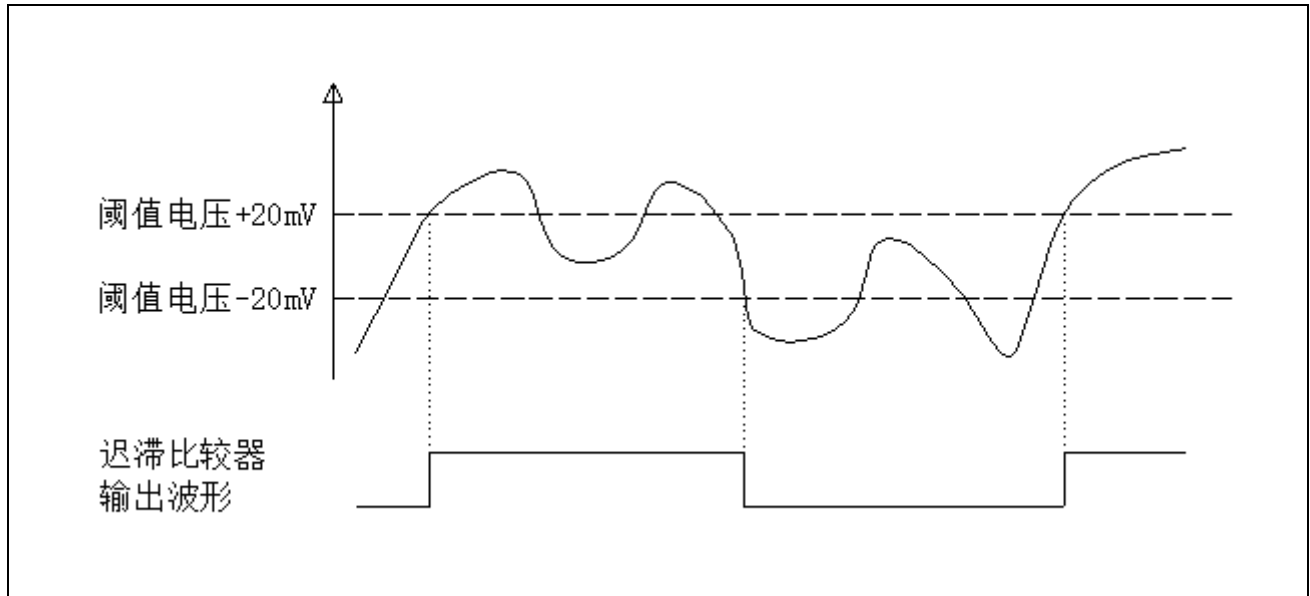
图 25-2 LVD 迟滞响应
