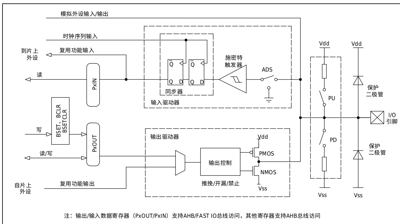
图 6-1 端口电路图
