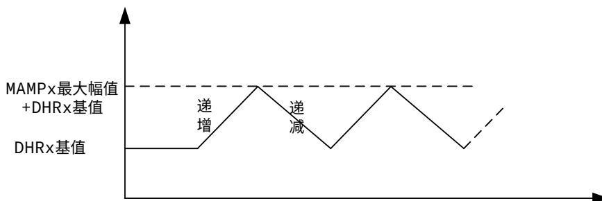
图 23-3 生成 DAC 三角波
