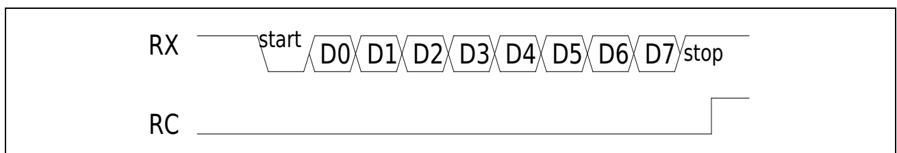
图 17-5 Mode1 接收数据
