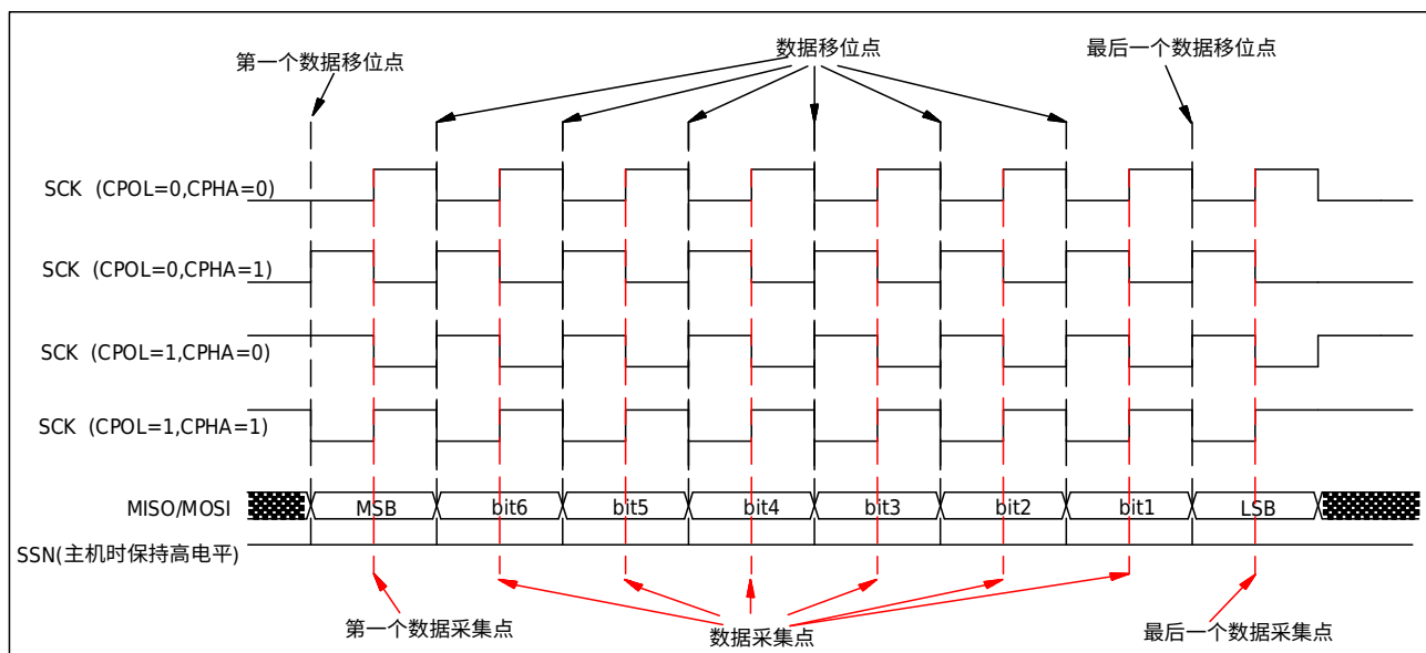
图 8-3 主机模式帧格式
