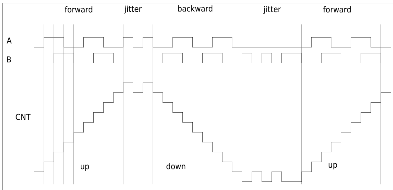
图 13-54 编码计数
