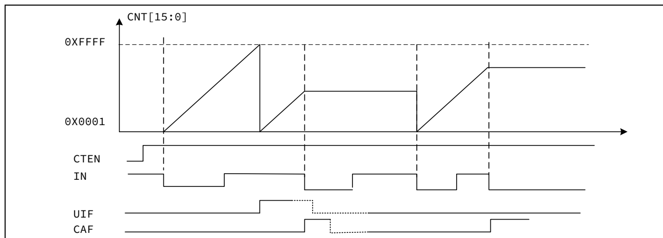
图 13-11 下降沿到下降沿周期测量
