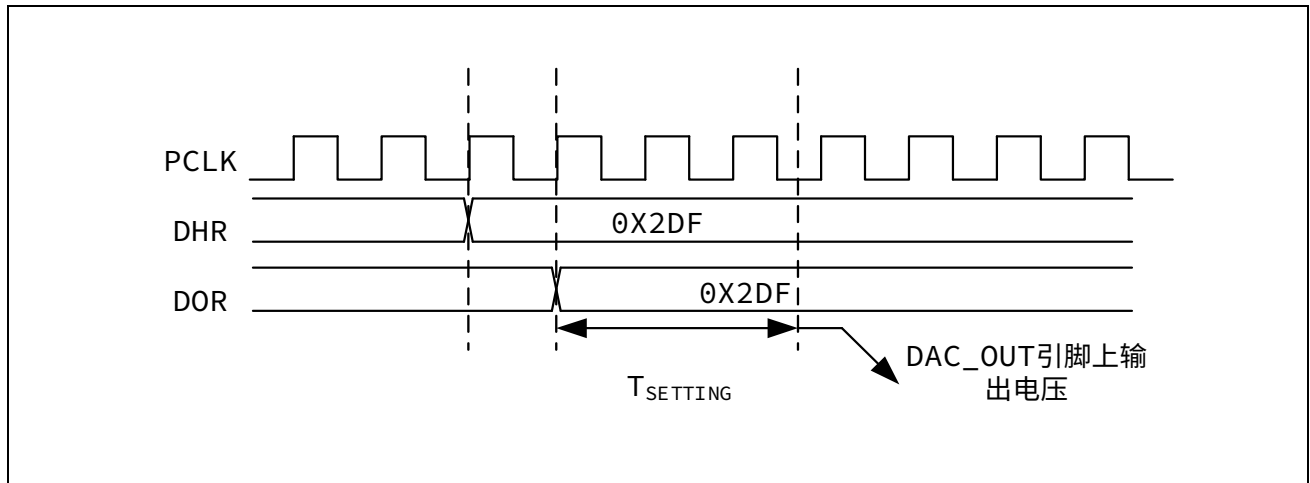
图 23-1 触发不使能时 DAC 转换时序图
