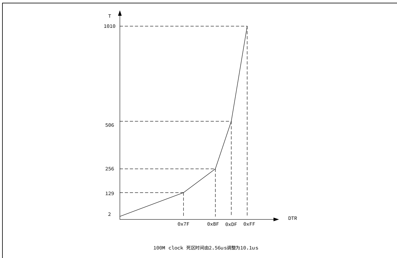
图 13-42 死区时间
