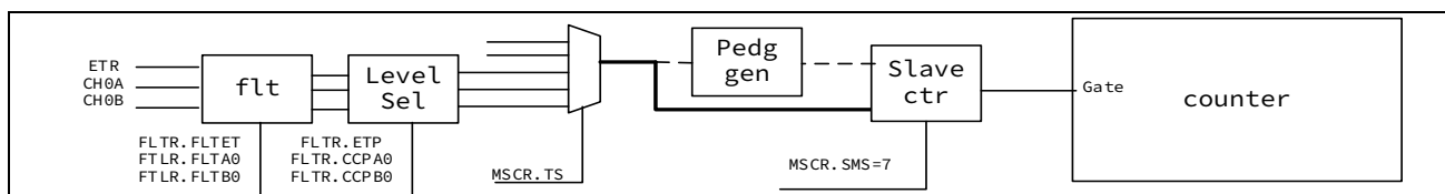
图 13-52 门控功能
