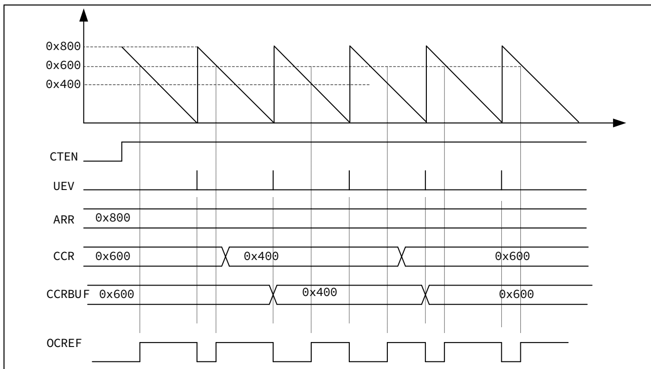
图 13-30 锯齿波模式下计数比较缓存使能
