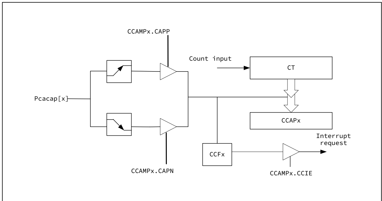
图 14-3 PCA 捕获功能框图
