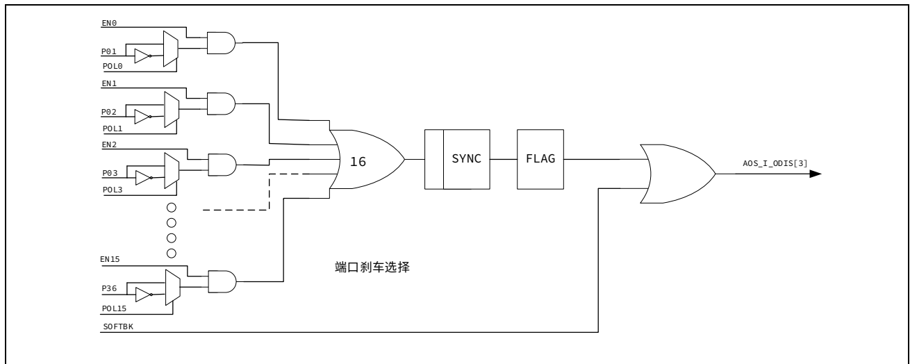
图 15-27 端口刹车与软件刹车示意图
