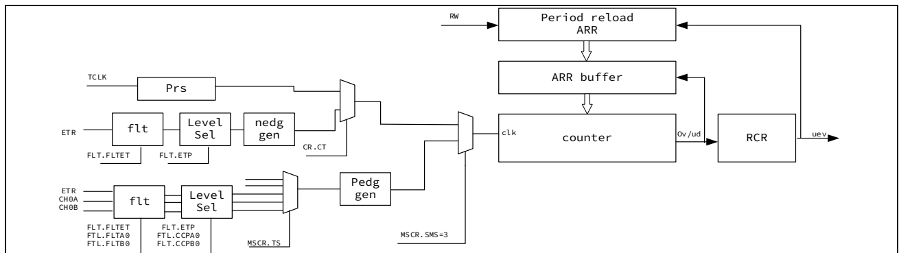
图 13-14 计数器框图
