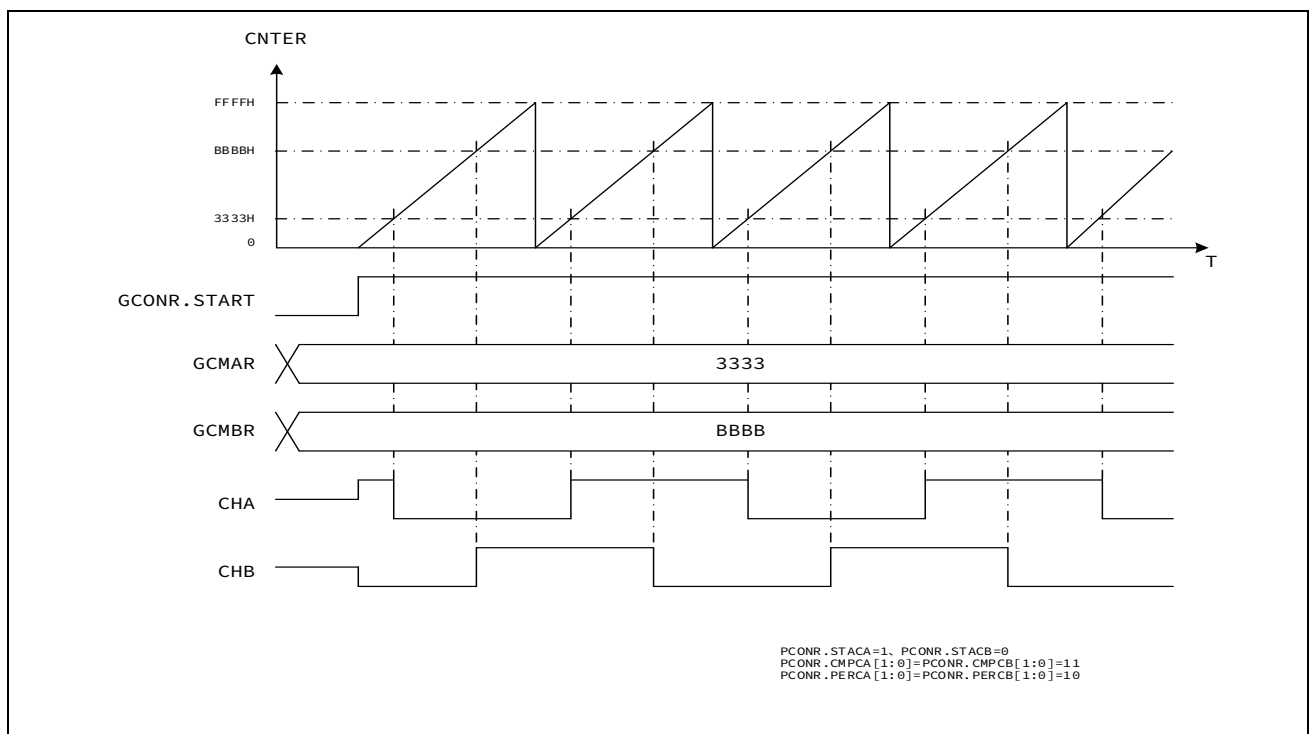
图 15-4 比较输出动作
