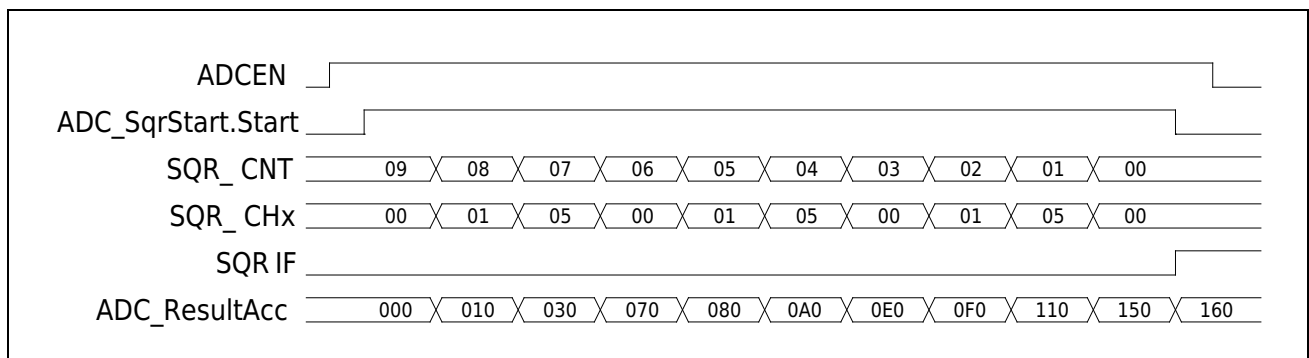
图 22-6 ADC 连续转换累加过程示例
