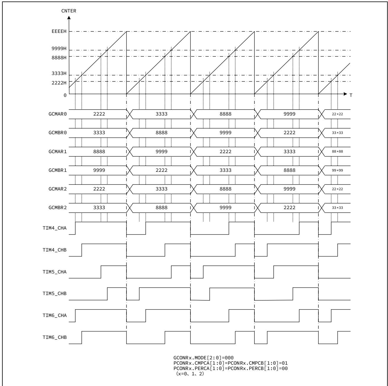
图 15-14 6 相 PWM 波
