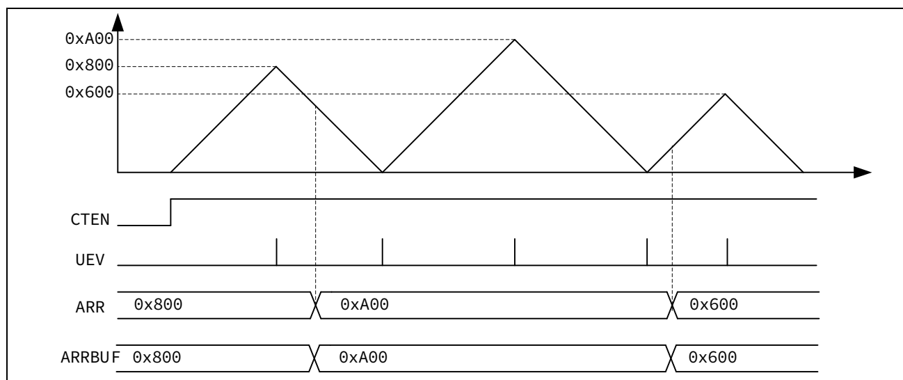
图 13-25 三角波模式下缓存无效
