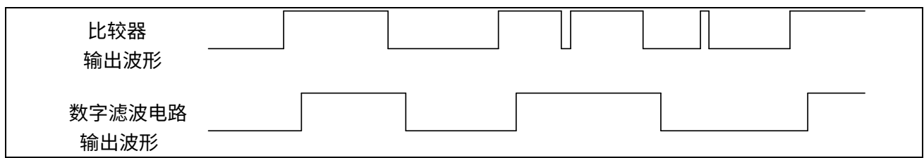
图 24-2 VC 滤波响应时间
