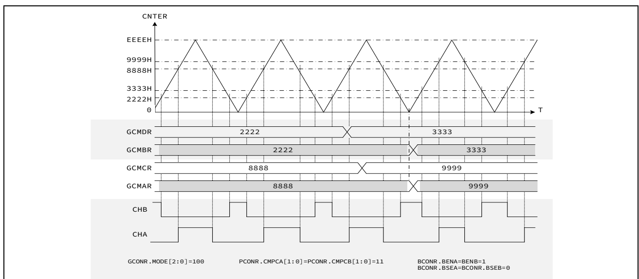
图 15-12 三角波 A 模式时软件设定 GCMBR 互补 PWM 波输出
