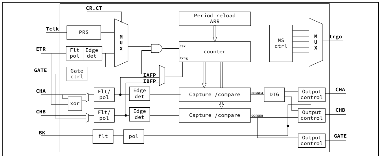
图 13-1 TIM0/1/2 框图
