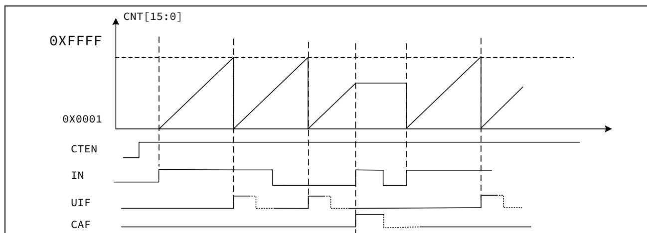
图 13-12 上升沿到上升沿周期测量
