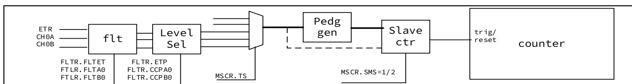
图 13-53 触发和复位功能
