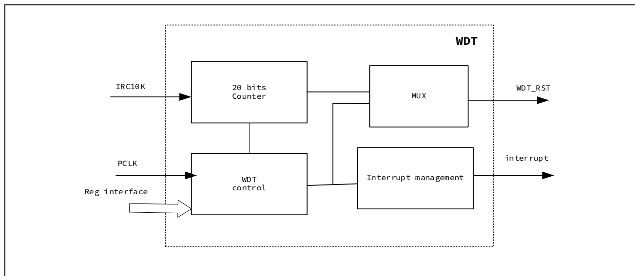
图 16-1 WDT 整体框图
