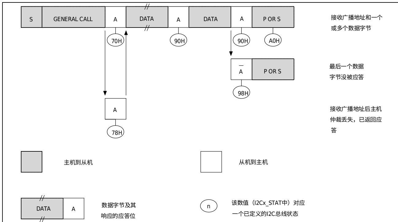
图 7-15 I2C 广播呼叫状态图
