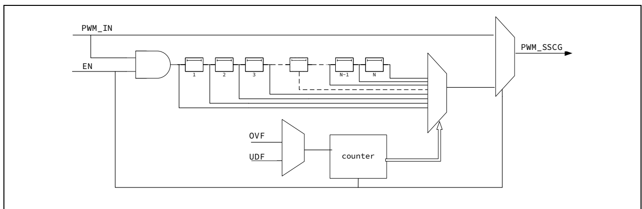
图 15-10 PWM 展频输出示意图
