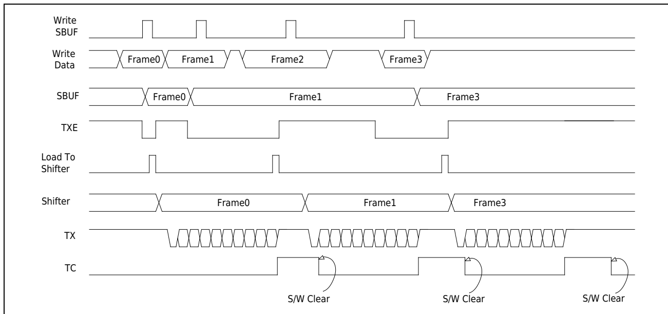
图 17-14 发送缓存
