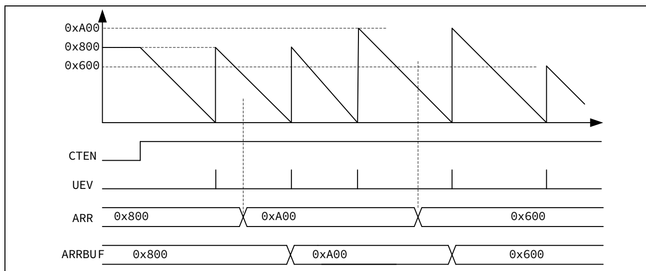
图 13-28 锯齿波模式下计数缓存使能
