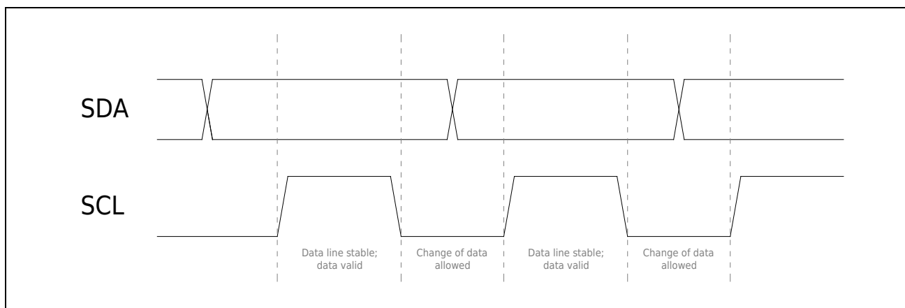
图 7-3 I2C 总线上位传输
