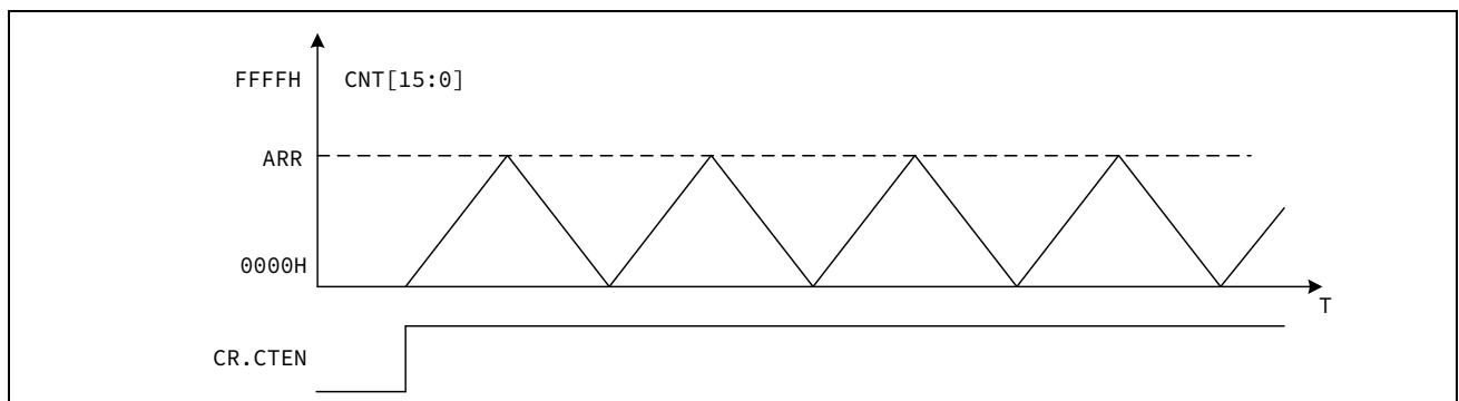
图 13-22 中心对齐计数器波形
