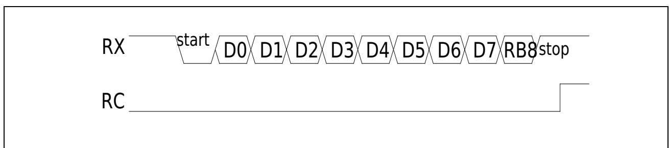
图 17-7 Mode2 接收数据
