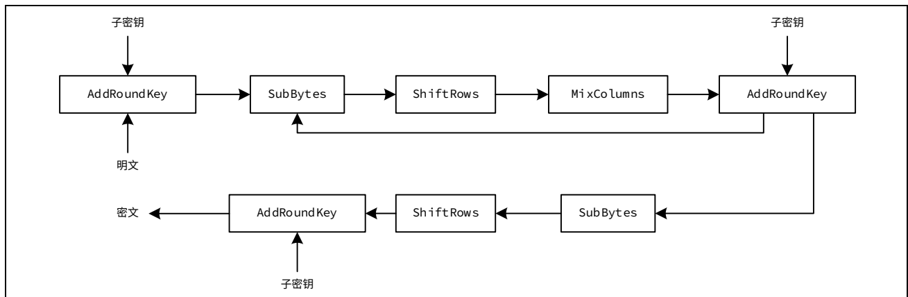
图 20-2 AES 的加密流程图
