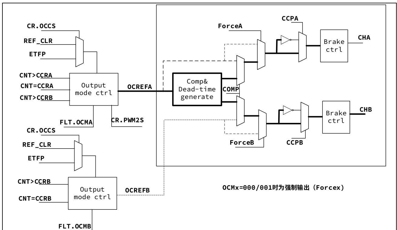
图 13-39 互补 PWM 输出框图
