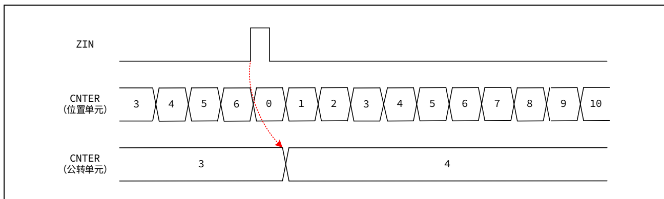
图 15-21 公转模式时 Z 相计数动作
