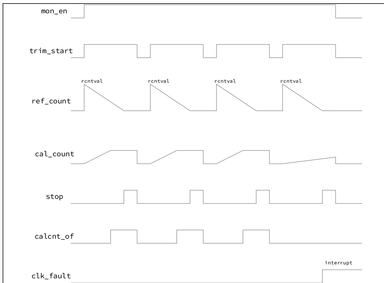
图 9-5 时钟监控波形示意图
