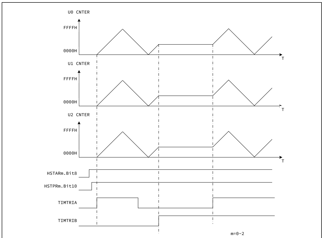
图 15-8 硬件同步动作
