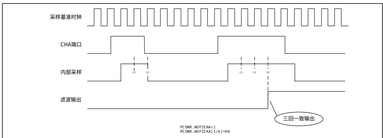
图 15-6 捕获输入端口的滤波功能
