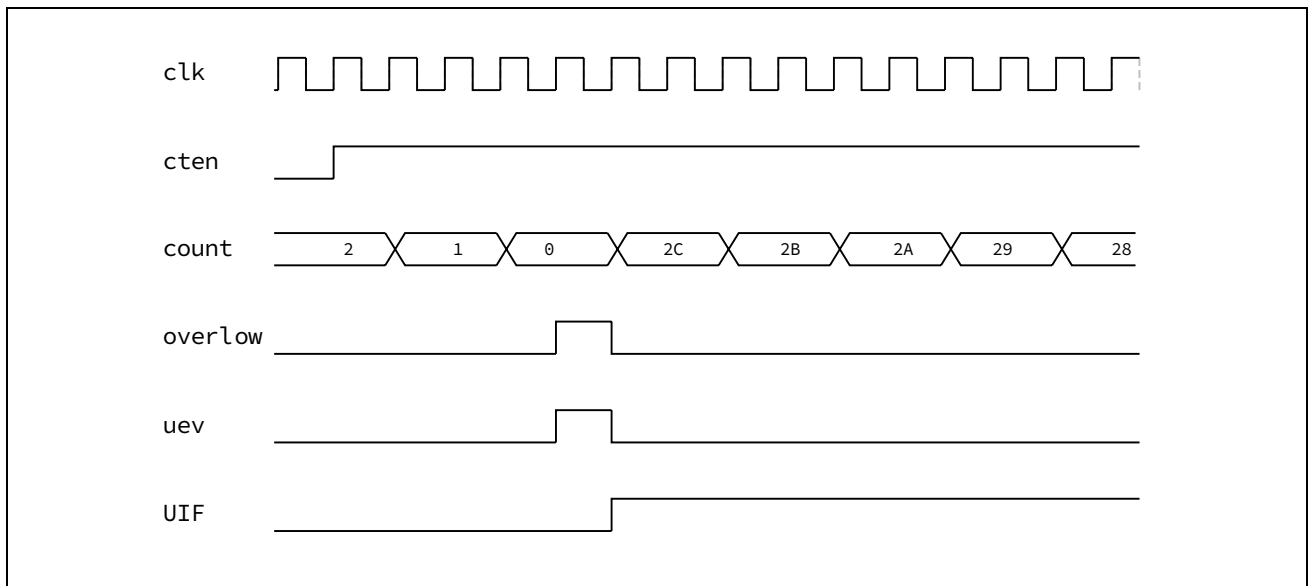
图 13-18 带预分频的下计数
