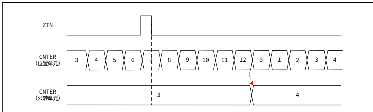
图 15-22 公转模式时位置计数器输出计数动作
