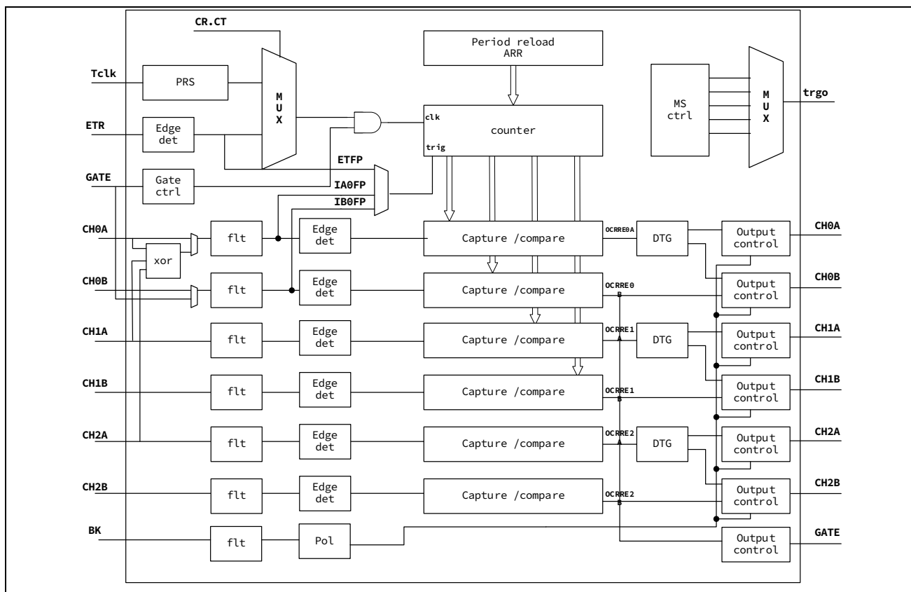
图 13-2 TIM3 框图
