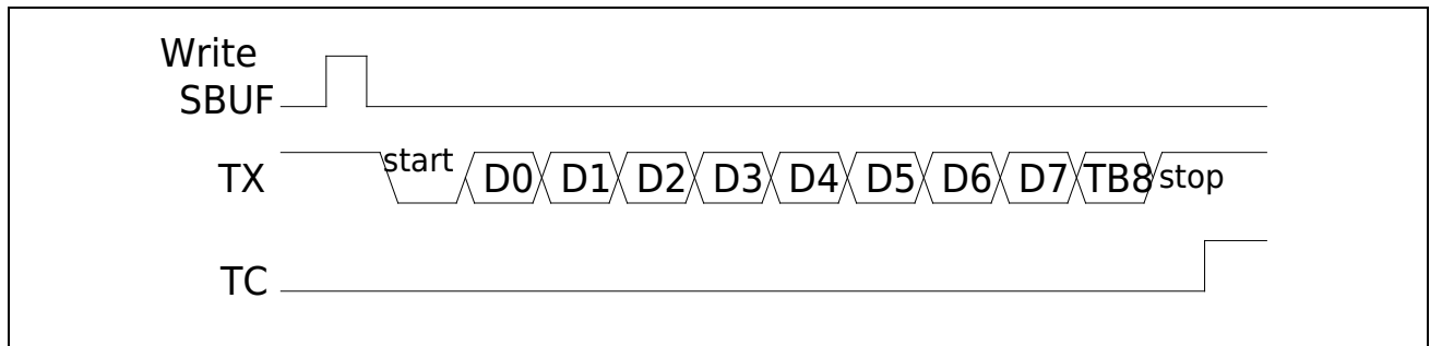
图 17-8 Mode3 发送数据
