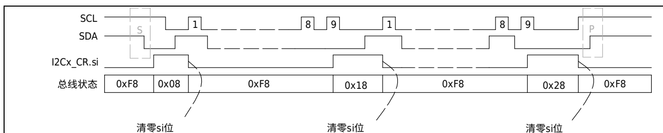
图 7-7 主发送模式数据同步图
