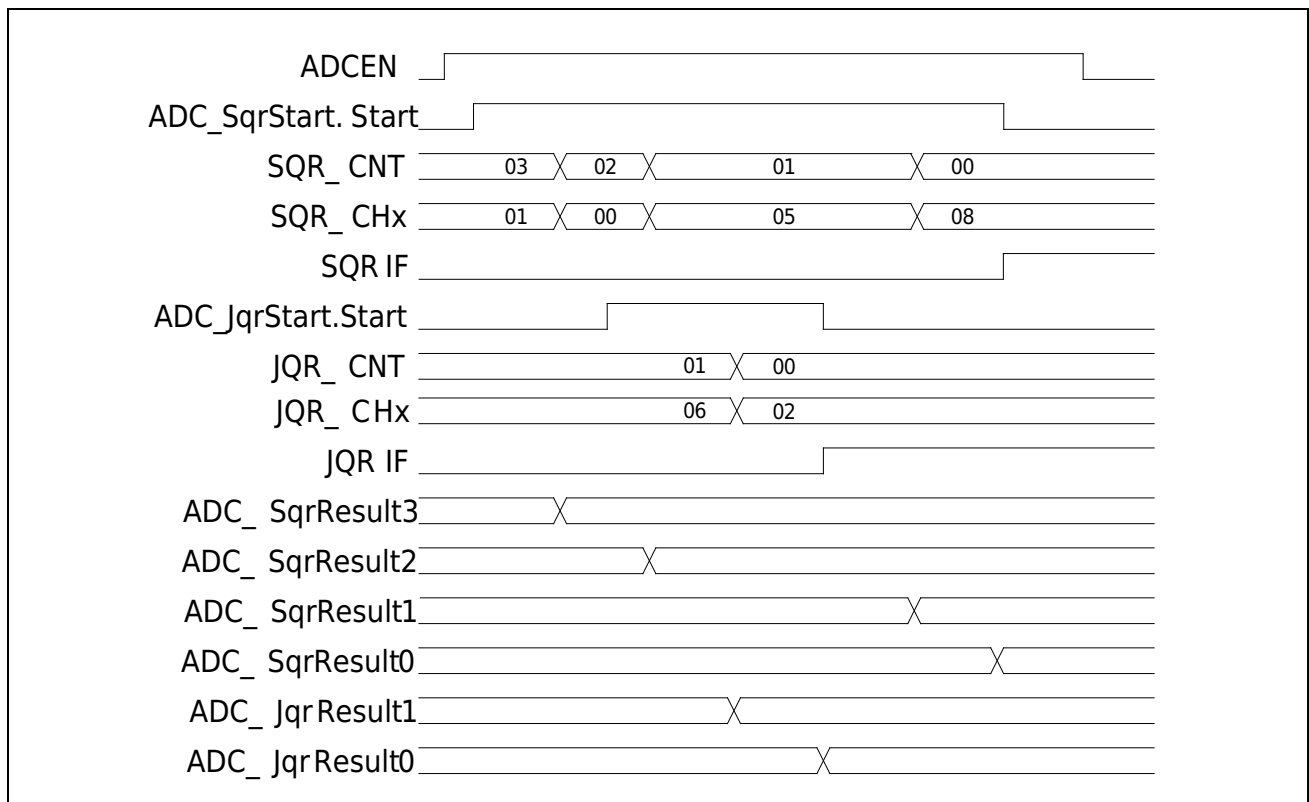
图 22-5 ADC 顺序扫描过程中进行插队扫描示例
