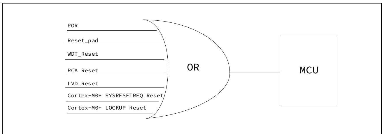
图 4-1 复位来源示意图
