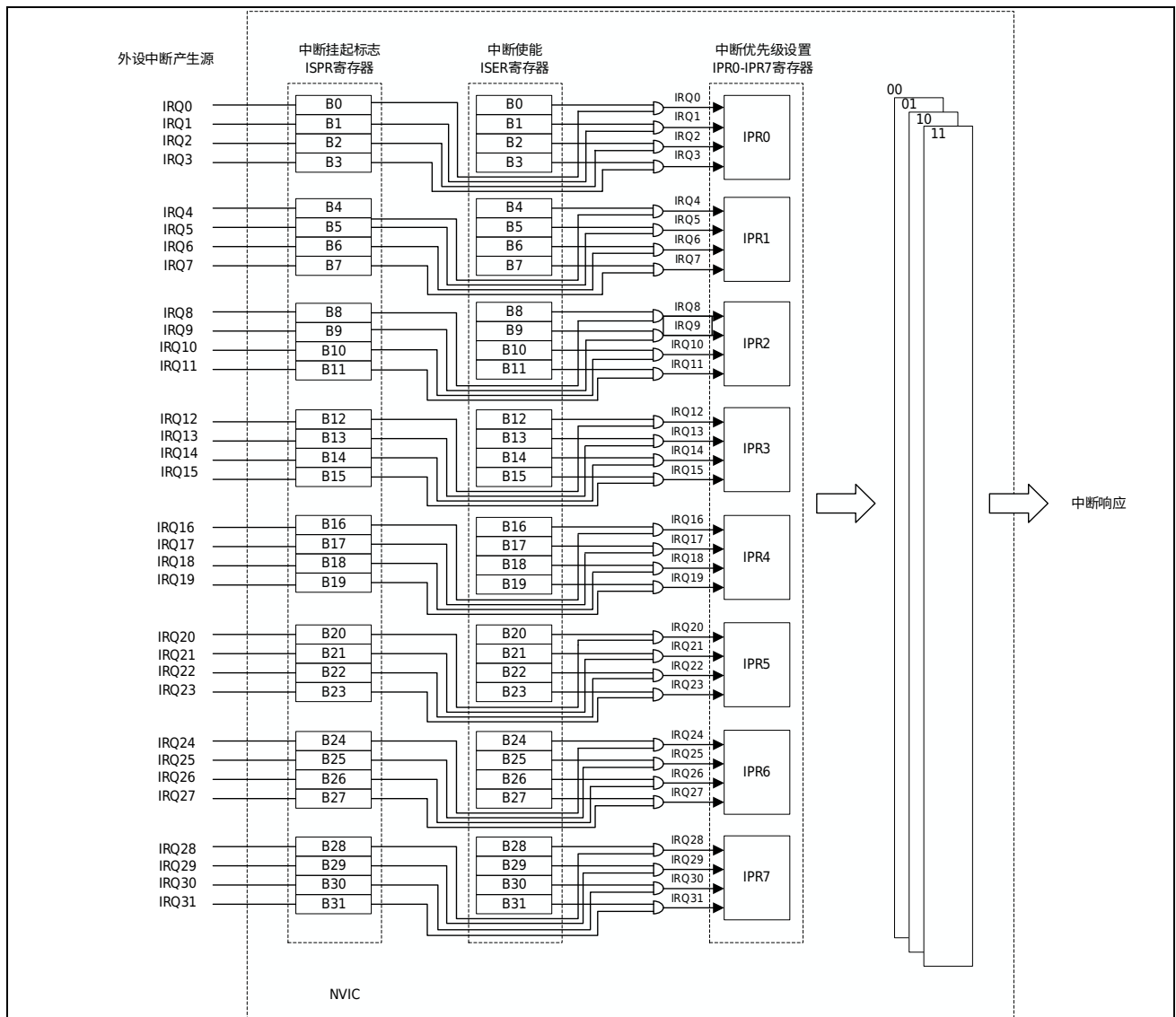
图 5-7 中断结构图
