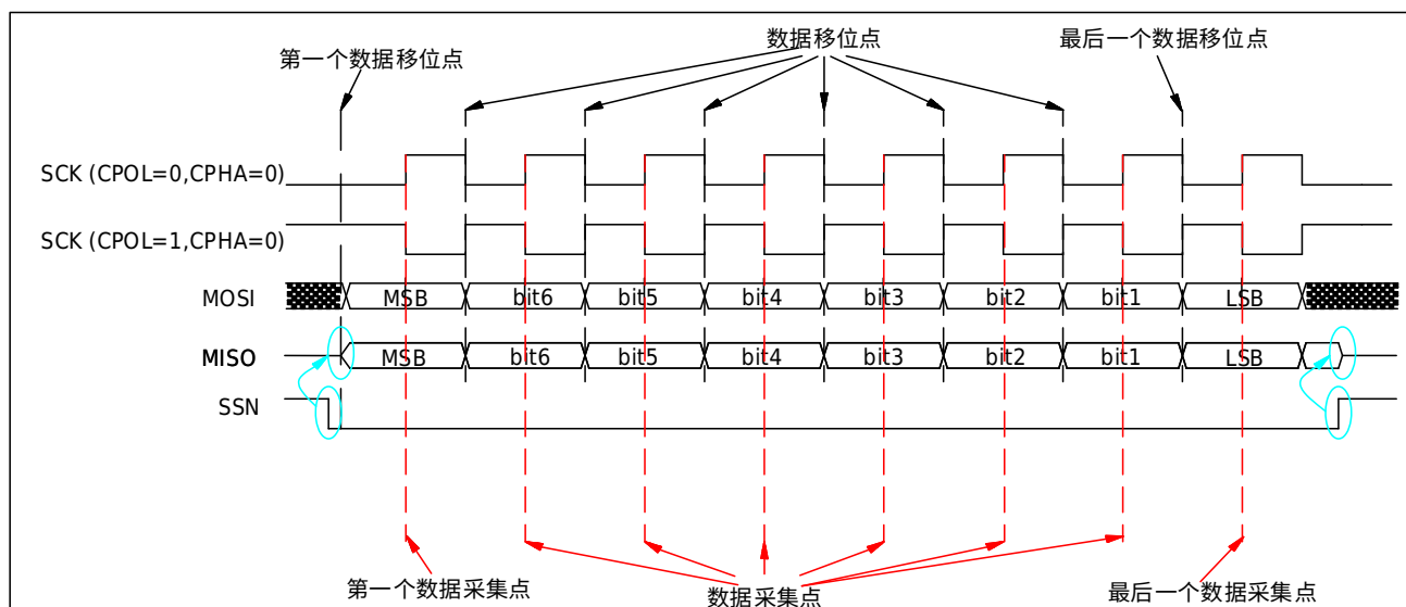
图 8-4 从机 CPHA 为 0 时数据帧格式
