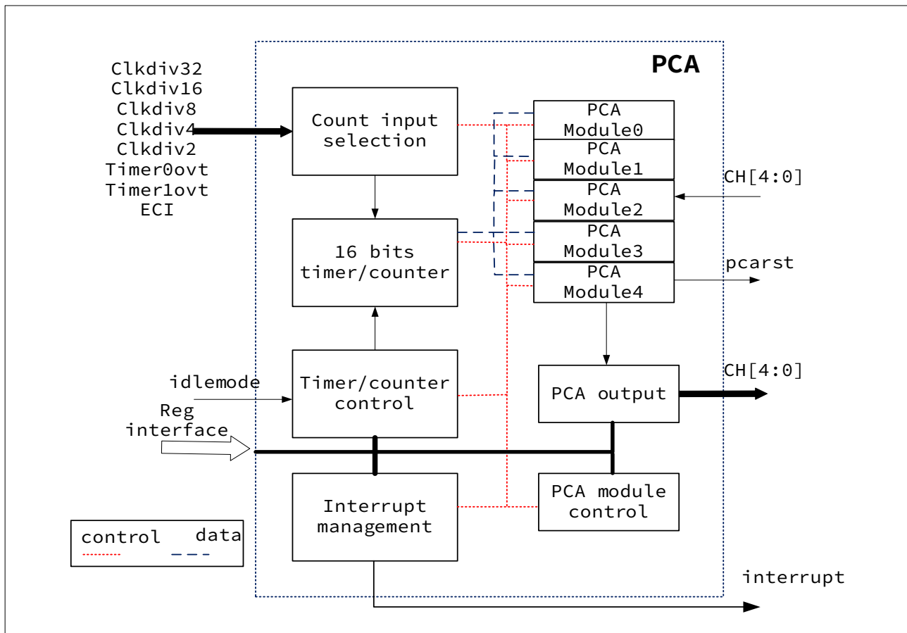
图 14-1 PCA 整体框图
