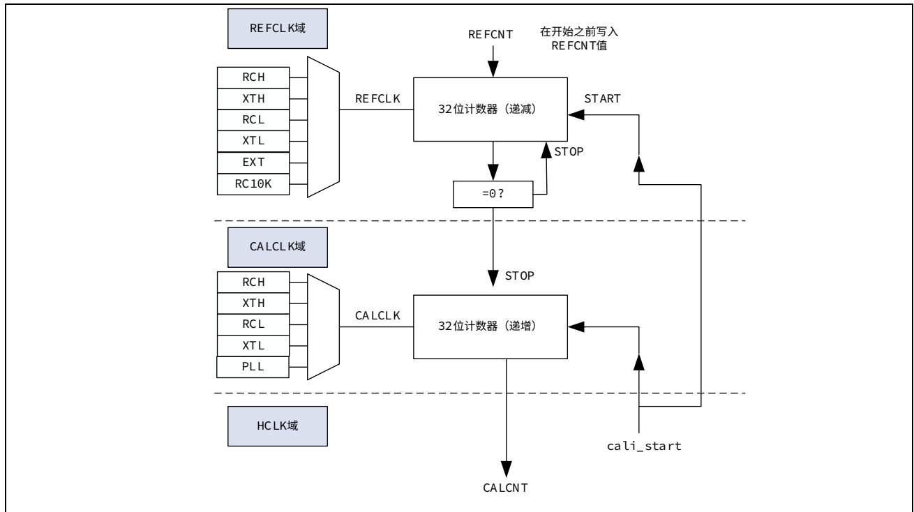
图 3-4 时钟校准原理图
