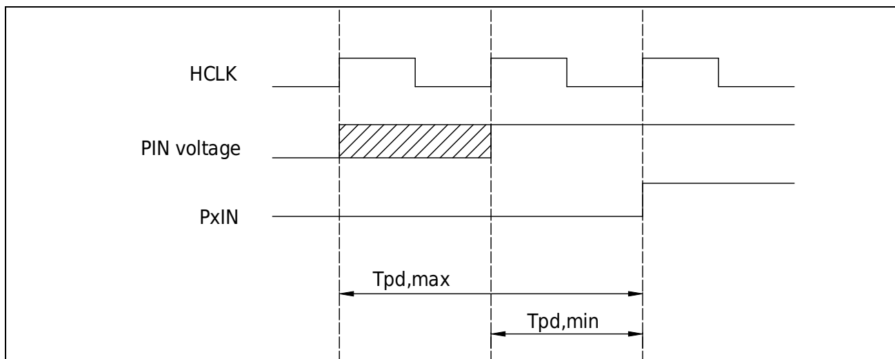
图 6-3 读取端口引脚数据同步图
