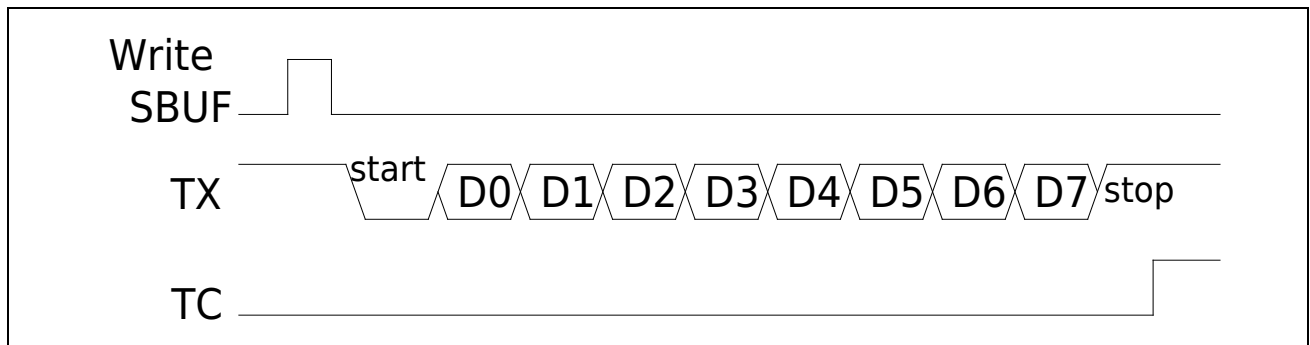
图 17-4 Mode1 发送数据
