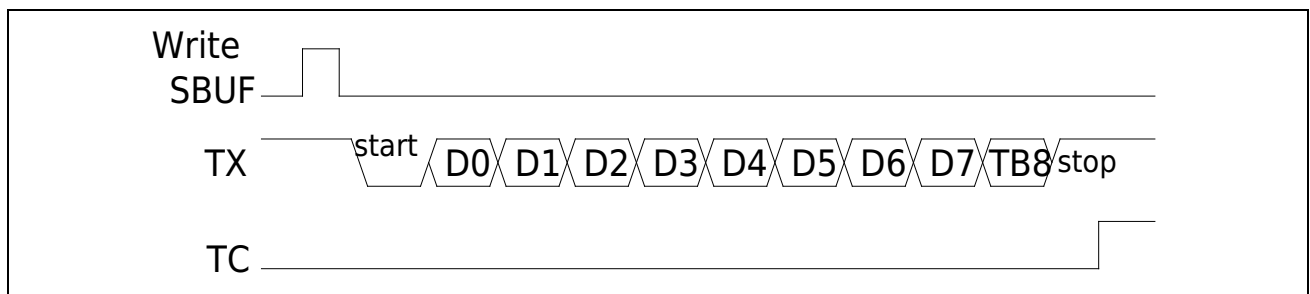
图 17-6 Mode2 发送数据
