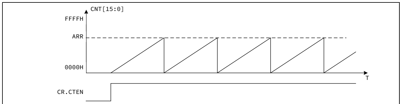
图 13-21 边沿对齐计时器波形 ( DIR =0)
