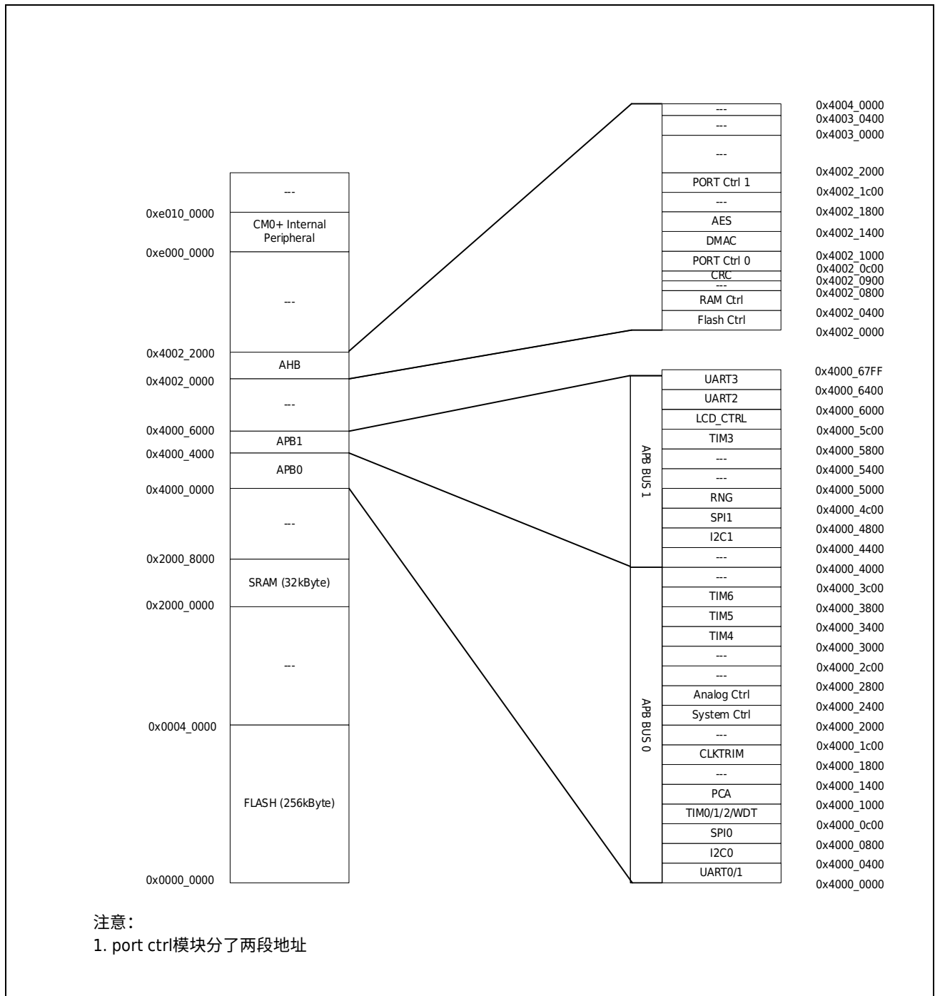
图 1-2 地址区域划分示意图
