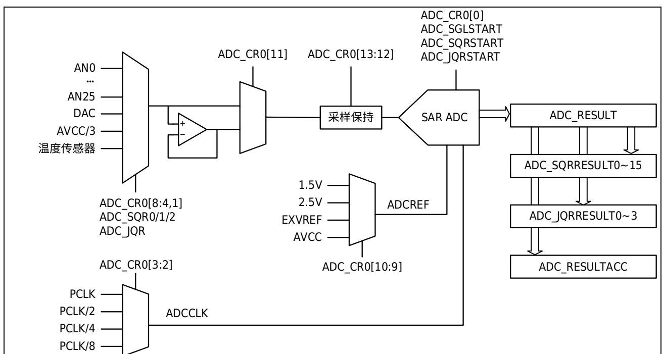
图 22-1 ADC 示意图
