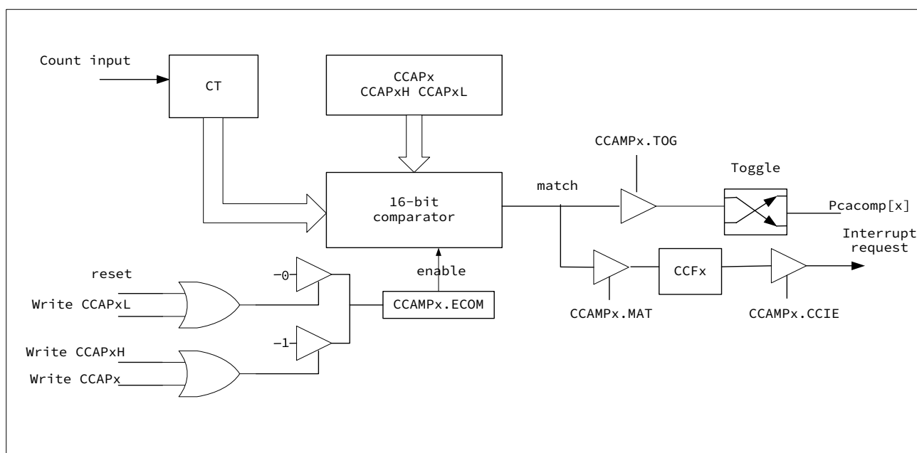
图 14-4 PCA 比较功能框图
