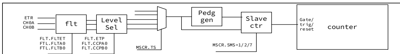
图 13-51 从模式示意图
