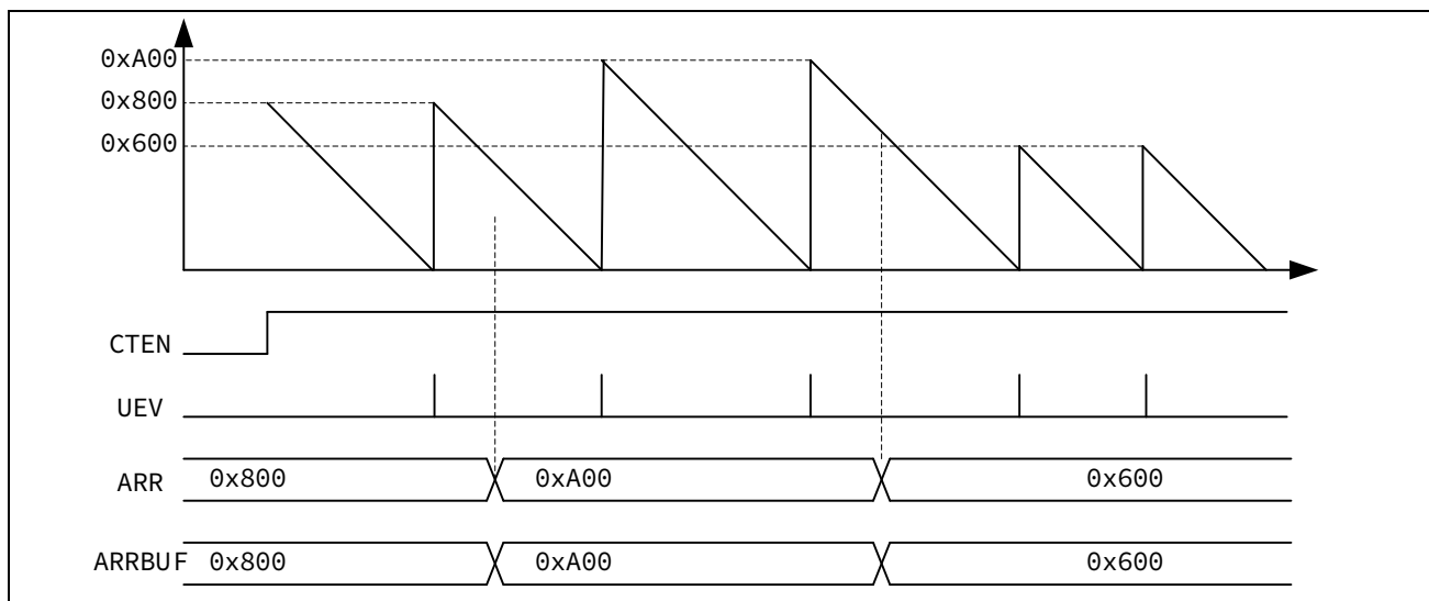
图 13-29 锯齿波模式下计数缓存无效
