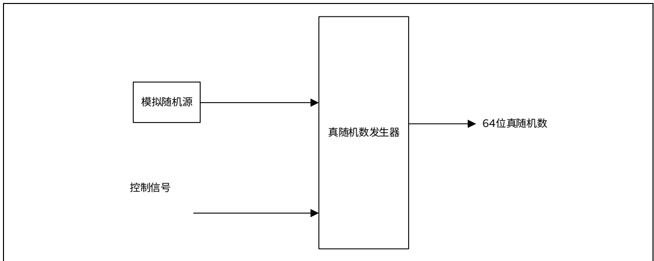
图 19-1 TRNG 数据流
