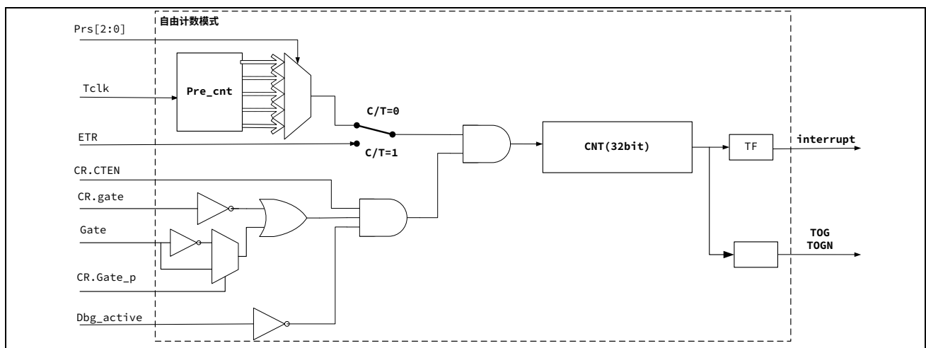
图 13-3 自由计数框图
