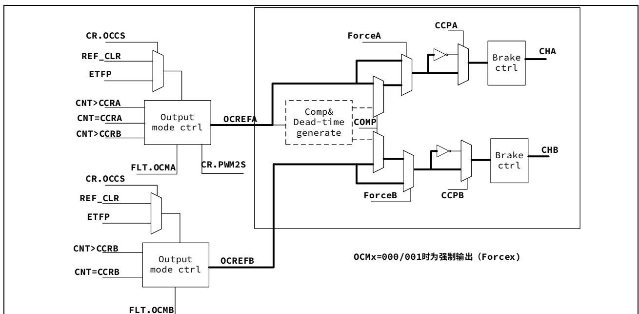
图 13-36 独立 PWM 输出框图
