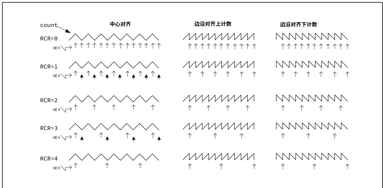
图 13-23 重复计数器产生更新时序
