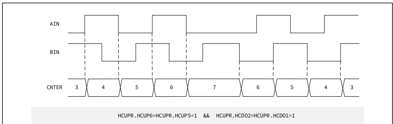
图 15-18 位置模式时相位差计数动作设定 (2 倍)
