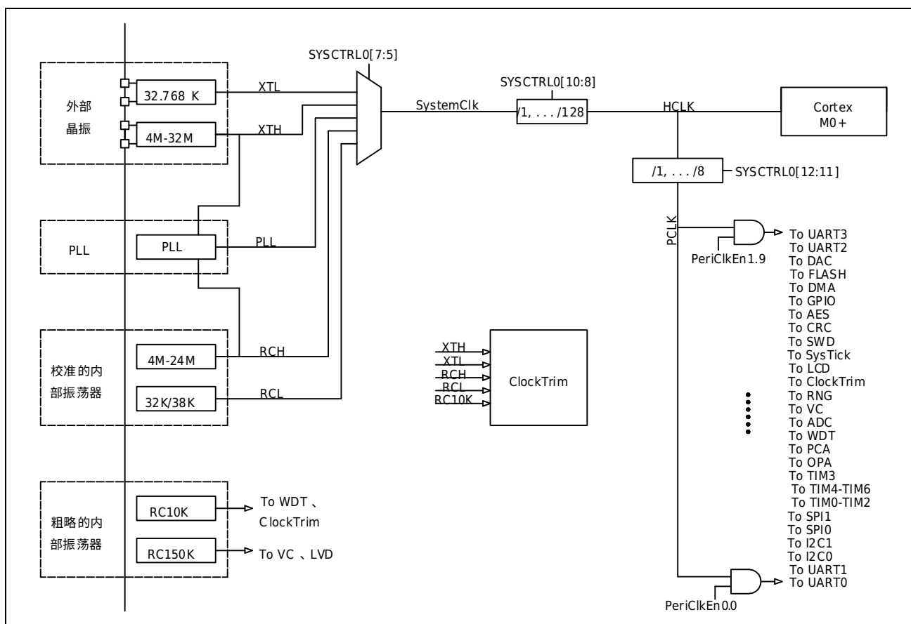
图 3-1 时钟控制模块框图
