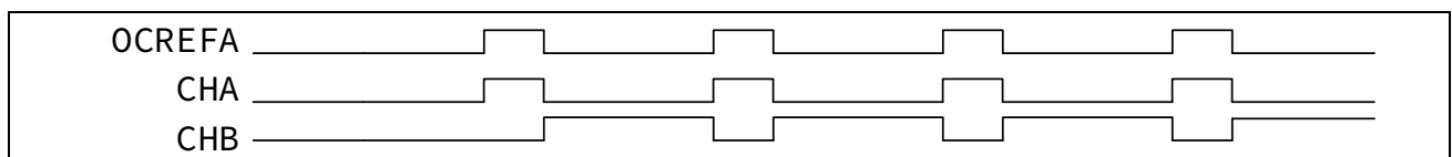
图 13-40 互补 PWM 输出波形图
