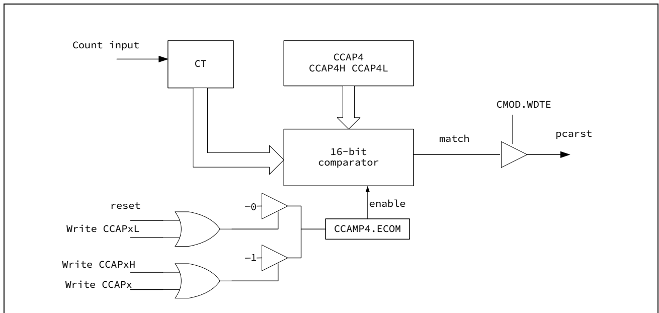
图 14-6 PCA WDT 功能框图
