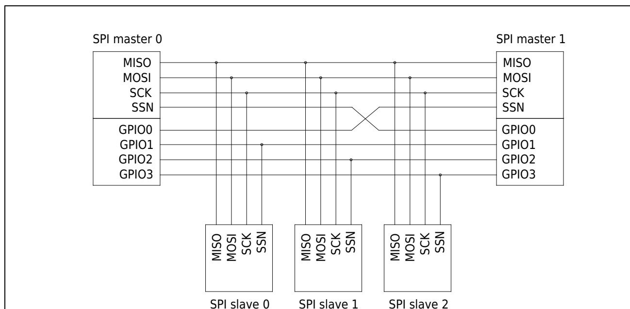
图 8-6 SPI 多主机/多从机系统的示意图
