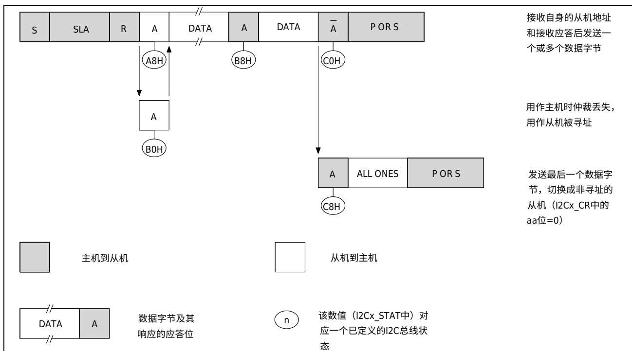
图 7-14 I2C 从机发送状态图
