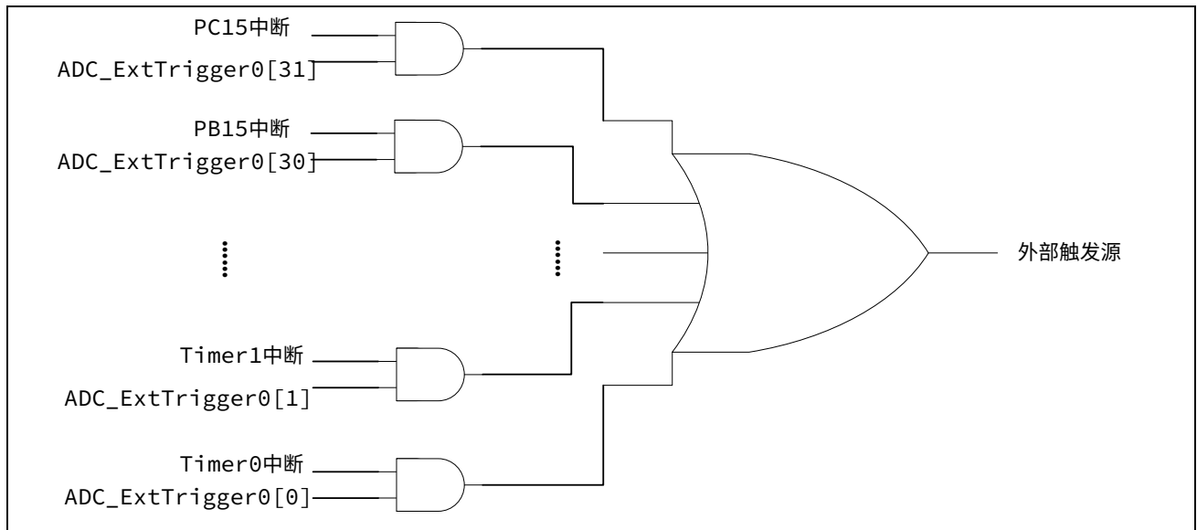
图 22-7 ADC 单次转换或顺序扫描转换外部触发源示意图
