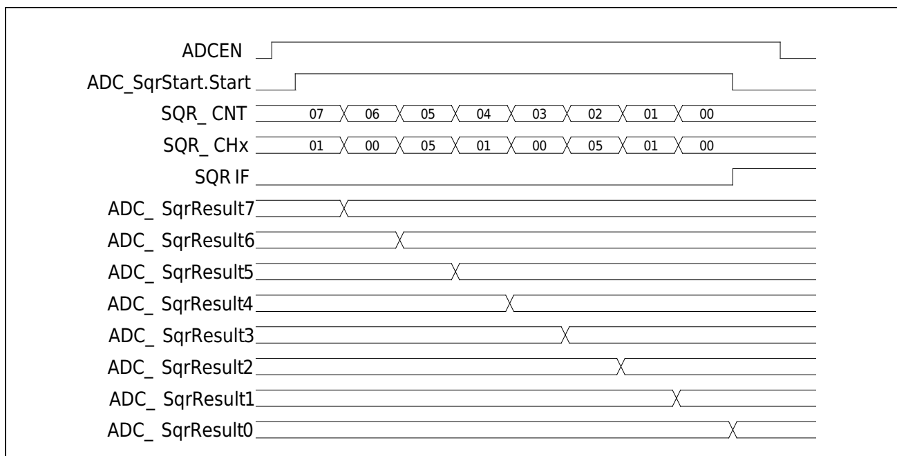
图 22-3 ADC 顺序扫描转换过程示例
