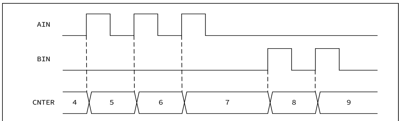
图 15-16 位置模式时基本计数动作
