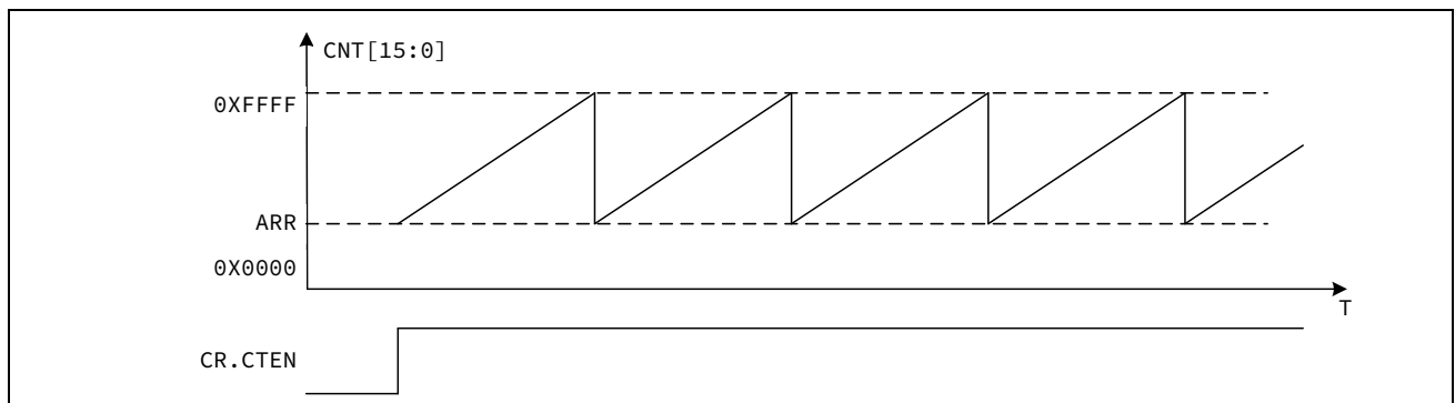
图 13-5 16 位重载计数波形
