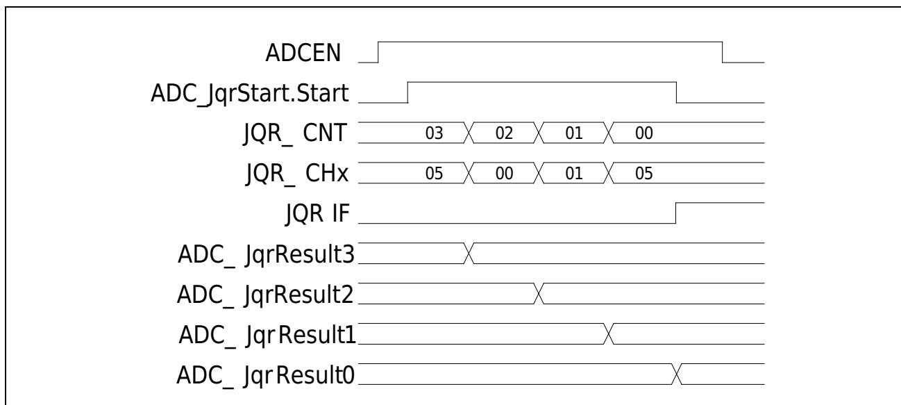
图 22-4 ADC 插队扫描转换过程示例
