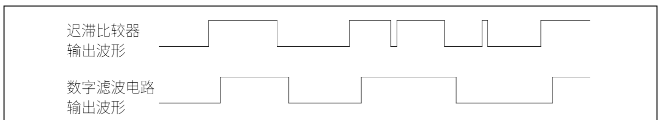
图 25-3 LVD 滤波输出
