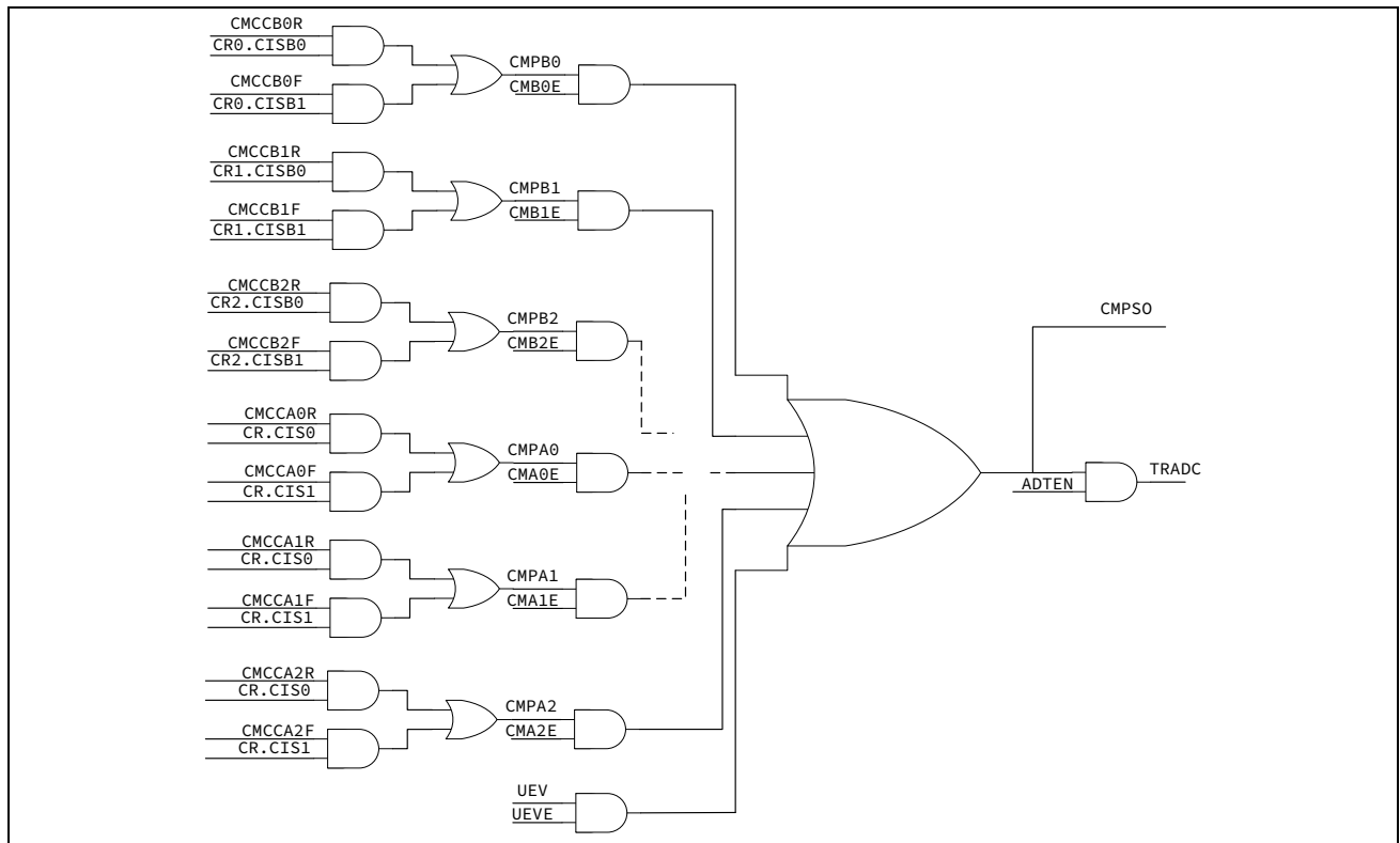
图 13-55 ADC 触发
