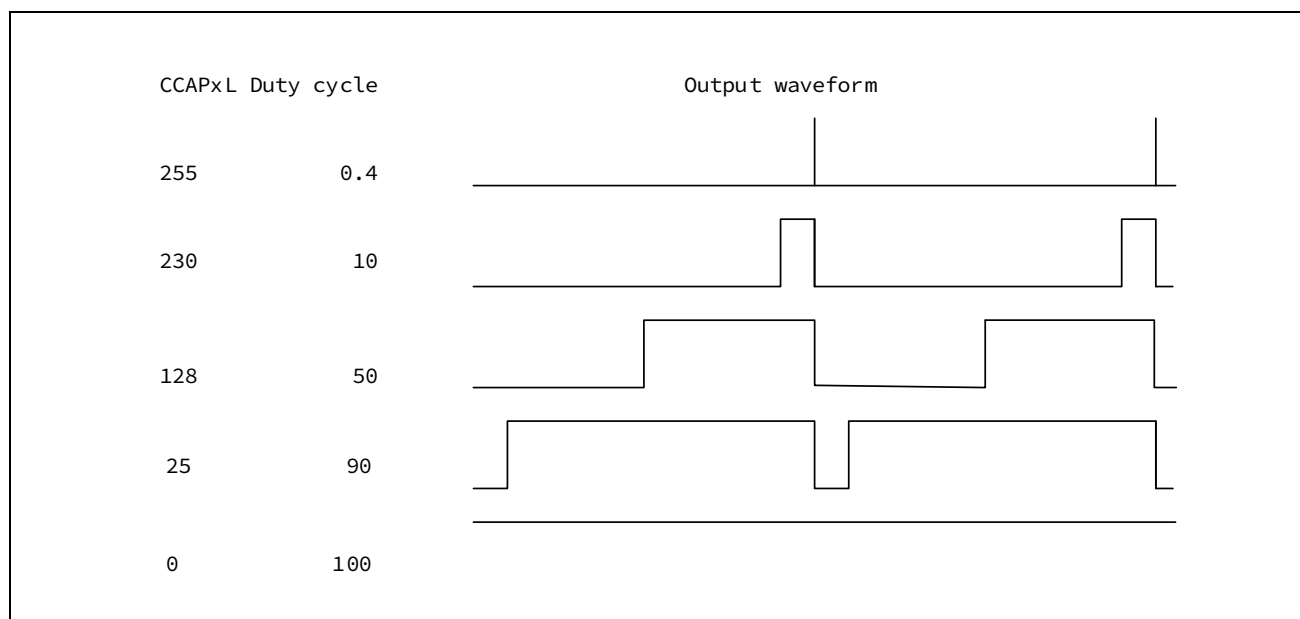
图 14-8 PCA PWM 输出波形
