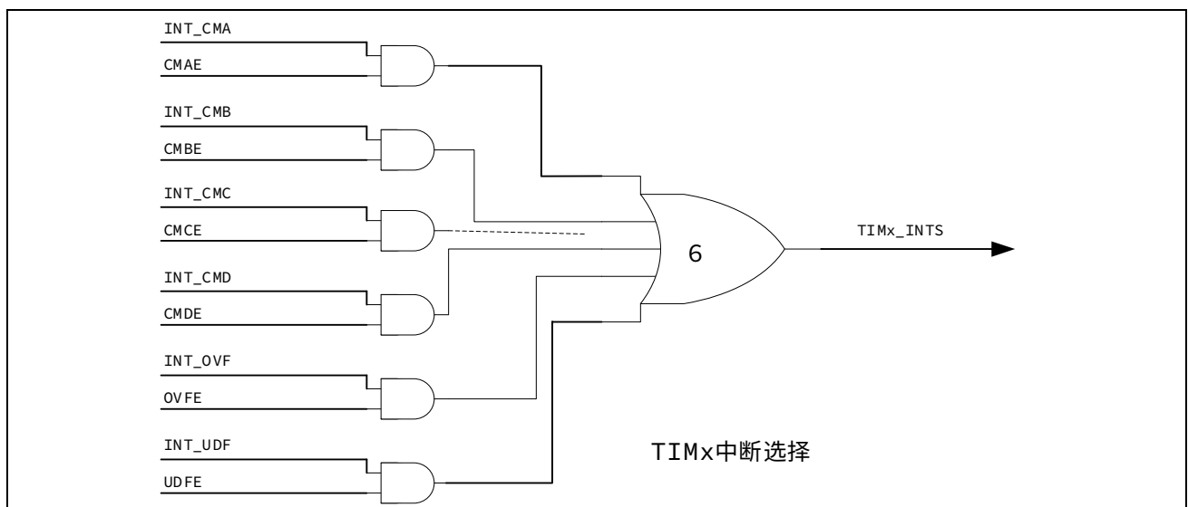
图 15-30 Timer4/5/6 中断选择
