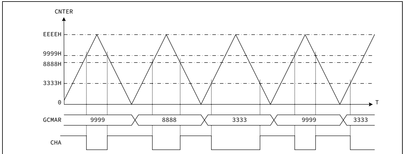
图 15-11 CHA 输出 PWM 波
