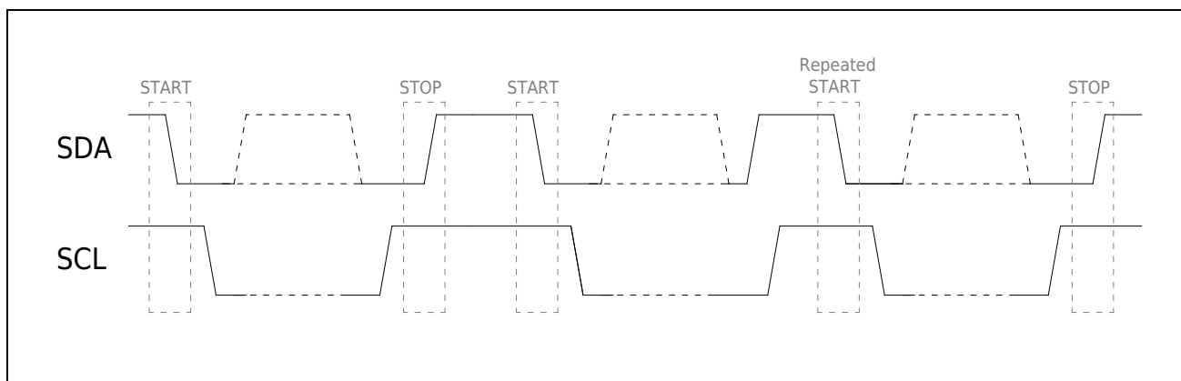
图 7-2 START 和 STOP 条件
