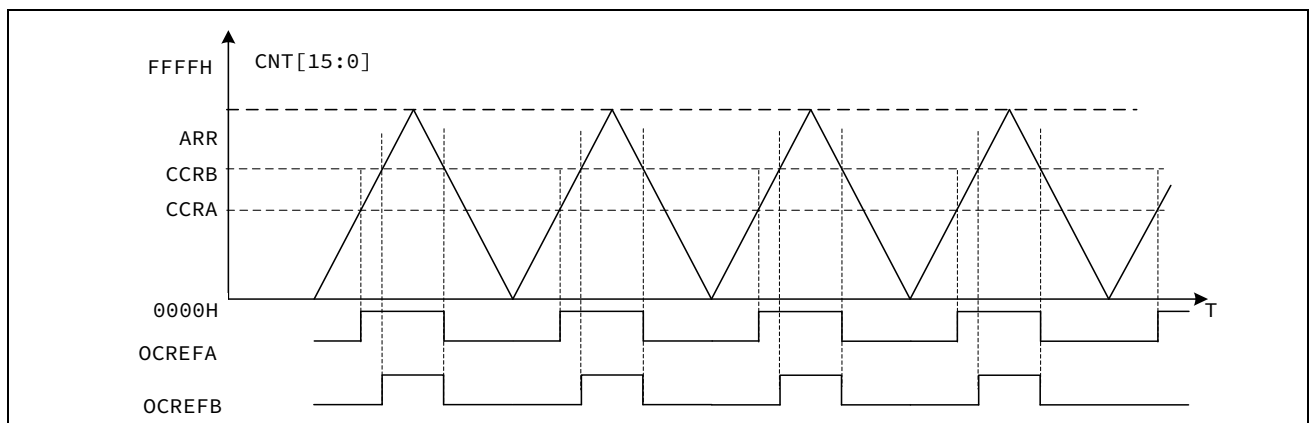
图 13-35 三角波计数双点比较 OCREF 输出 (OCMx=111)
