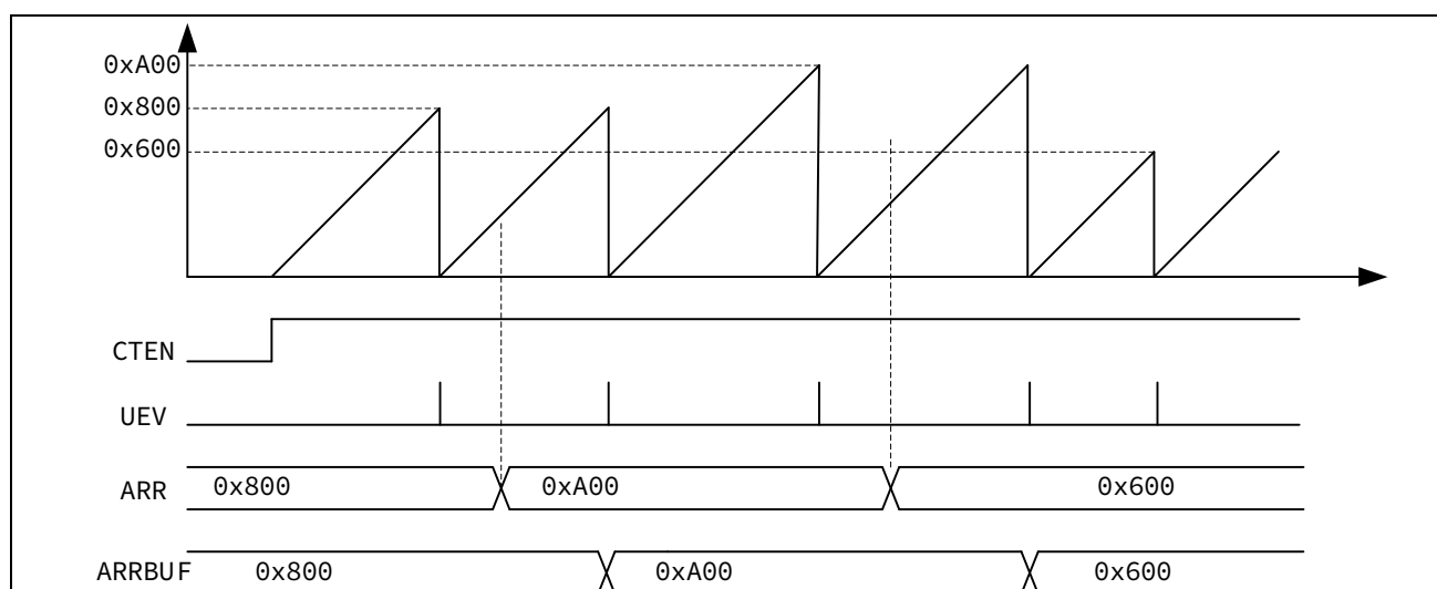
图 13-26 锯齿波模式下计数缓存使能
