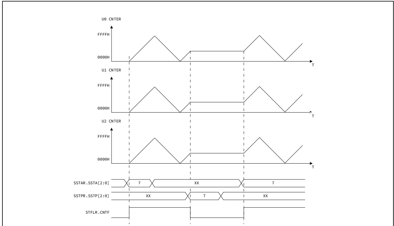
图 15-7 软件同步动作
