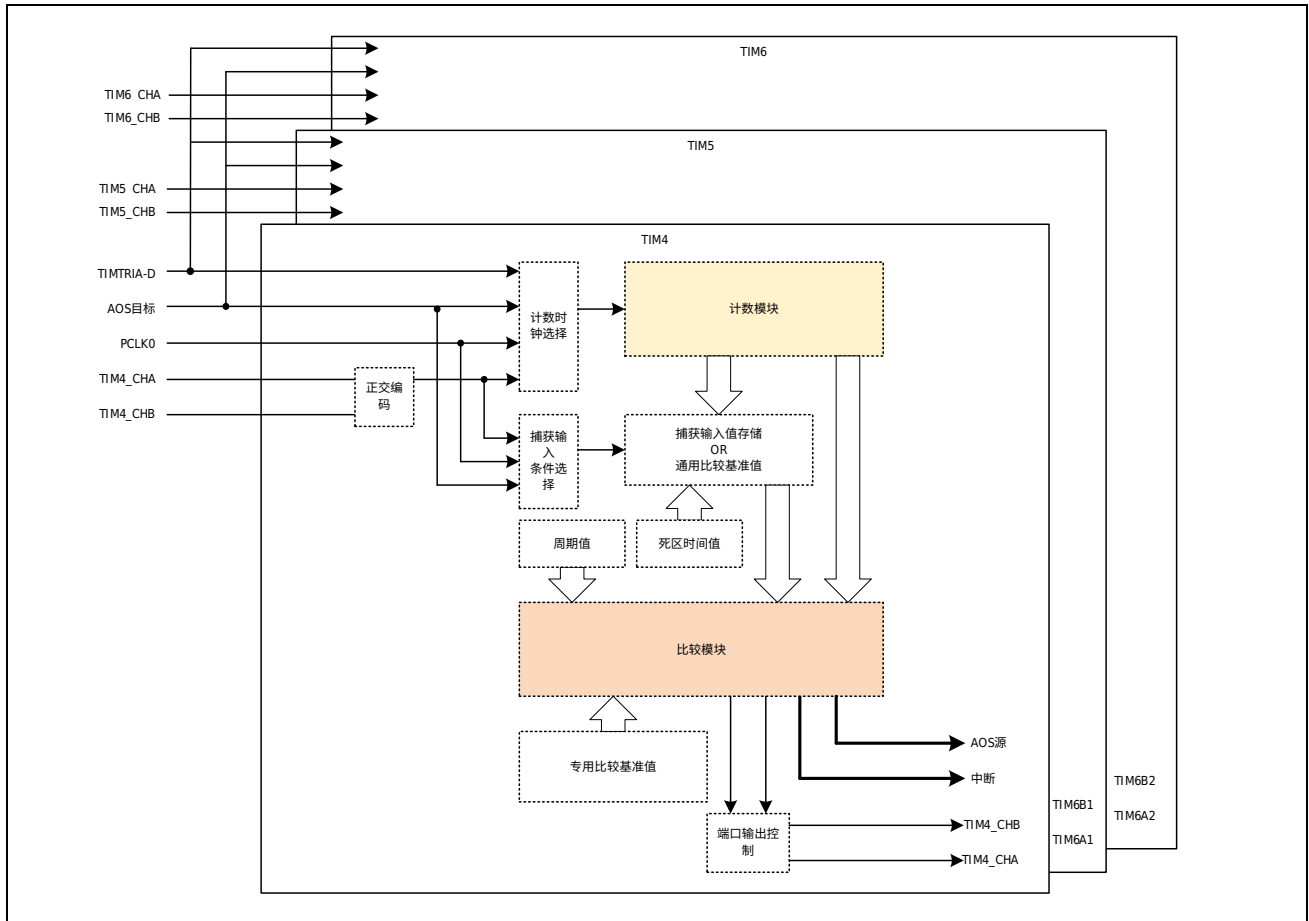
图 15-1 Advanced Timer 框图
