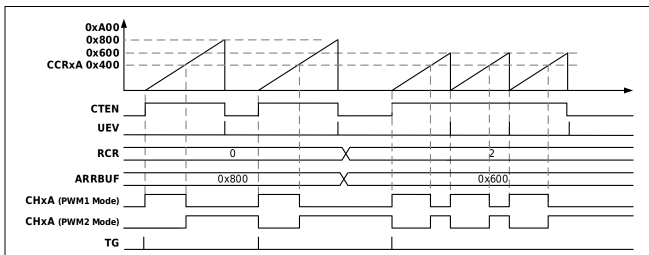
图 13-44 锯齿波上计数单脉冲模式
