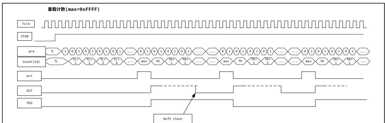
图 13-8 重载计数时序图（预分频设置为 2）
