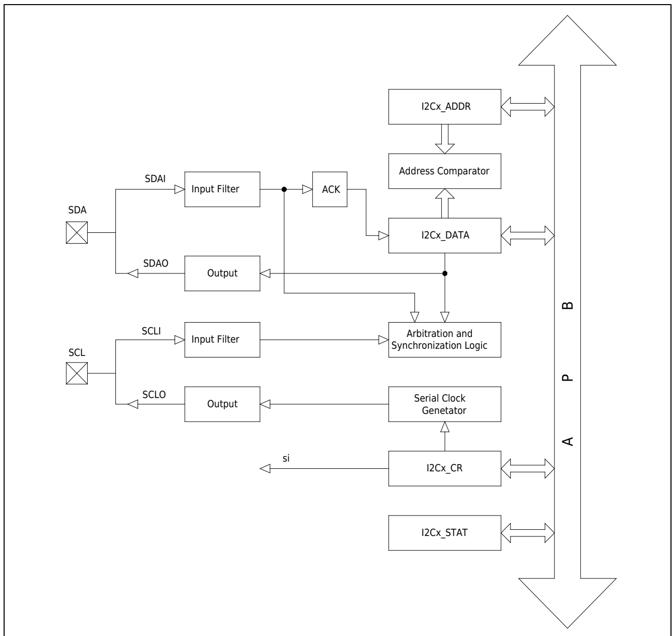
图 7-6 I2C 功能模块图
