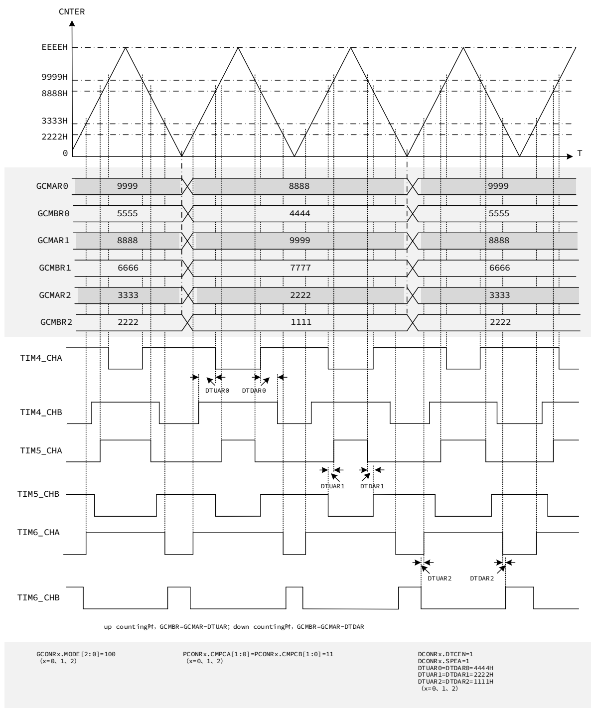
图 15-15 三角波 A 模式时带死区时间三相互补 PWM 波输出
