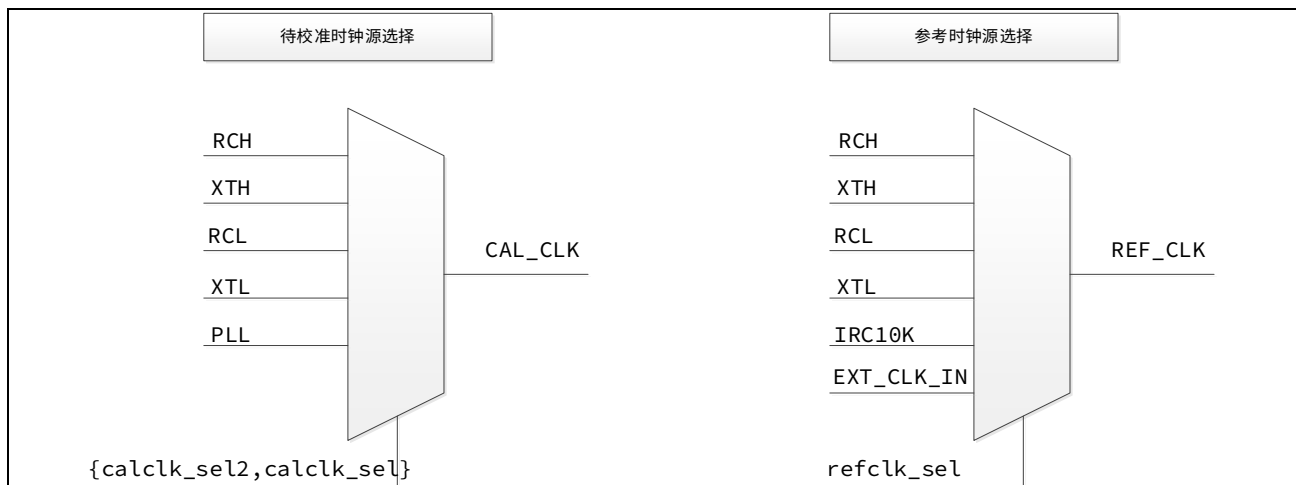
图 9-1 时钟源选择示意图
