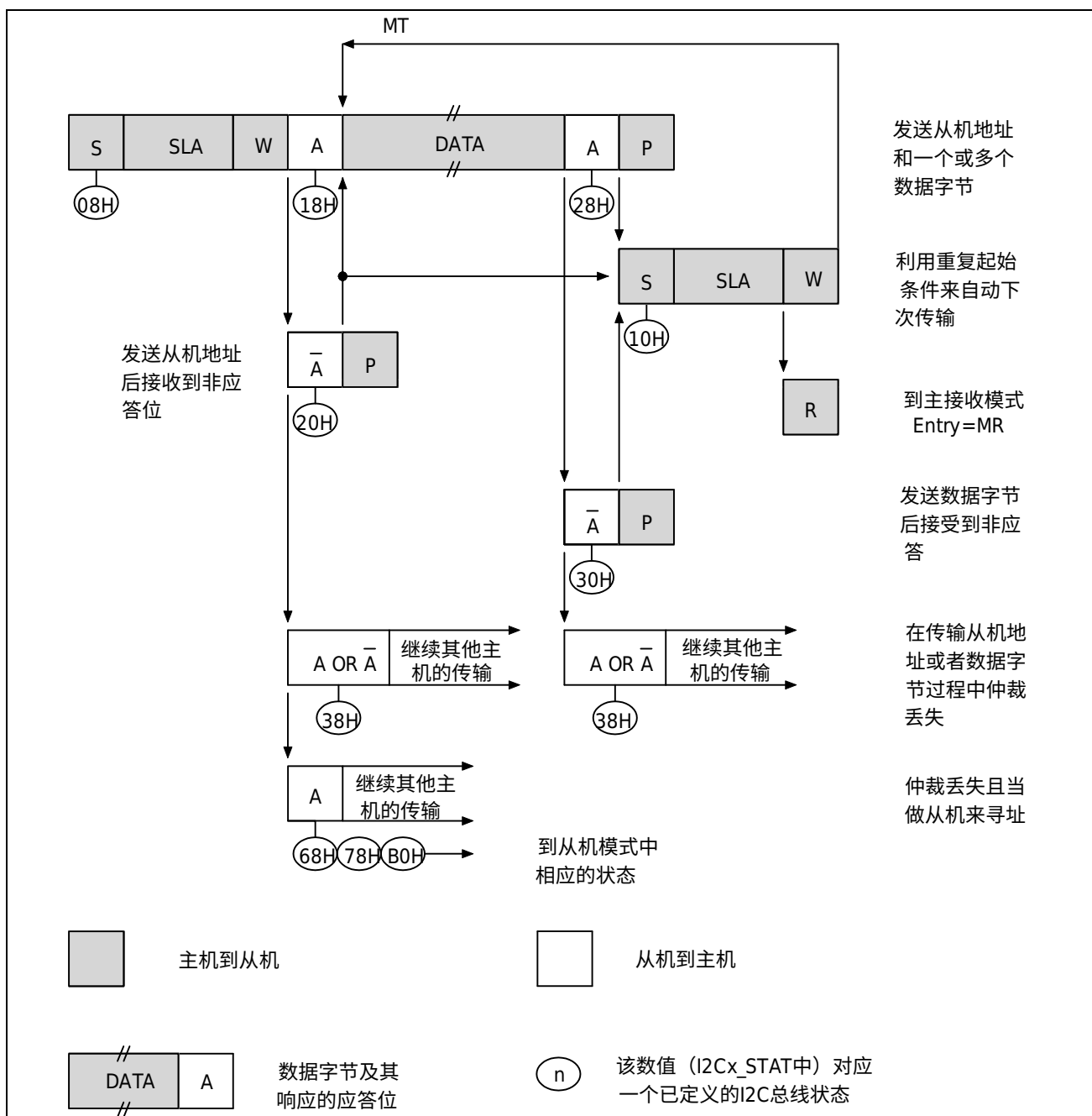
图 7-8 I2C 主机发送状态图
