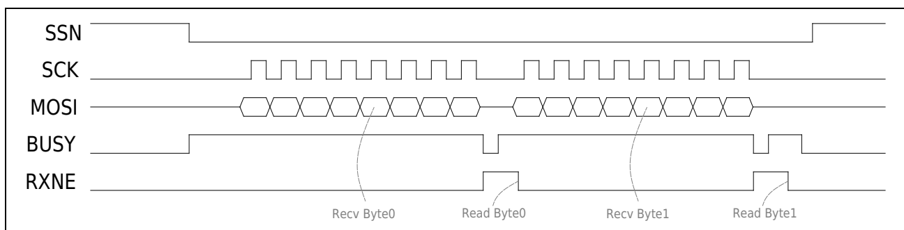
图 8-1 从机接收示意图
