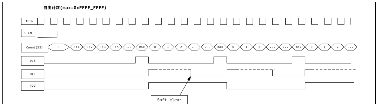
图 13-7 自由计数时序图
