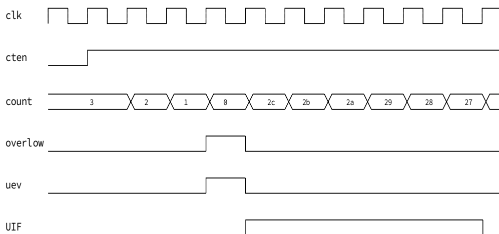
图 13-17 不带预分频的下计数
