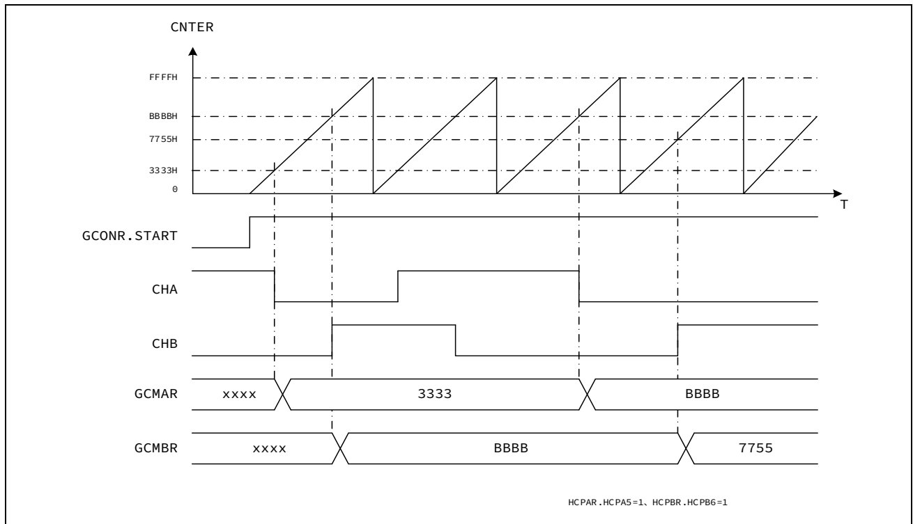
图 15-5 捕获输入动作
