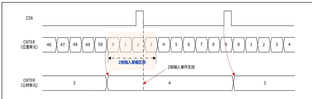
图 15-24 公转计数模式-混合计数 Z 相屏蔽动作例 1
