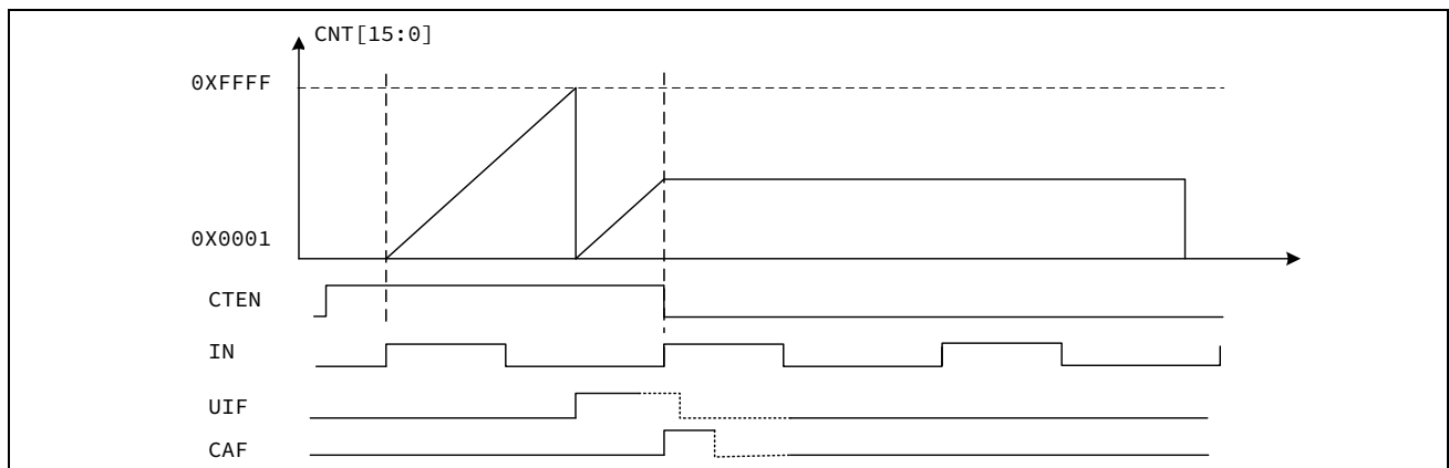
图 13-13 上升沿到上升沿周期测量单次模式
