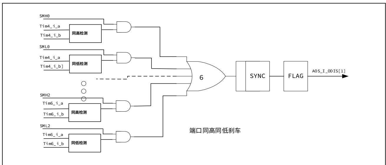
图 15-28 输出同高同低刹车示意图
