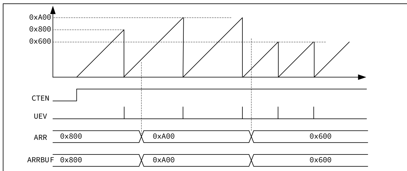
图 13-27 锯齿波模式下上计数缓存无效
