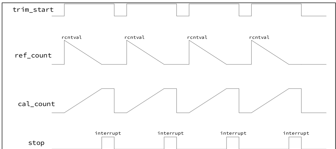
图 9-3 时钟校准波形示意图
