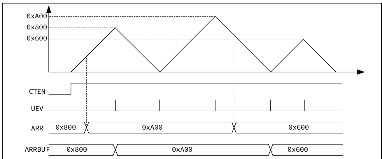
图 13-24 三角波模式下缓存使能
