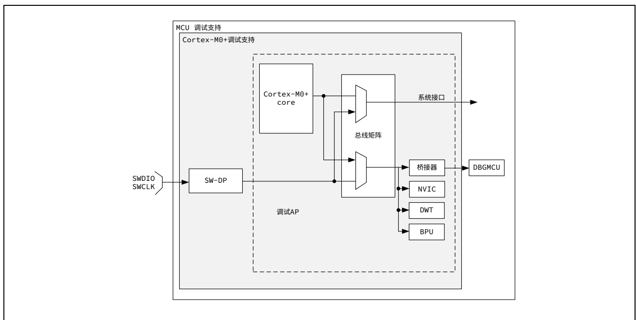
图 28-1 调试支持框图
