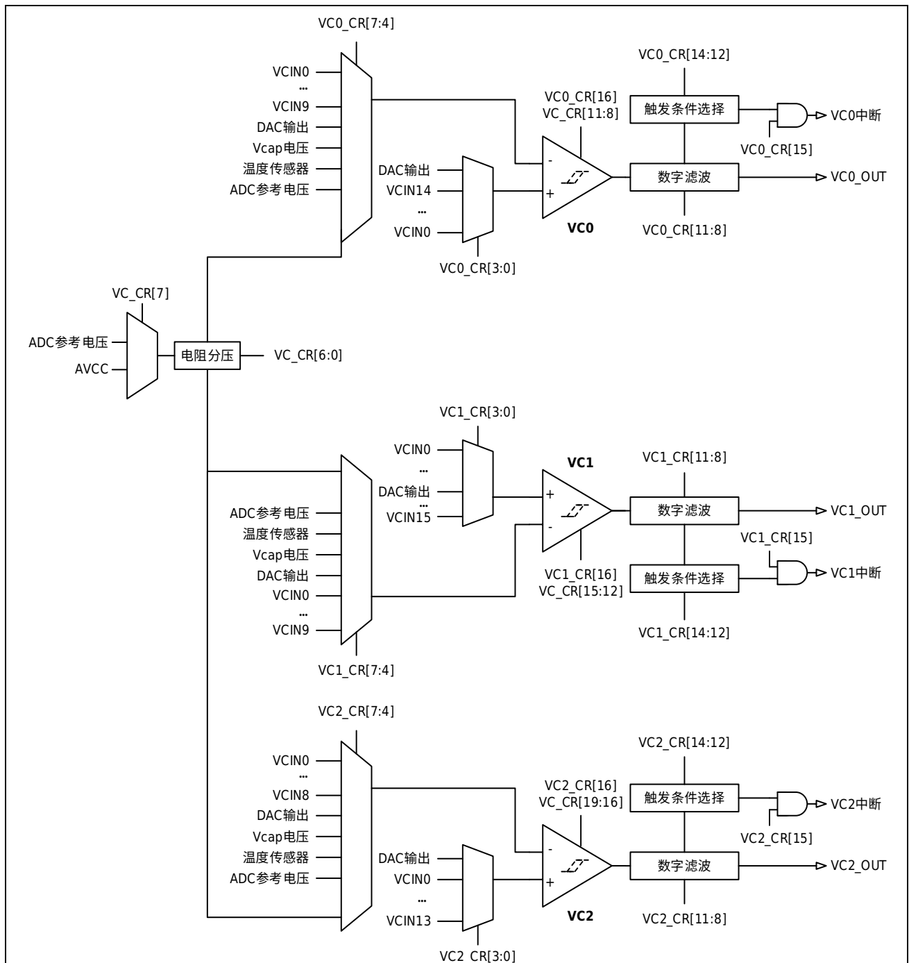
图 24-1 VC 框架图
