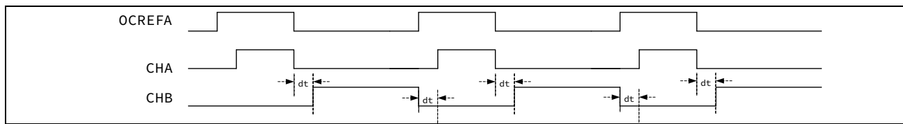
图 13-41 互补 PWM 输出波形图
