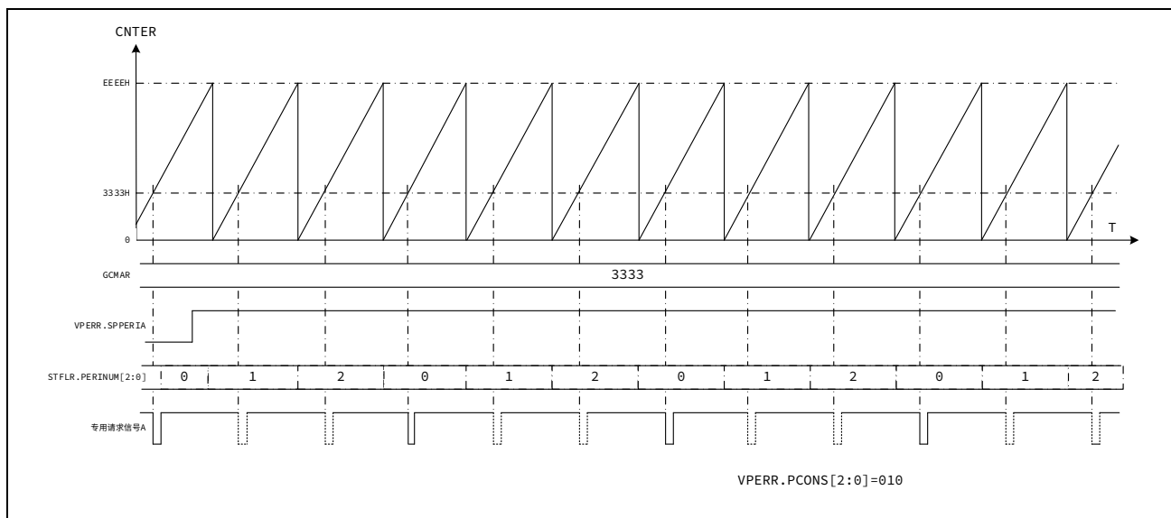
图 15-26 周期间隔有效请求信号动作
