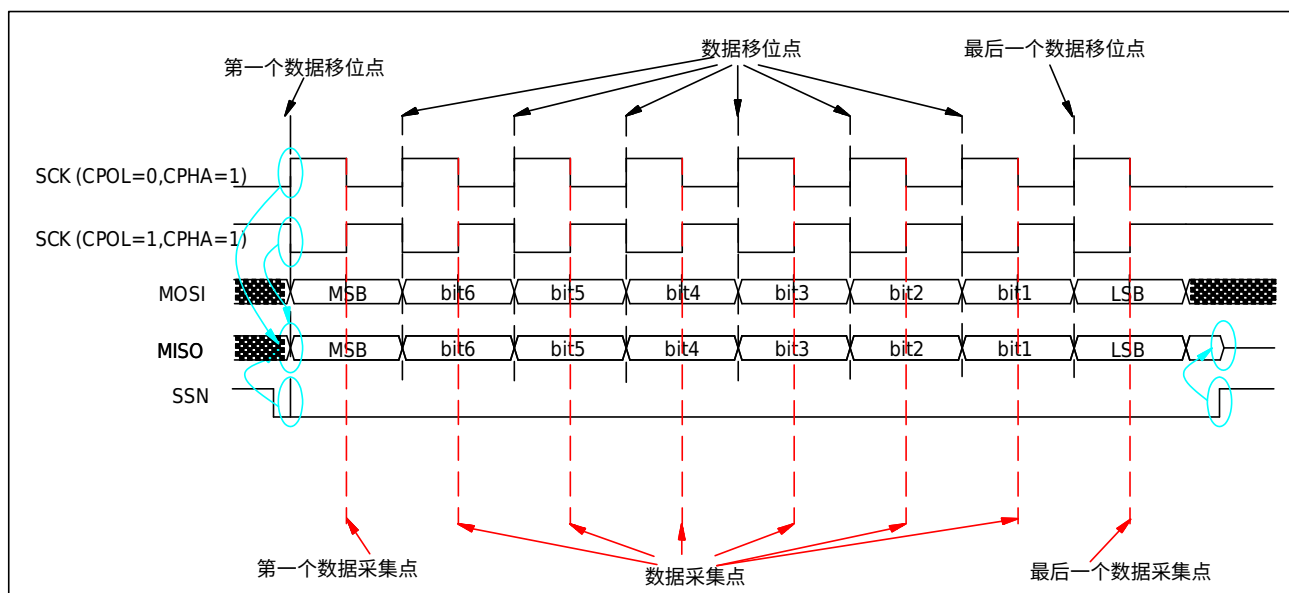
图 8-5 从机 CHPA 为 1 时数据帧格式
