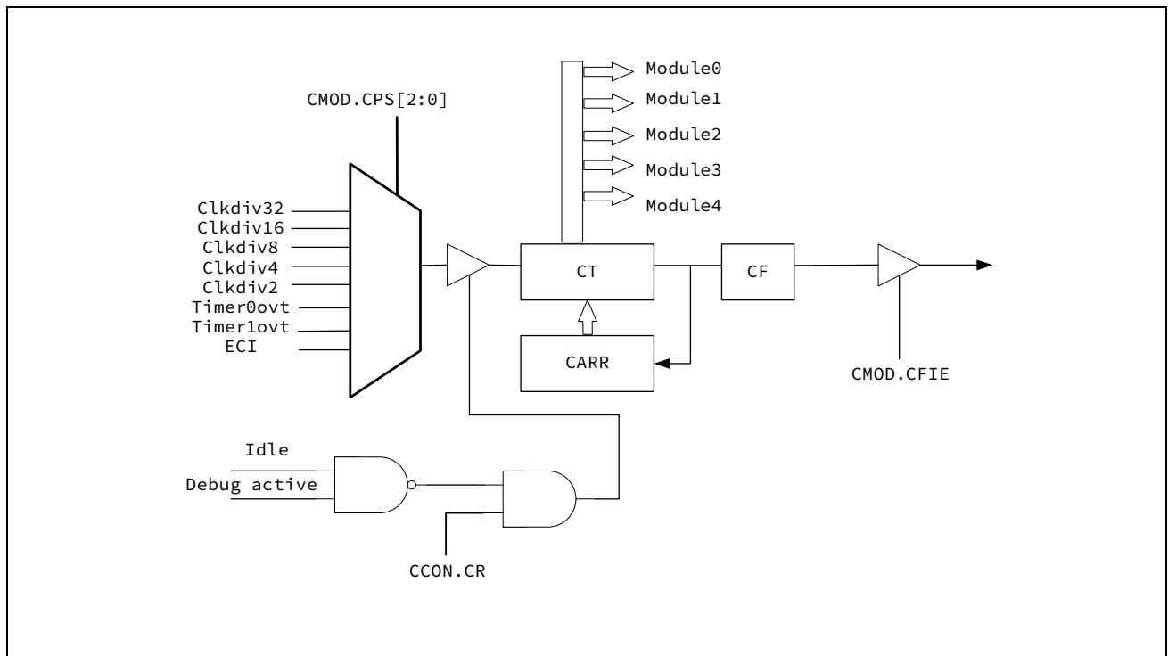
图 14-2 PCA 计数器框图
