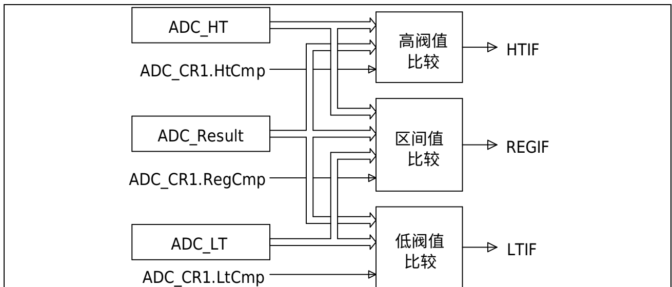
图 28-9 ADC 转换结果
