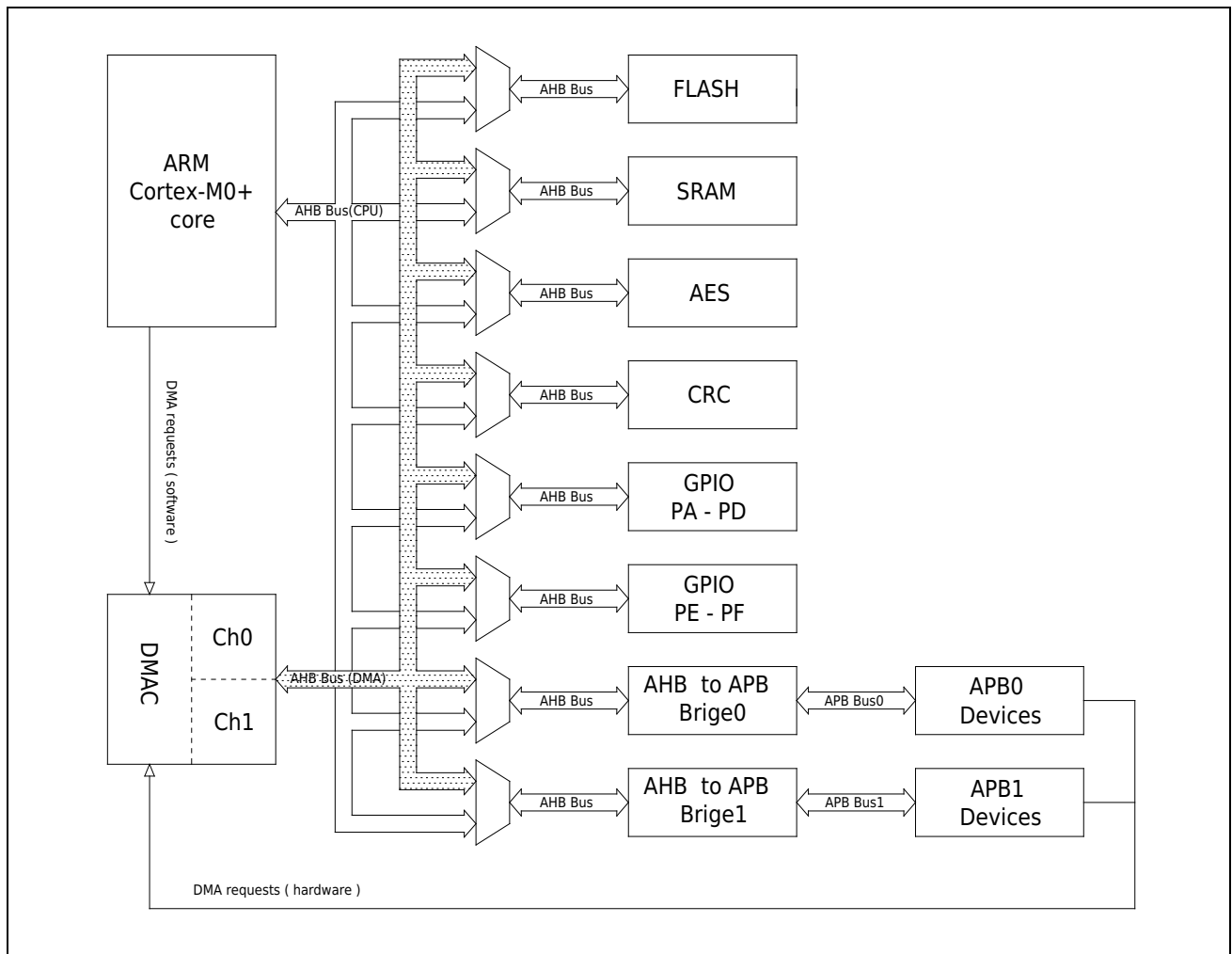
图 12-1 功能框图
