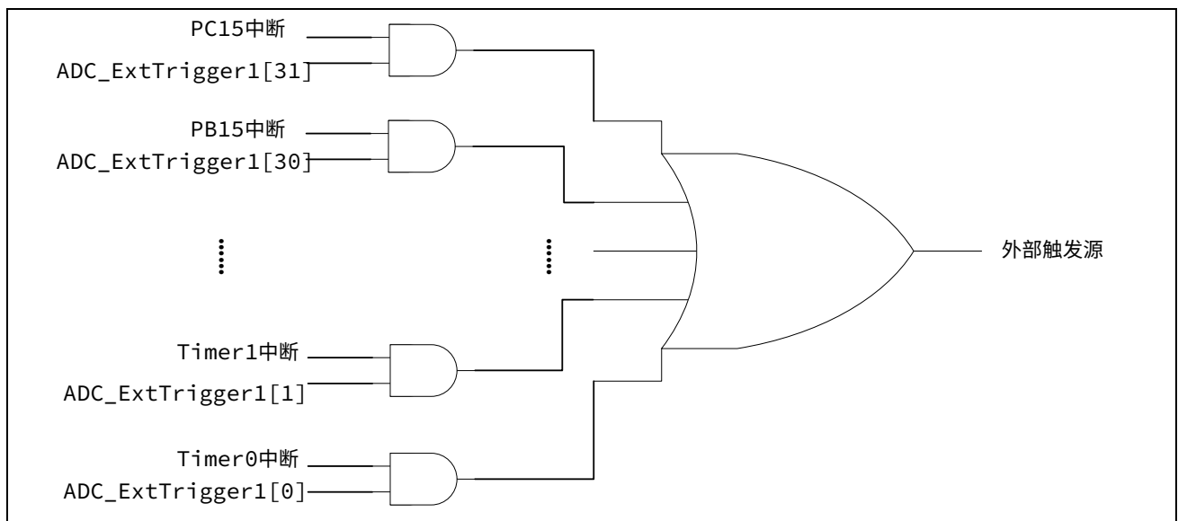
图 22-8 ADC 插队扫描转换外部触发源示意图
