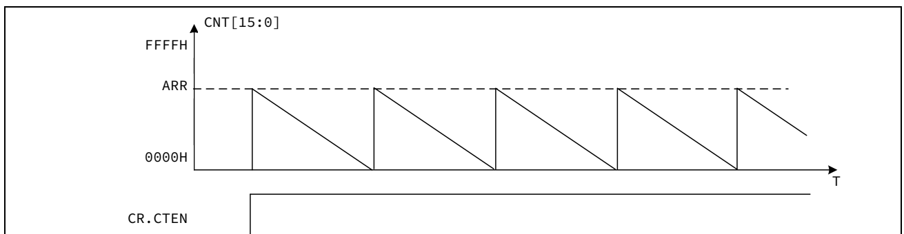
图 13-20 边沿对齐计数器波形 ( DIR =1)
