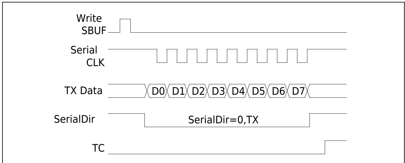
图 17-2 Mode0 发送数据
