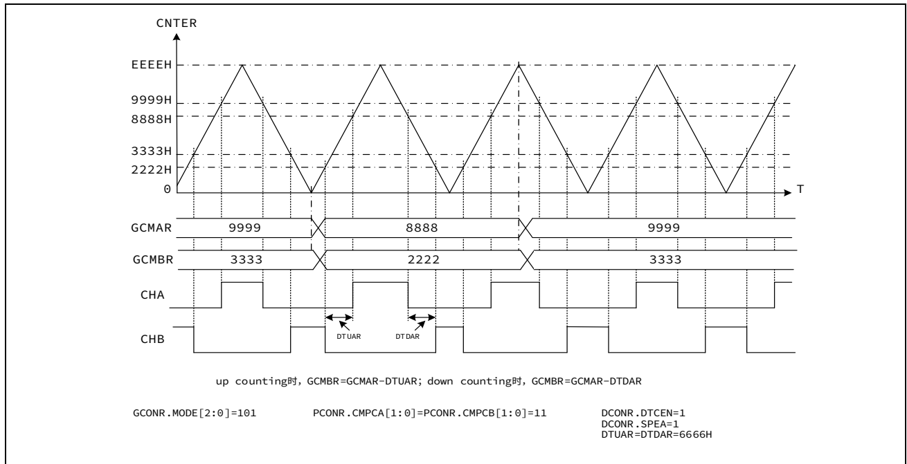
图 15-13 三角波 B 模式时硬件设定 GCMBR 互补 PWM 波输出（对称死区）
