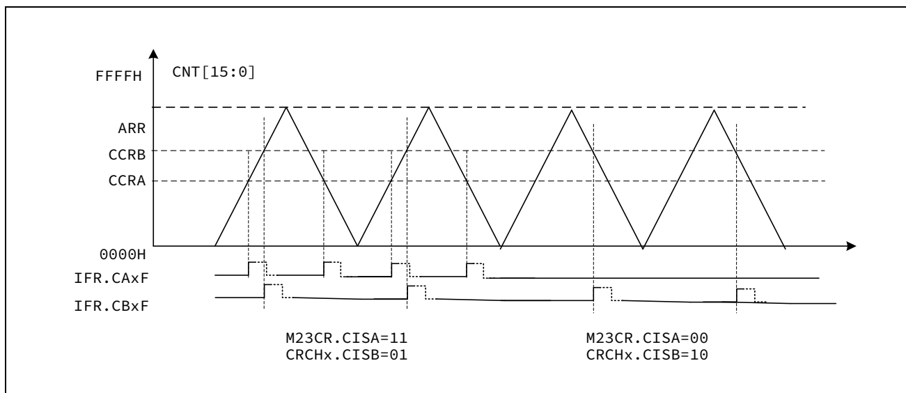
图 13-46 中断示意图
