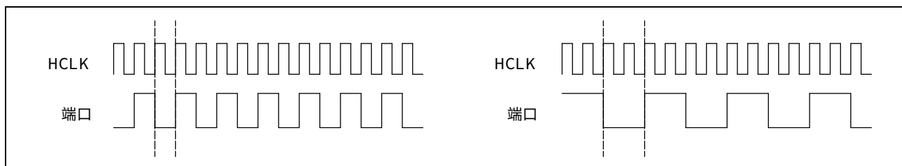
图 6-2 AHB/FASTIO 总线端口随系统时钟的变化
