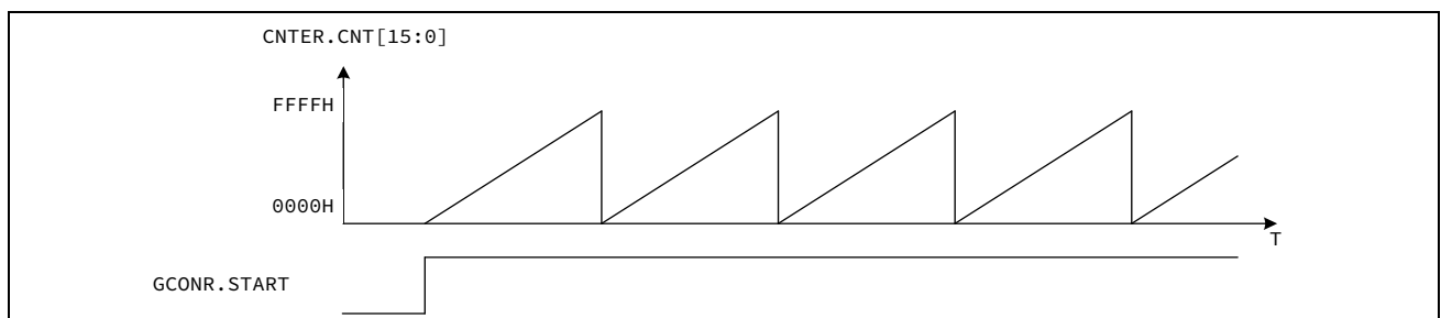
图 15-2 锯齿波波形（递加计数）
