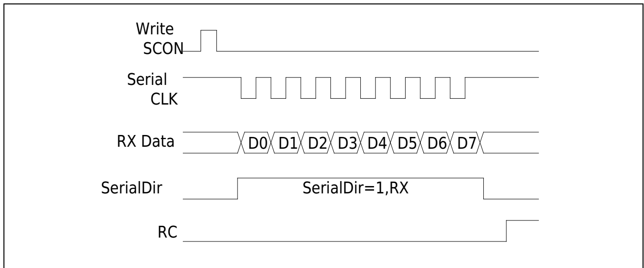
图 17-3 Mode0 接收数据
