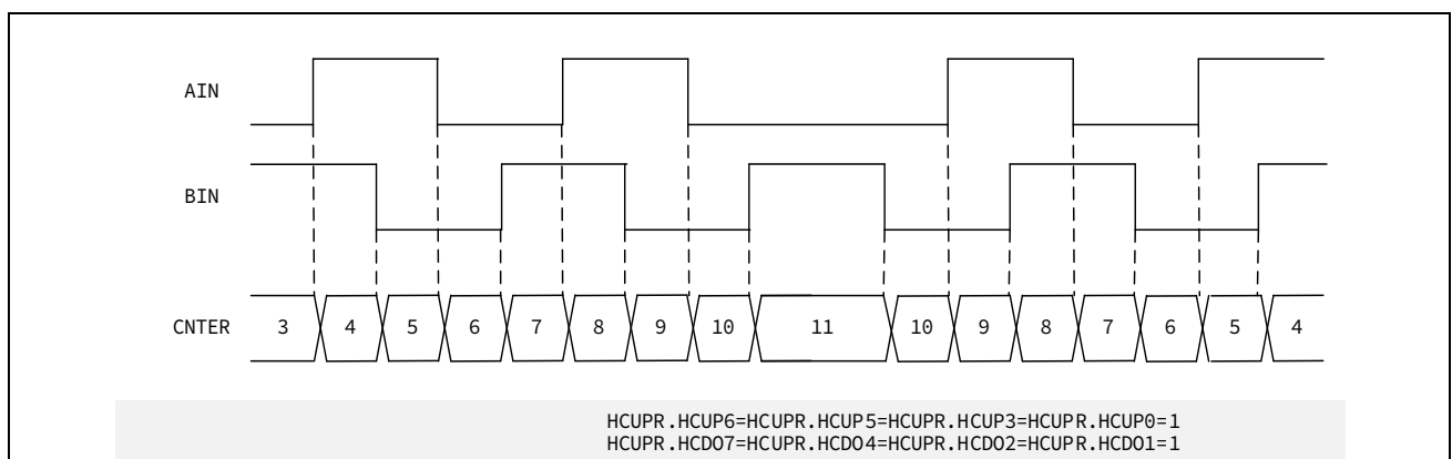
图 15-19 位置模式时相位差计数动作设定 (4 倍)
