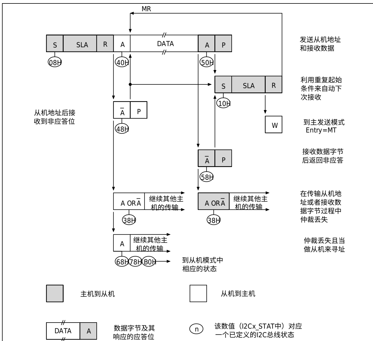
图 7-10 I2C 主机接收状态图
