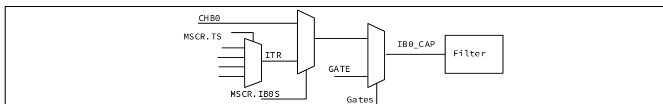
图 13-50 CHB 端口选择
