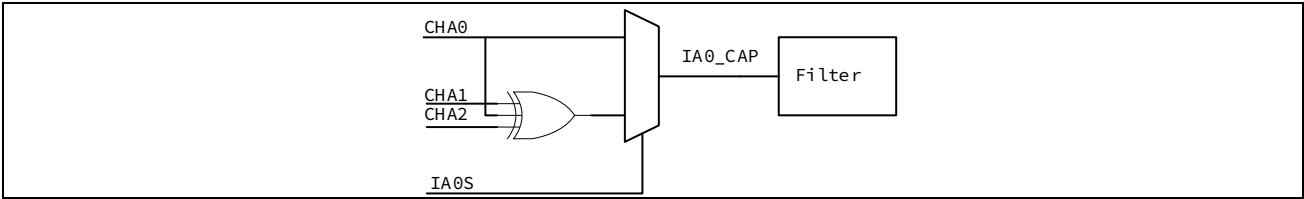
图 13-49 CHA 端口选择
