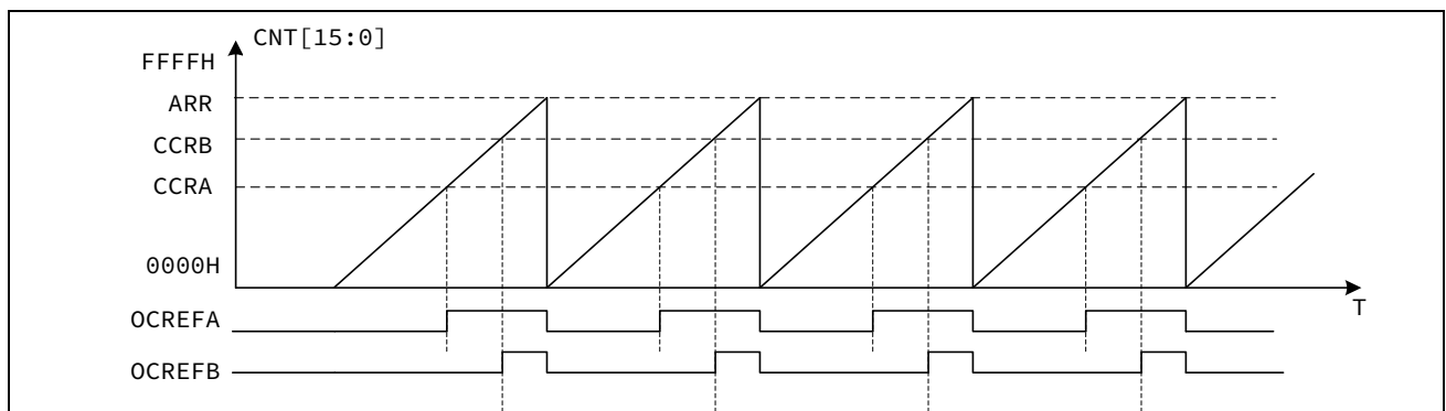
图 13-32 锯齿波计数单点比较 OCREF 输出波形 (OCMx=111)
