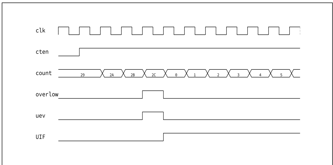
图 13-15 无预分频的向上计数
