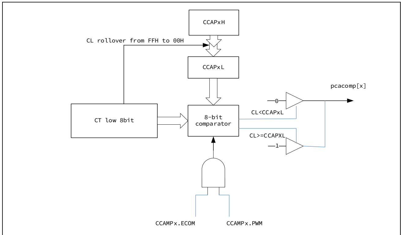
图 14-7 PCA PWM 功能框图
