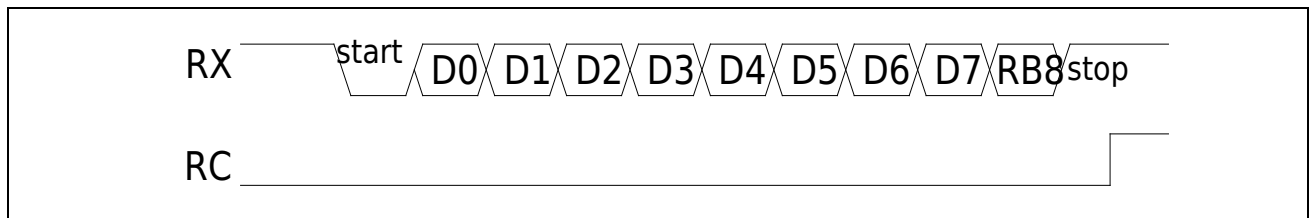
图 17-9 Mode3 接收数据
