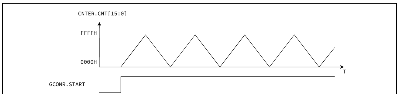
图 15-3 三角波波形
