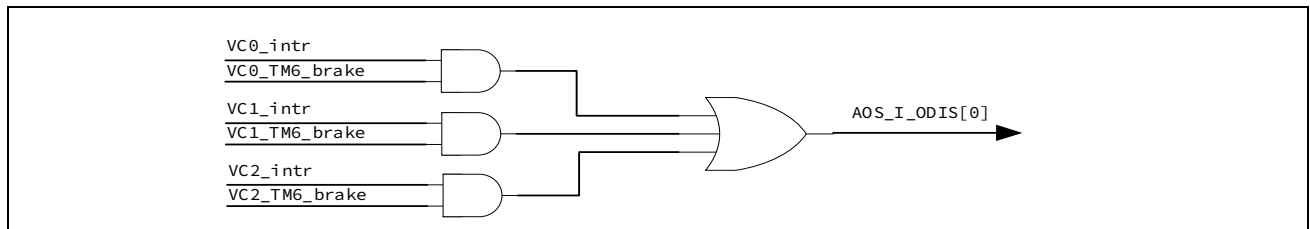
图 15-29 VC 刹车控制示意图
