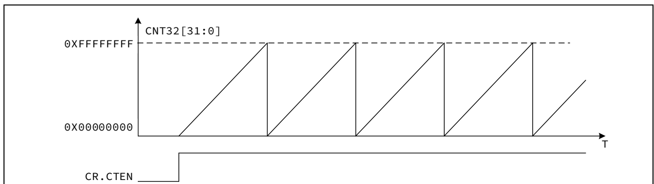
图 13-6 32 位自由计数波形
