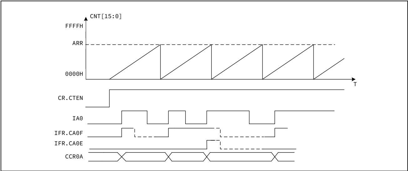
图 13-48 捕获时序图
