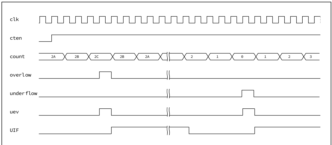
图 13-19 带预分频的上下计数
