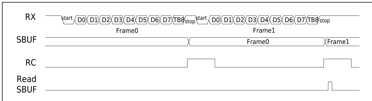
图 17-13 接收缓存
