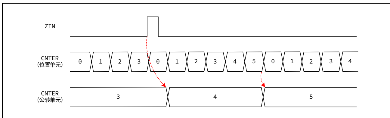
图 15-23 公转模式时 Z 相计数和位置计数器输出混计数动作
