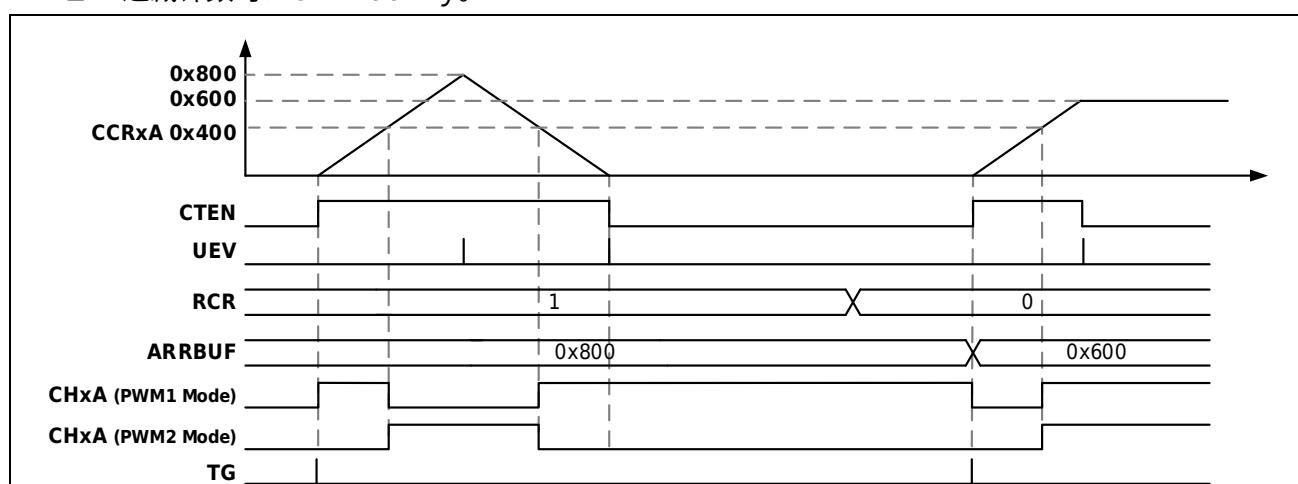
图 13-43 三角波模式单脉冲计数
