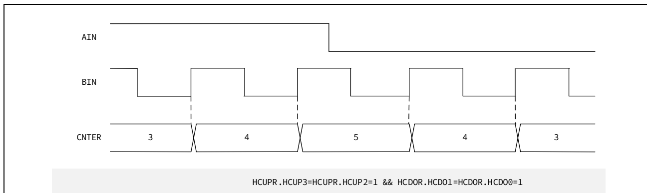
图 15-20 位置模式时方向计数动作
