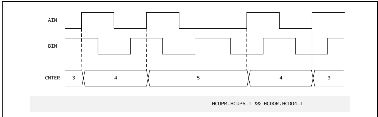
图 15-17 位置模式时相位差计数动作设定 (1 倍)
