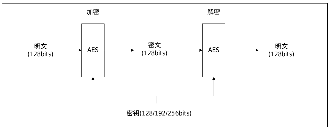
图 20-1 AES 的加解密示意图
