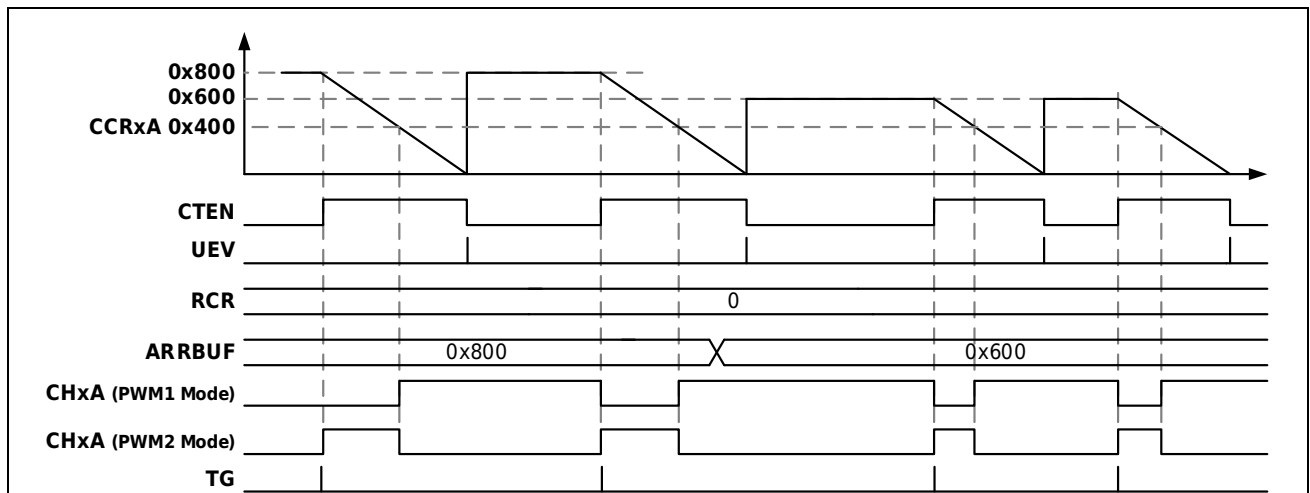
图 13-45 锯齿波下计数单脉冲模式
