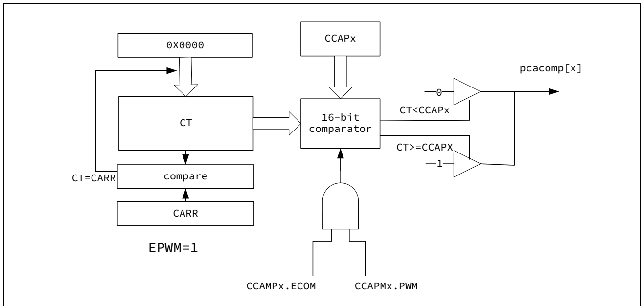
图 14-5 PCA 16 位 PWM 功能框图
