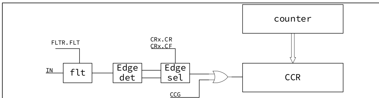
图 13-47 捕获功能框图
