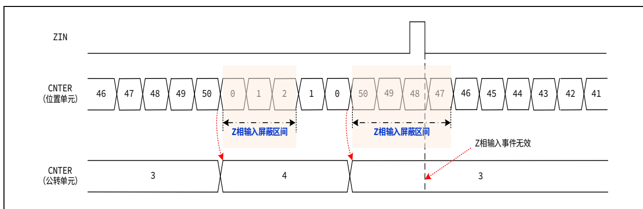
图 15-25 公转计数模式-混合计数 Z 相屏蔽动作例 2
