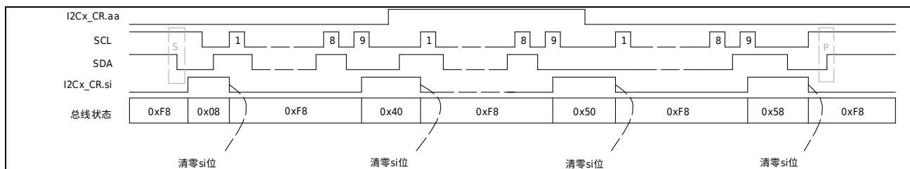
图 7-9 主接收模式数据同步图
