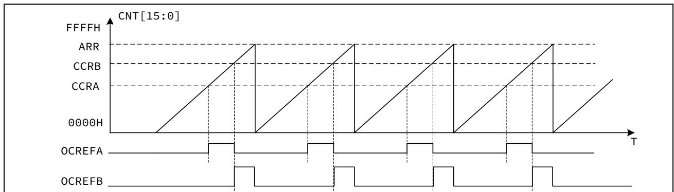
图 13-34 锯齿波计数双点比较 OCREF 输出 (OCMx=111)
