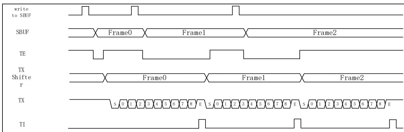
图 16-11 发送缓存
