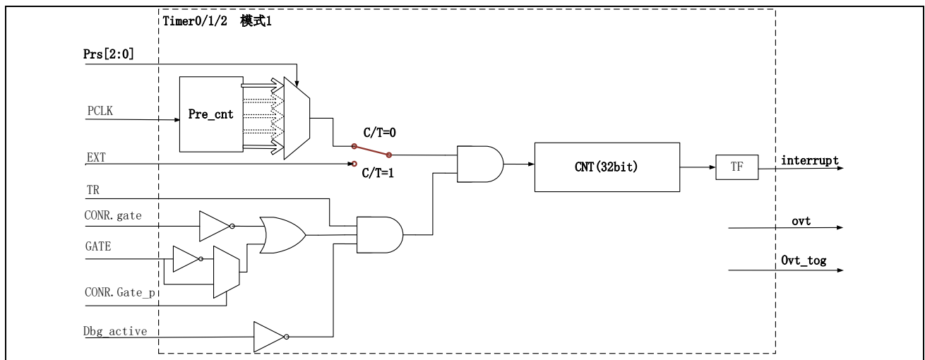
图 9-2 Timer 模式 1 框图
