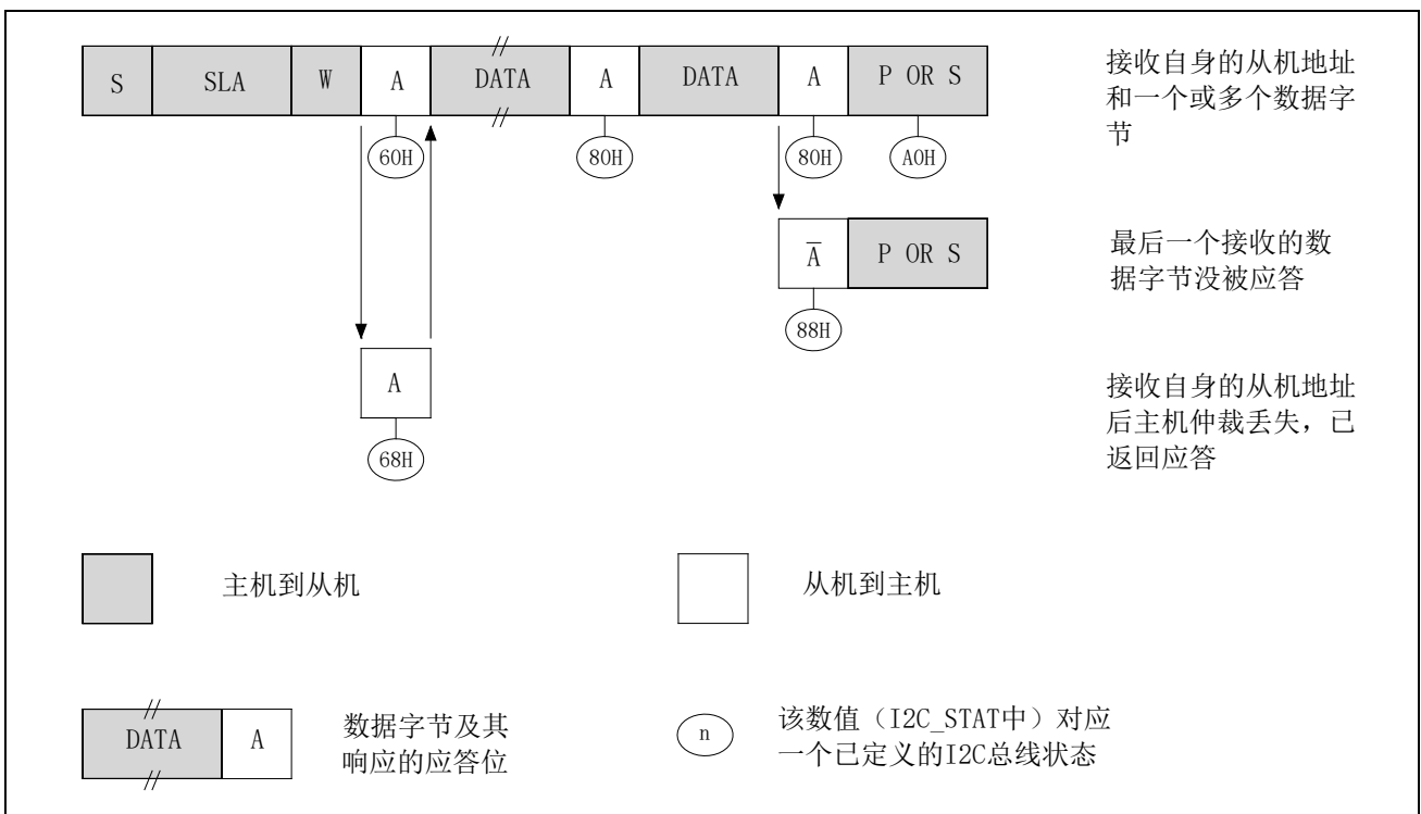
图 17-12 从机接收状态图
