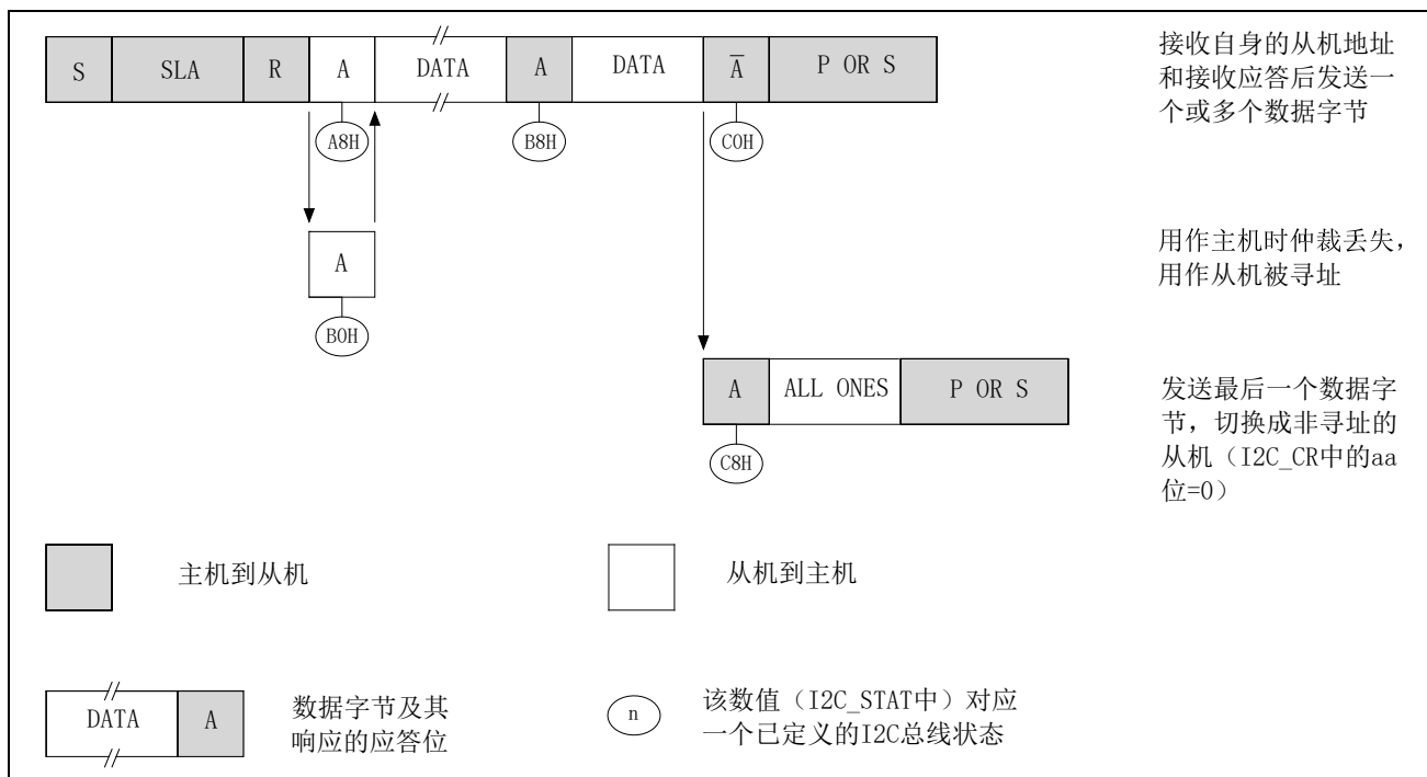
图 17-14 I2C 从机发送状态图
