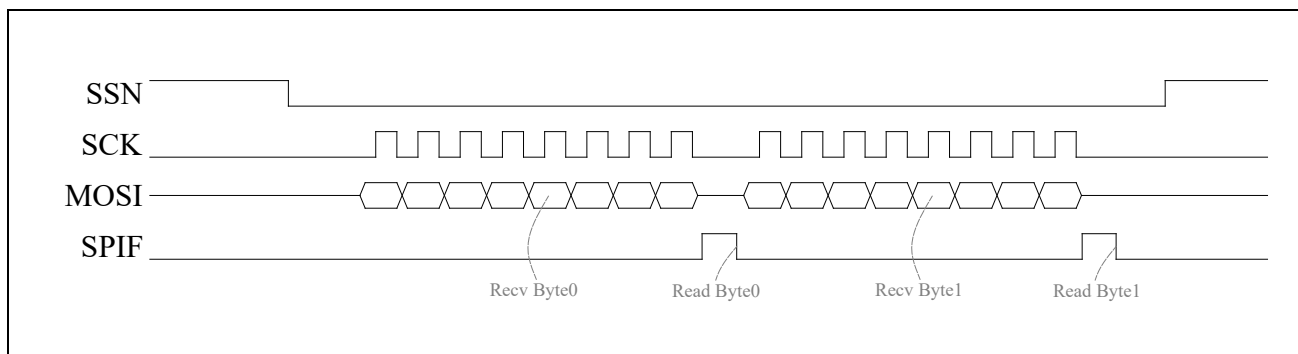
图 18-1 从机接收示意图
