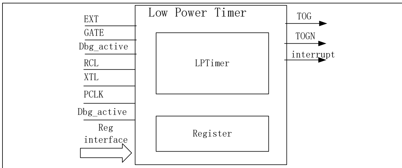
图 10-1 LPTimer 框图
