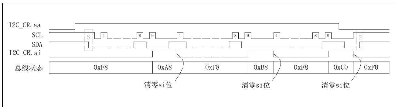
图 17-13 从发送模式数据同步图
