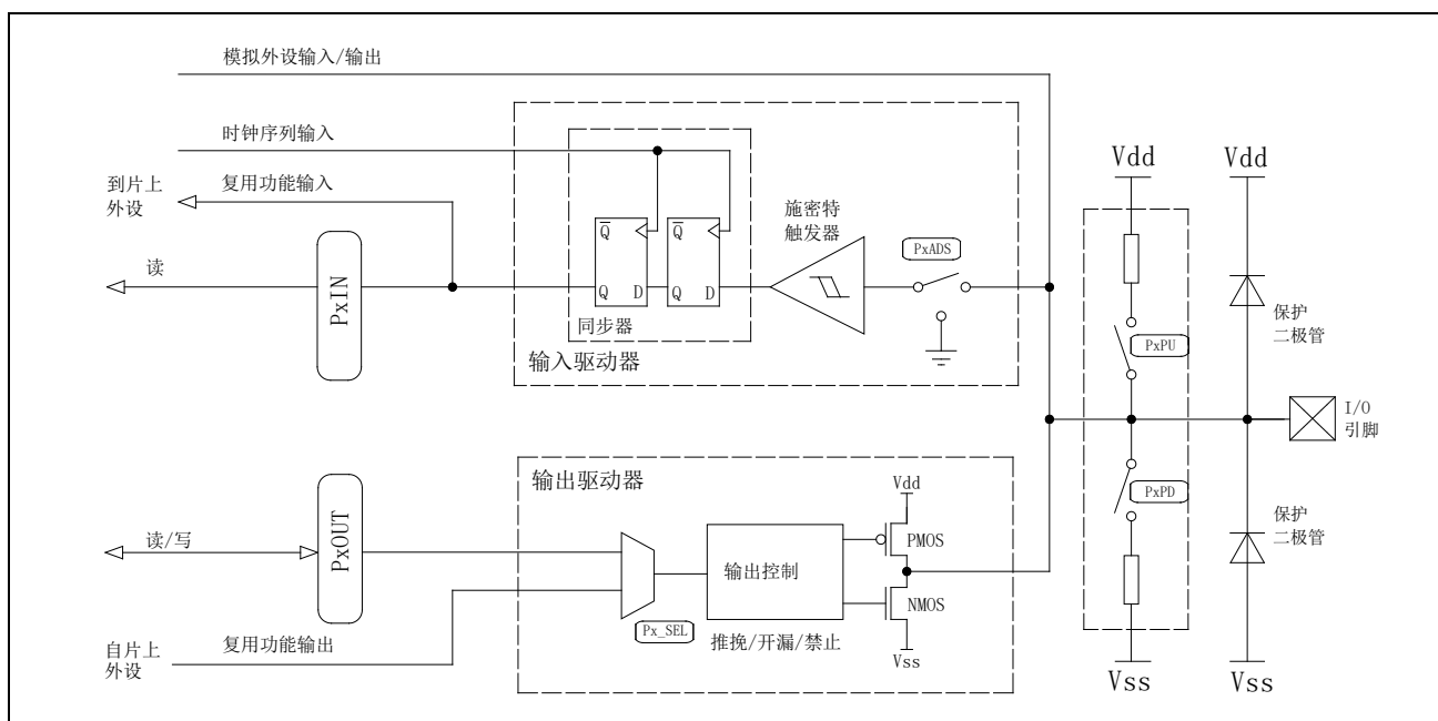
图 6-1 端口电路示意图
