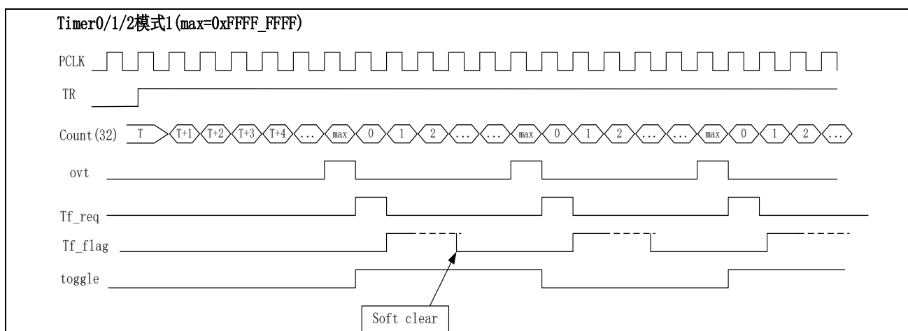
图 9-4 模式 1 时序图
