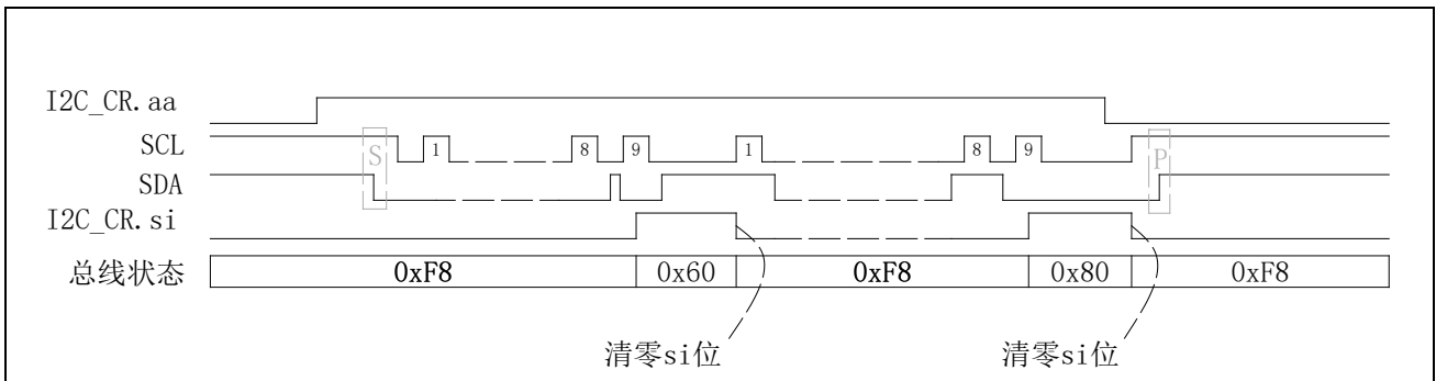
图 17-11 从接收模式数据同步图
