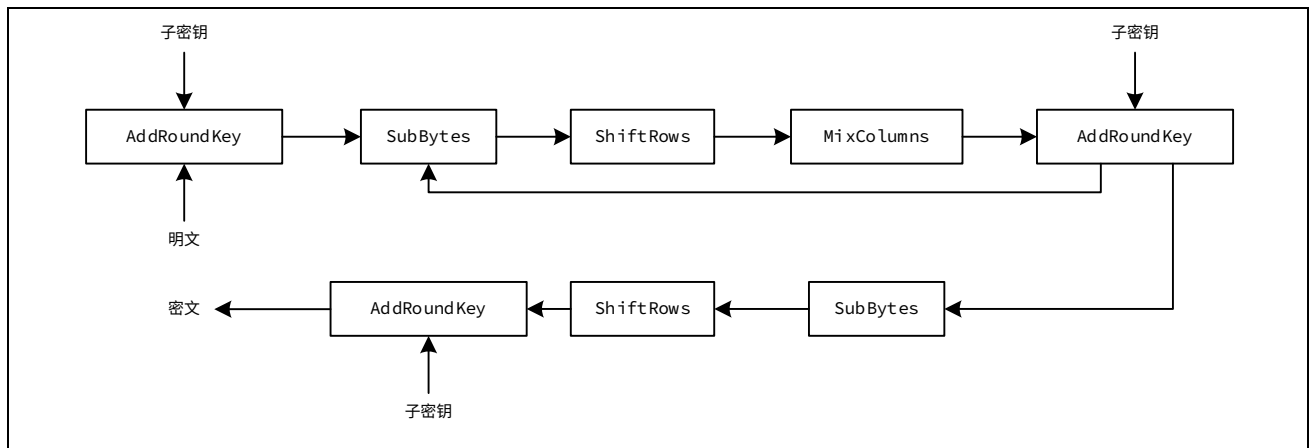
图 24-2 AES 的加密流程图
