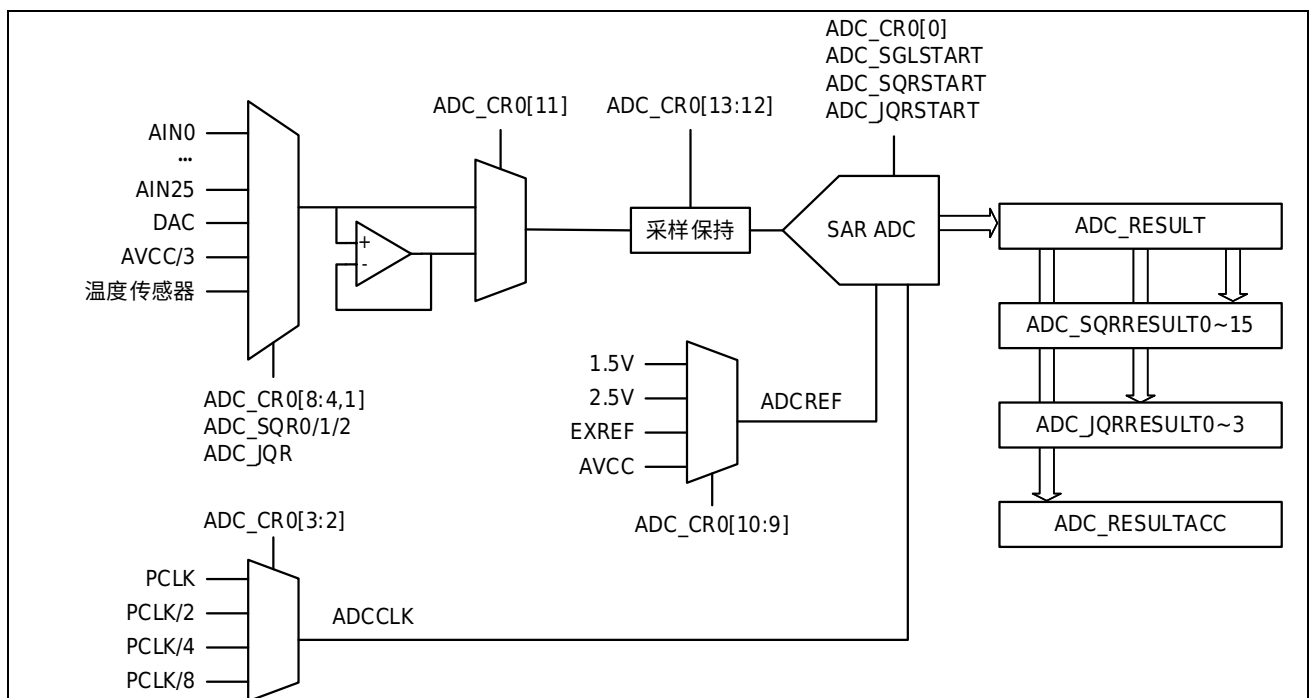
图 26-1 ADC 示意图
