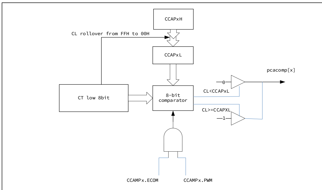
图 15-7 PCA PWM 功能框图
