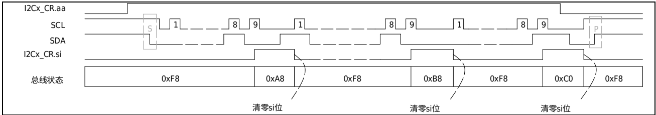
图 7-13 从发送模式数据同步图
