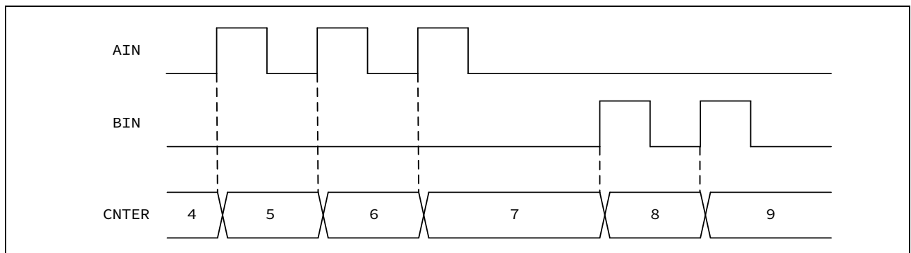
图 16-16 位置模式时基本计数动作
