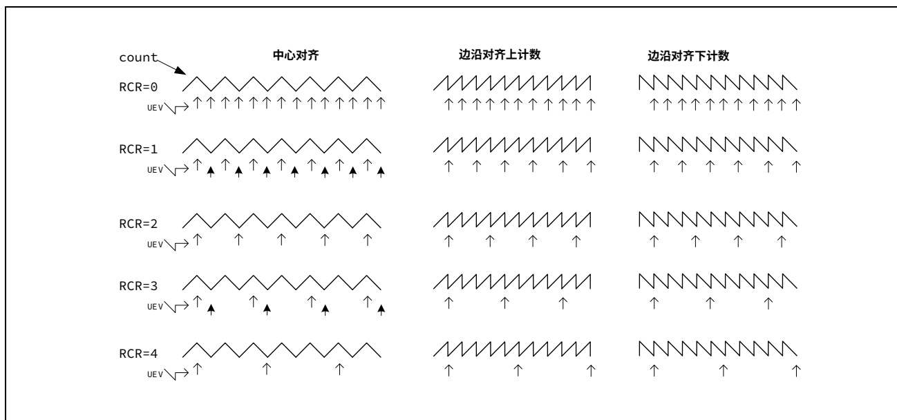
图 13-23 重复计数器产生更新时序
