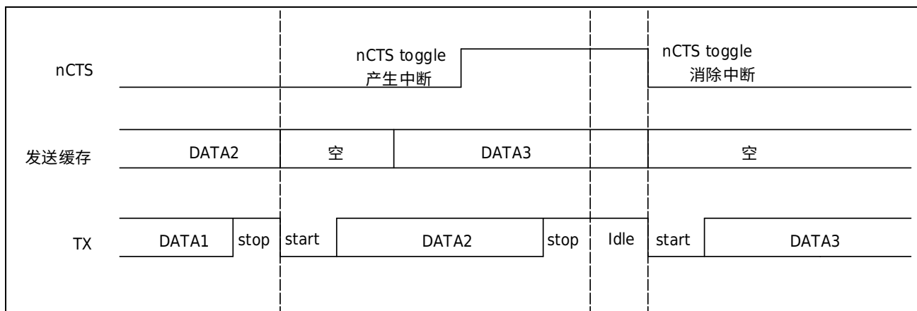
图 21-12 nCTS 硬件流控信号
