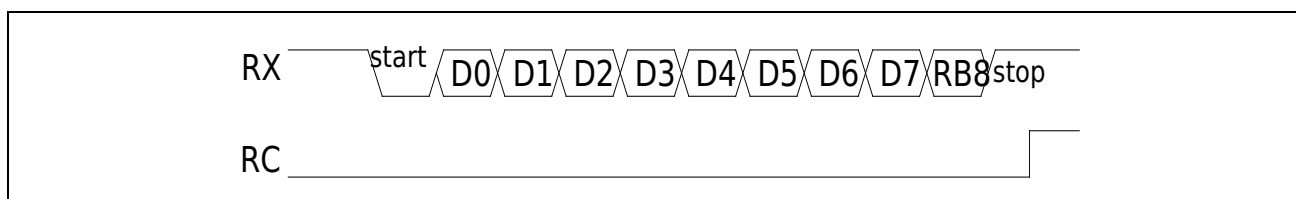
图 21-9 Mode3 接收数据
