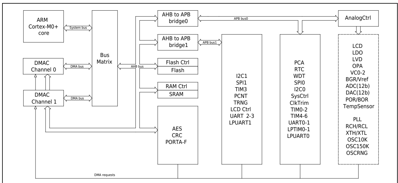
图 1-1 系统架构示意图
