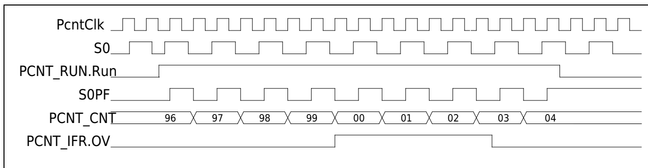
图 19-2 单通道脉冲计数模式加计数波形
