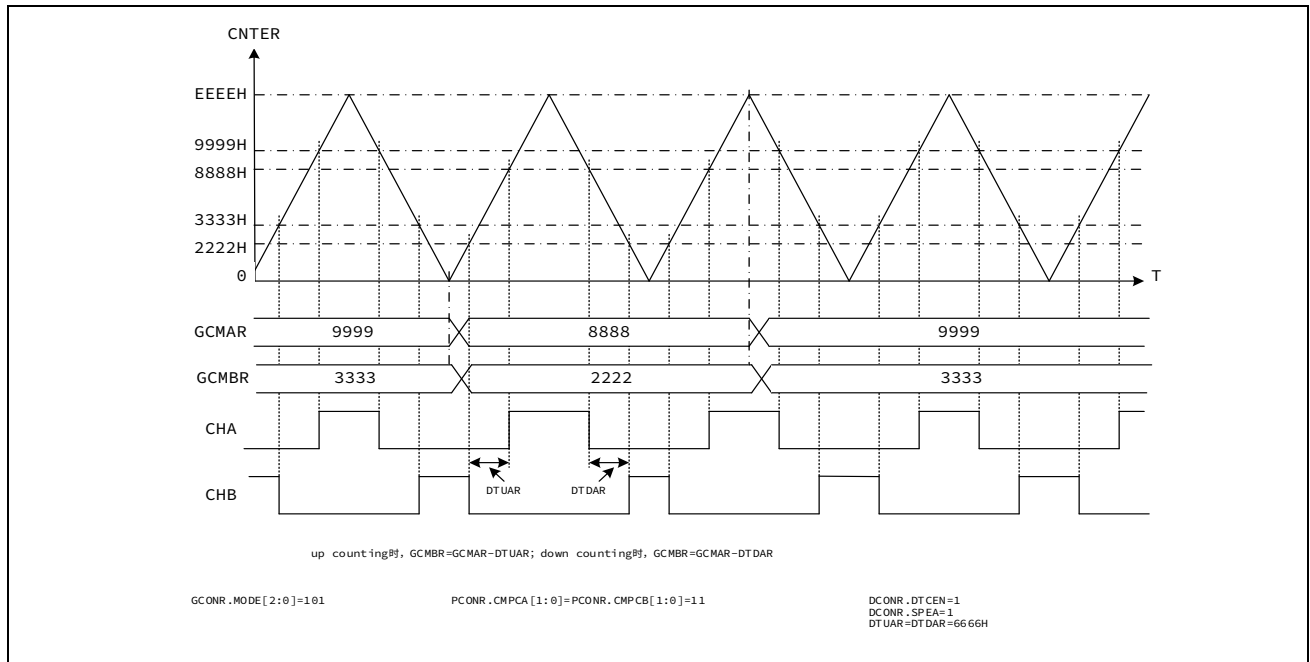
图 16-13 三角波 B 模式时硬件设定 GCMBR 互补 PWM 波输出（对称死区）
