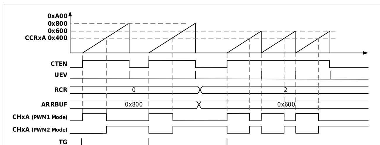
图 13-44 锯齿波上计数单脉冲模式
