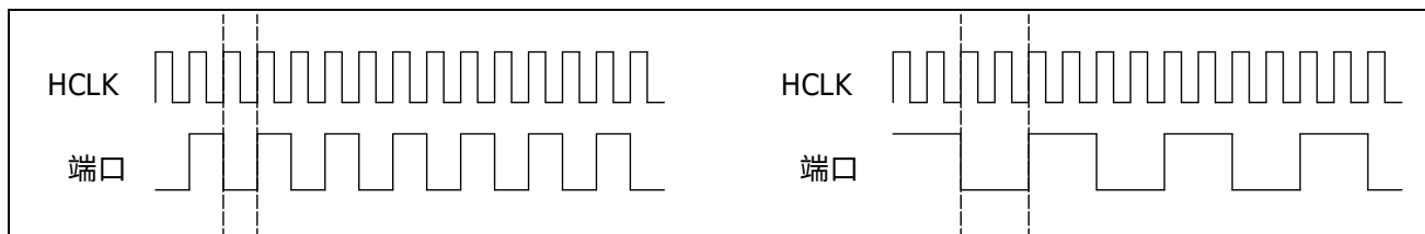
图 6-2 AHB/FASTIO 总线端口随系统时钟的变化
