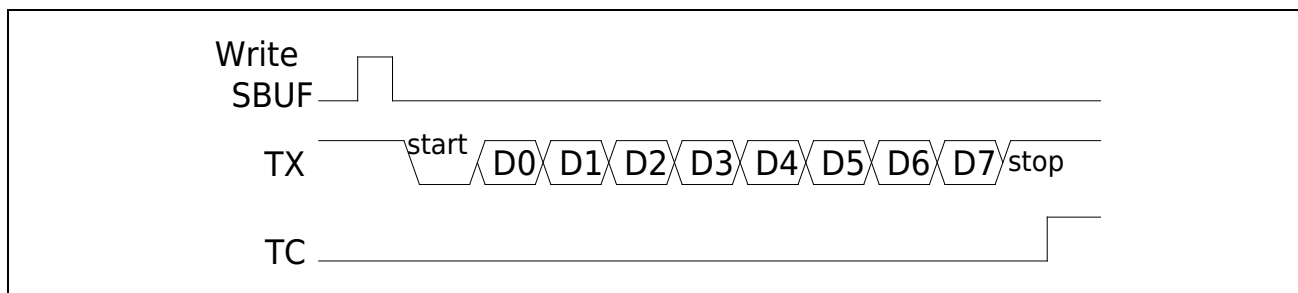
图 21-4 Mode1 发送数据
