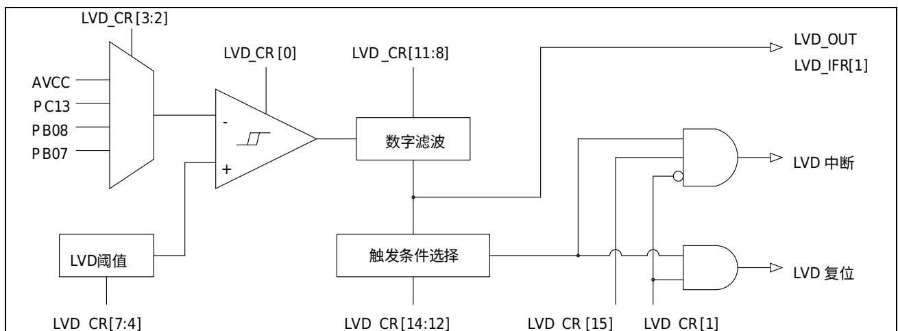
图 29-1 LVD 框图
