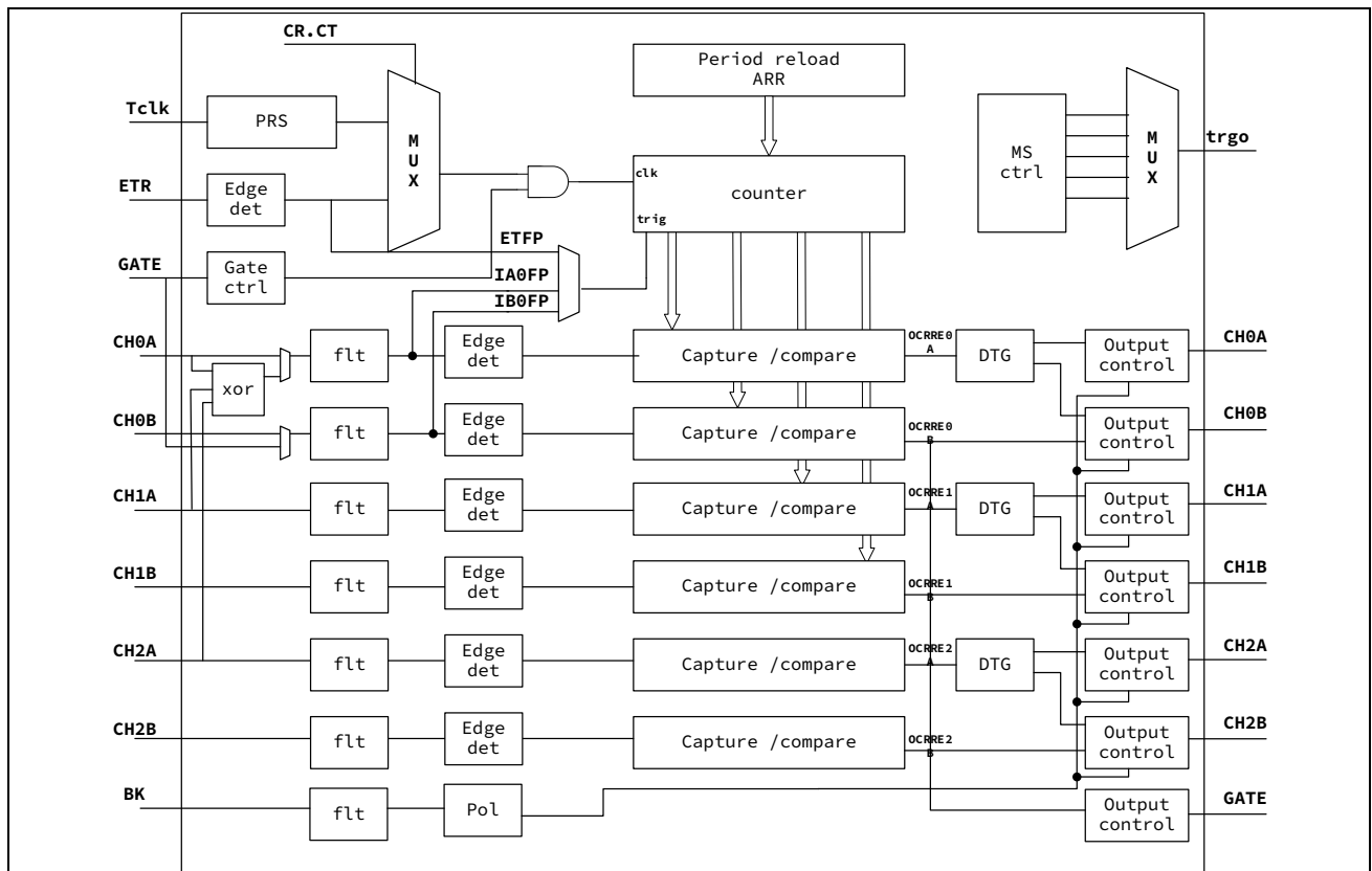
图 13-2 TIM3 框图
