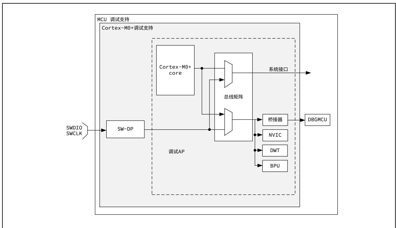
图 32-1 调试支持框图
