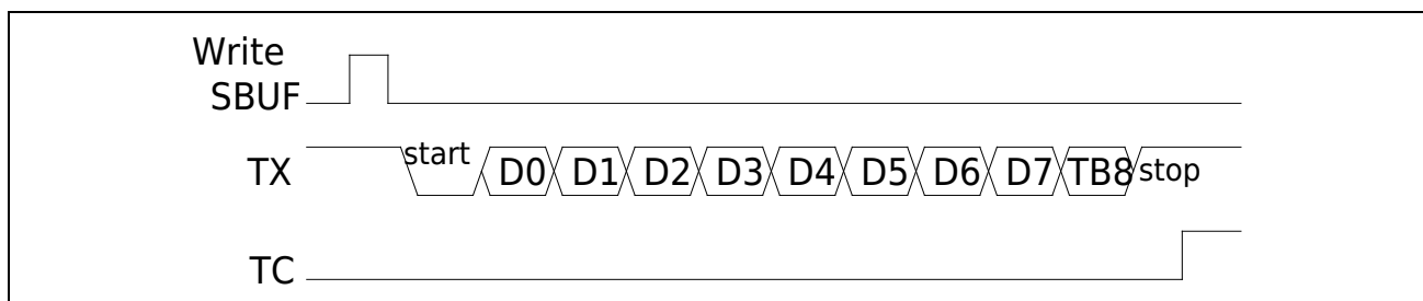
图 21-6 Mode2 发送数据
