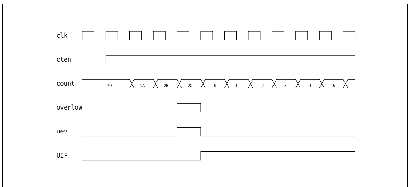
图 13-15 无预分频的向上计数
