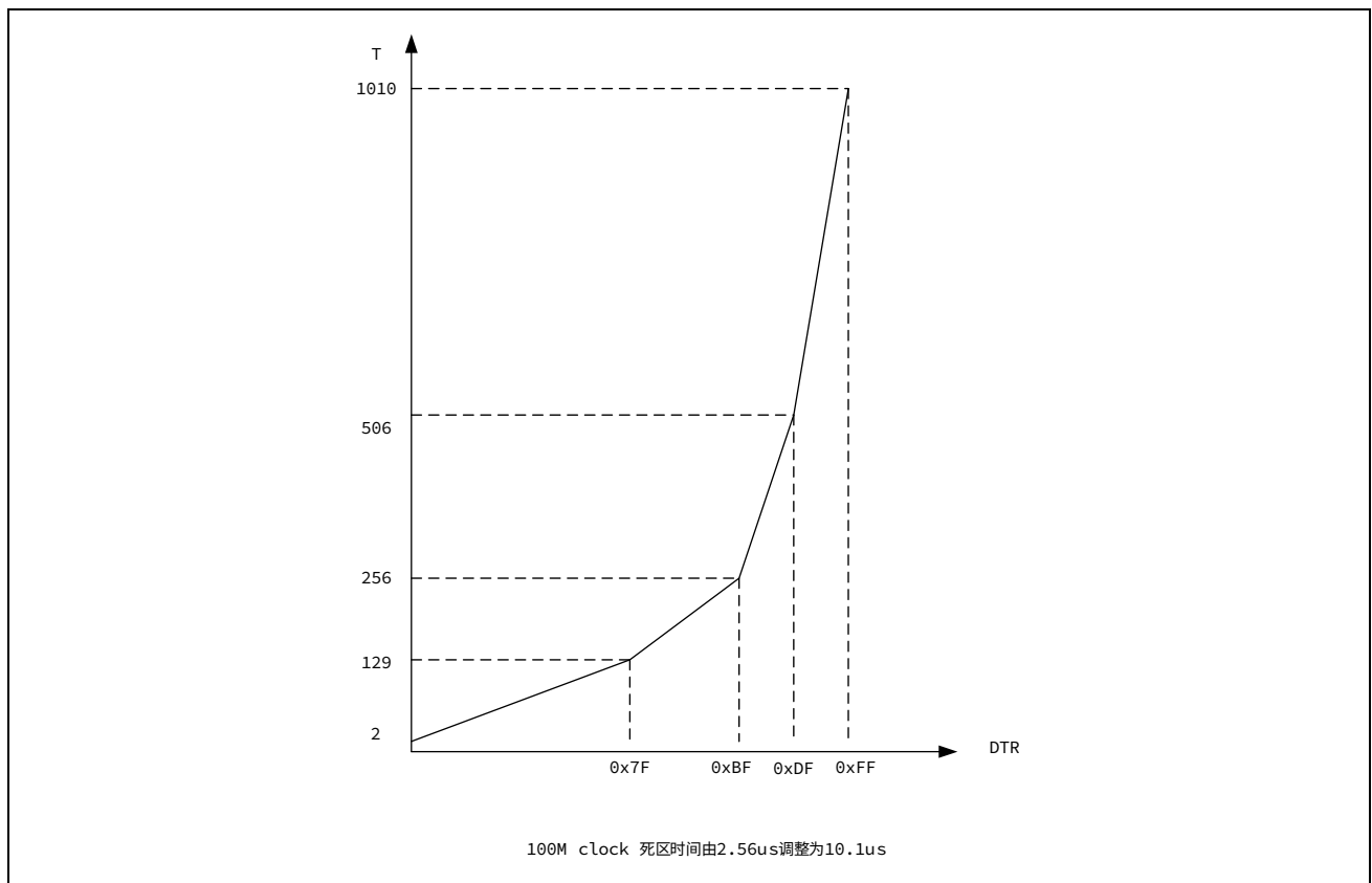
图 13-42 死区时间
