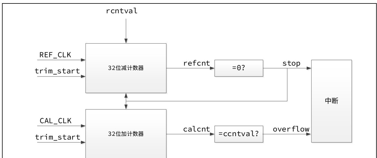
图 9-2 时钟校准模块硬件示意图
