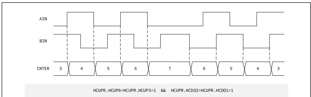
图 16-18 位置模式时相位差计数动作设定 (2 倍)
