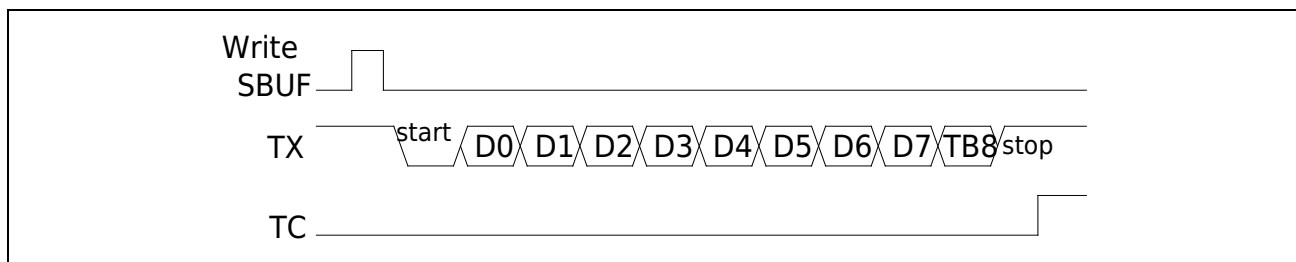
图 21-8 Mode3 发送数据
