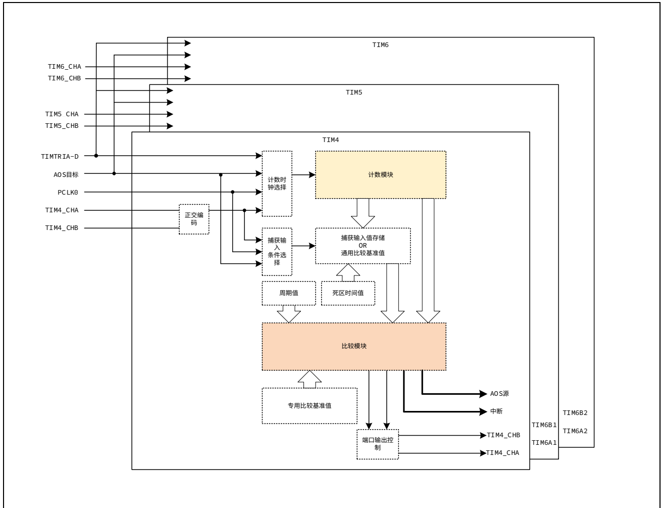
图 16-1 Advanced Timer 框图
