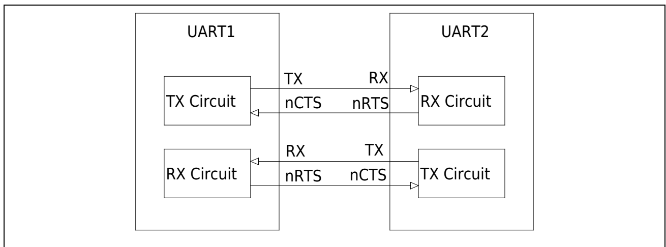
图 20-10 UART 硬件流控
