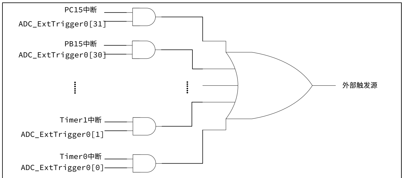
图 26-7 ADC 单次转换或顺序扫描转换外部触发源示意图
