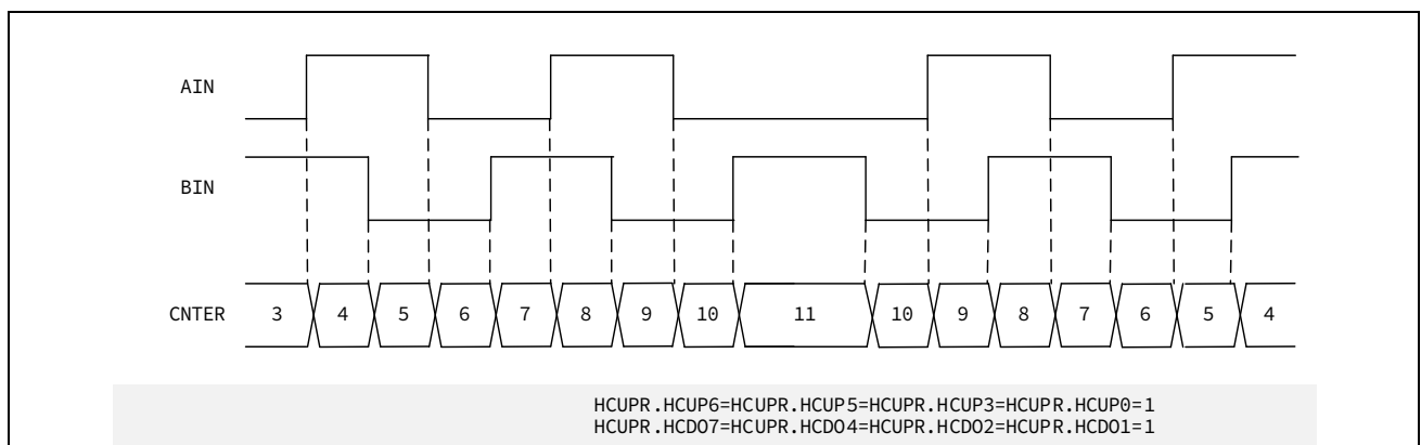
图 16-19 位置模式时相位差计数动作设定 (4 倍)
