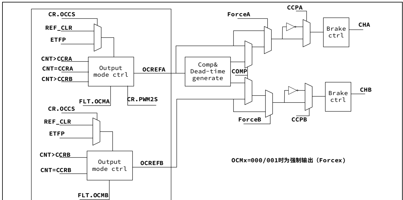
图 13-31 OCREF 输出框图
