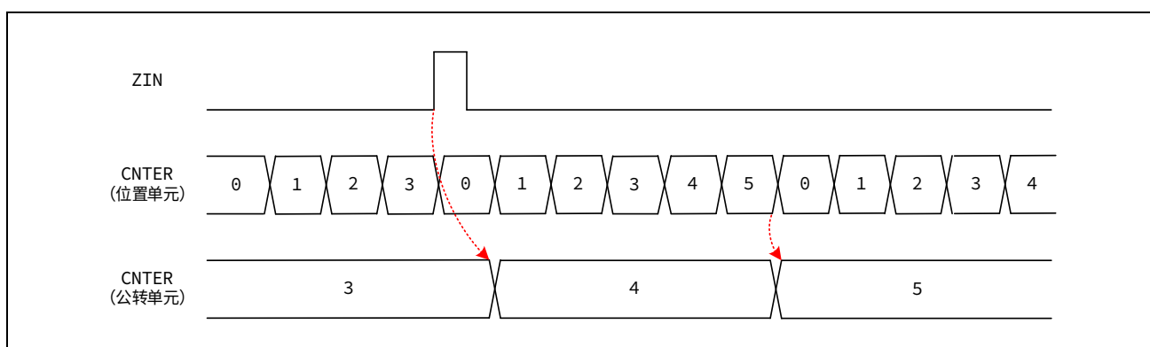
图 16-23 公转模式时 Z 相计数和位置计数器输出混合同步计数动作
