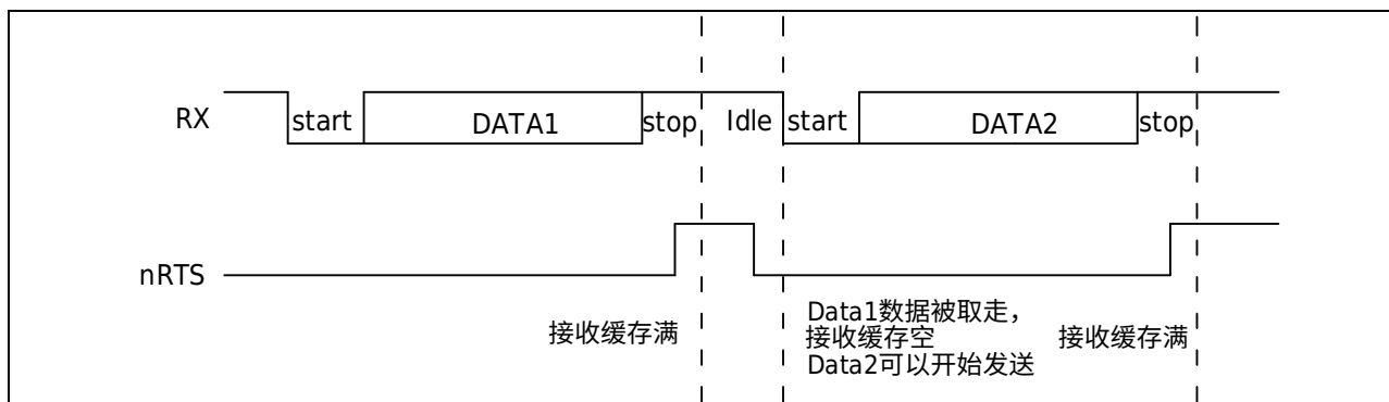
图 21-11 nRTS 硬件流控信号
