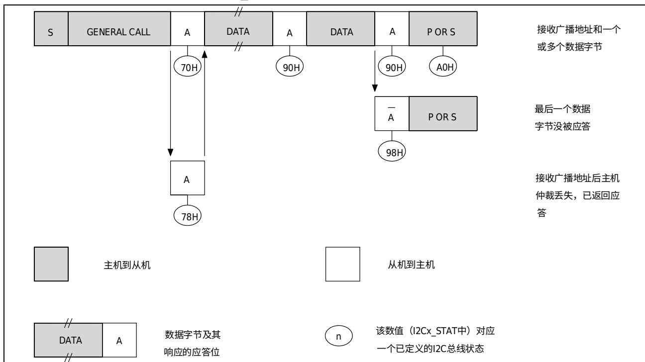
图 7-15 I2C 广播呼叫状态图
