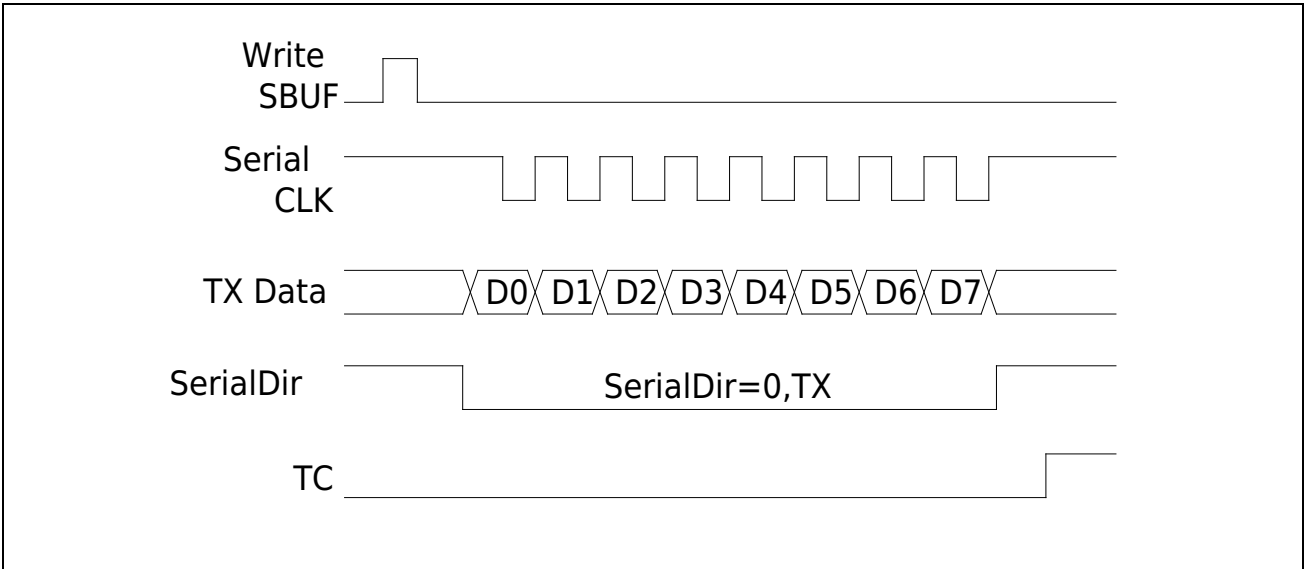
图 20-2 Mode0 发送数据
