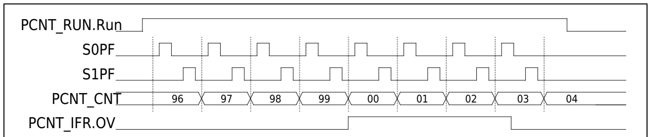
图 19-4 双通道非交脉冲计数模式加计数波形
