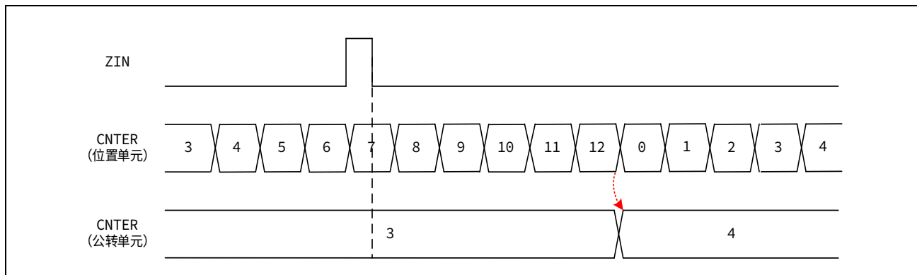
图 16-22 公转模式时位置计数器输出计数动作
