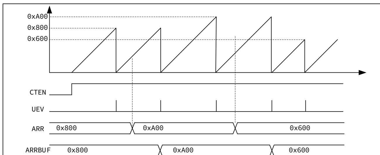
图 13-26 锯齿波模式下上计数缓存使能
