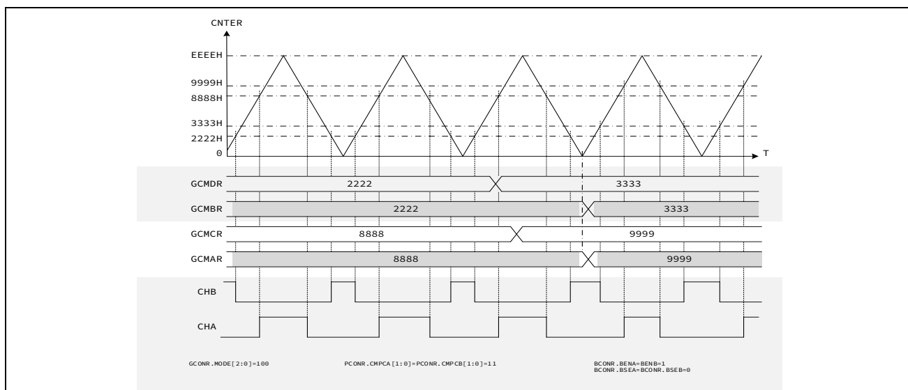
图 16-12 三角波 A 模式时软件设定 GCMBR 互补 PWM 波输出
