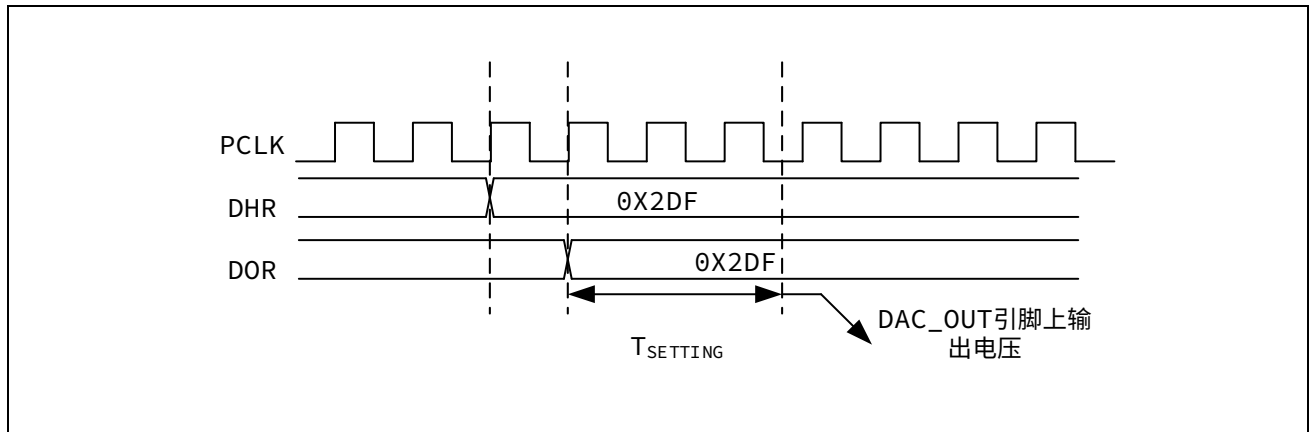
图 27-1 触发不使能时 DAC 转换时序图
