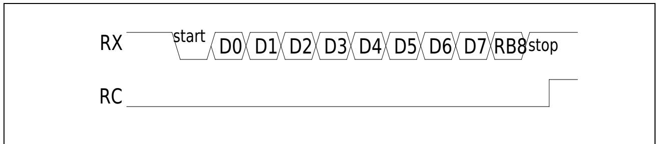
图 20-7 Mode2 接收数据
