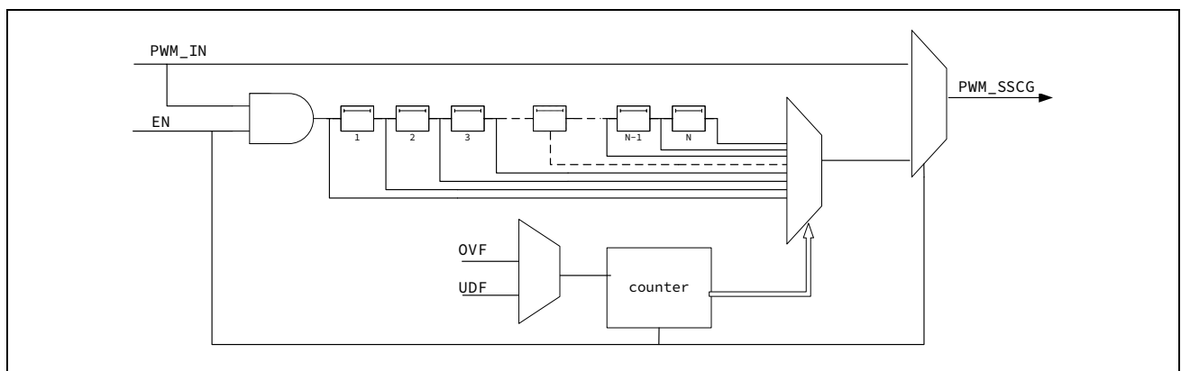
图 16-10 PWM 展频输出示意图
