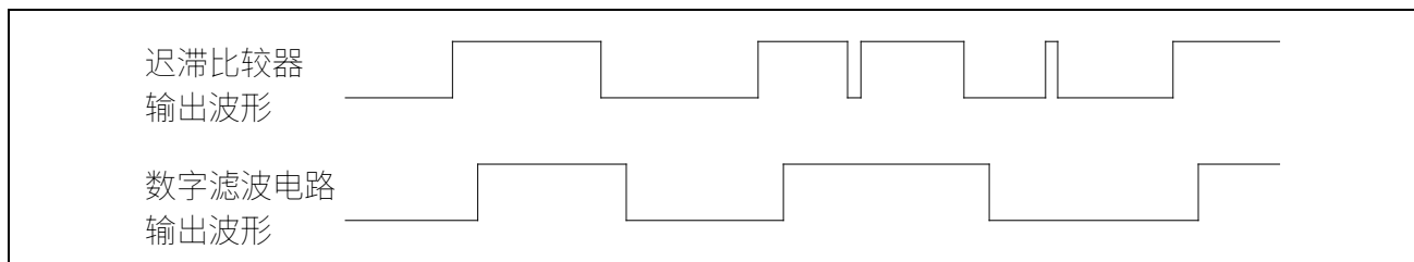
图 29-3 LVD 滤波输出
