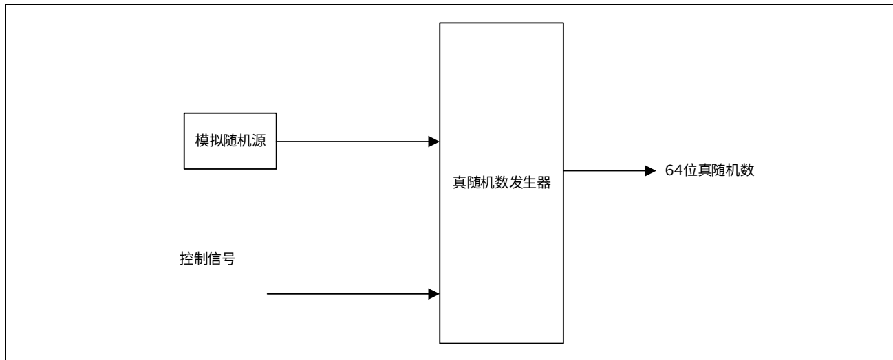
图 23-1 TRNG 数据流
