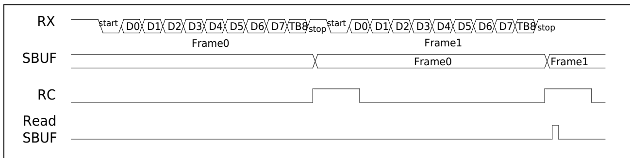
图 21-13 接收缓存
