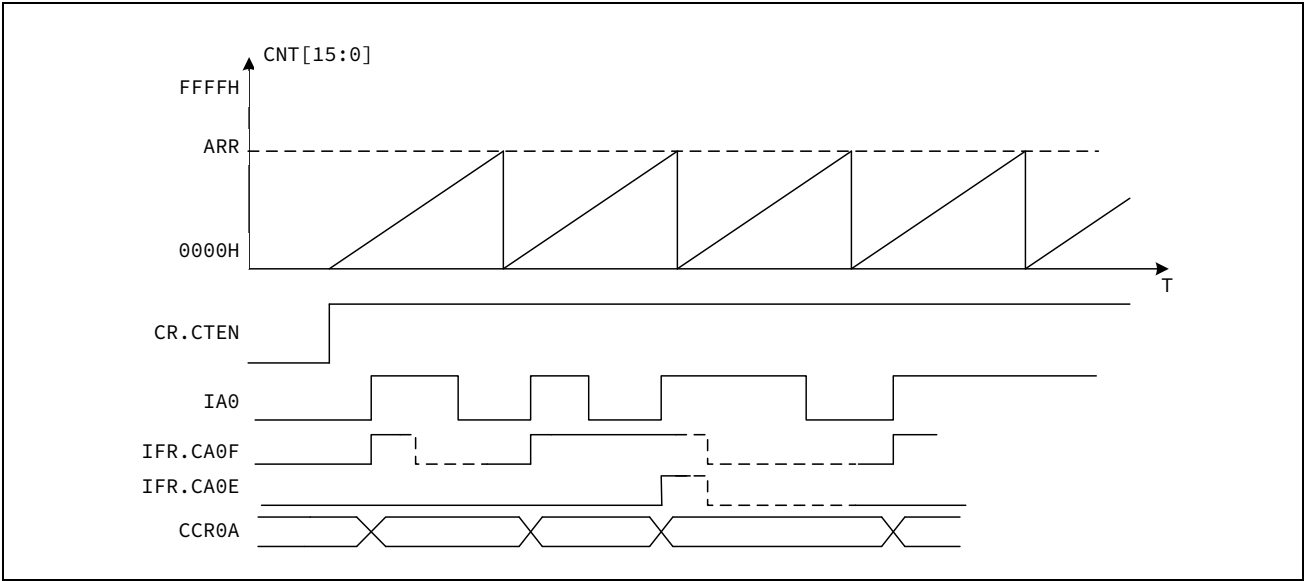
图 13-48 捕获时序图
