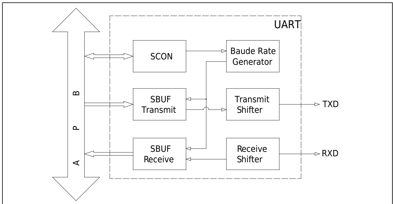
图 20-1 结构框图
