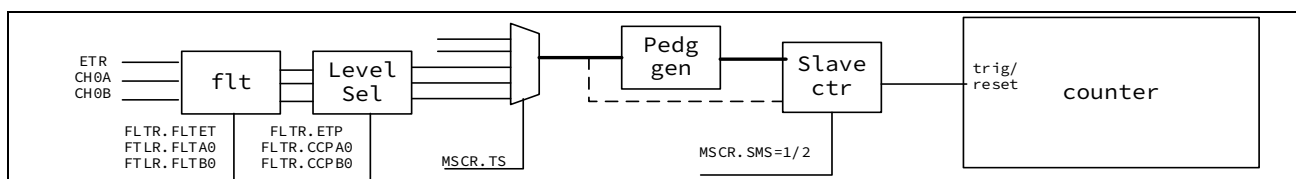
图 13-53 触发和复位功能
