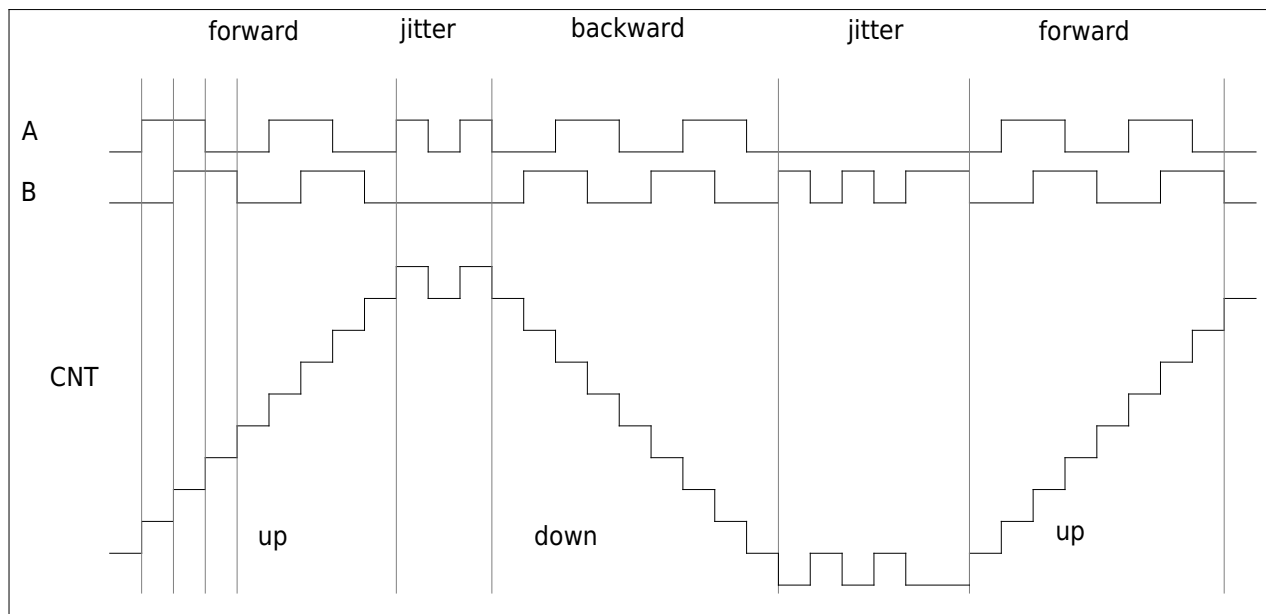
图 13-54 编码计数
