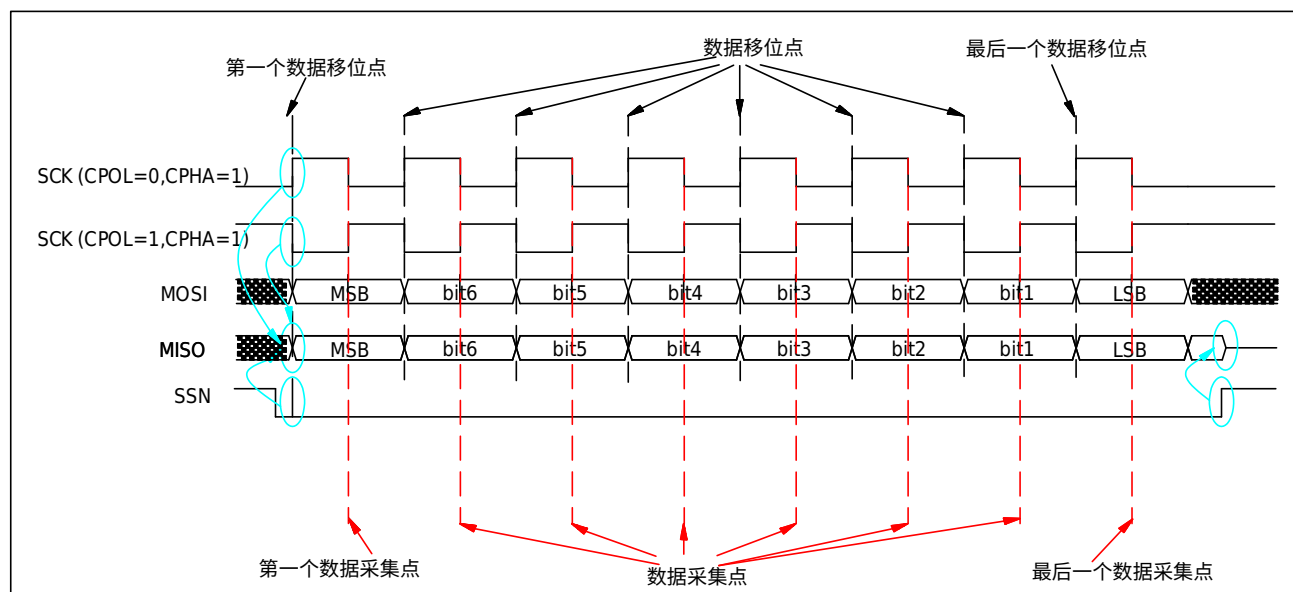
图 8-5 从机 CPHA 为 1 时数据帧格式
