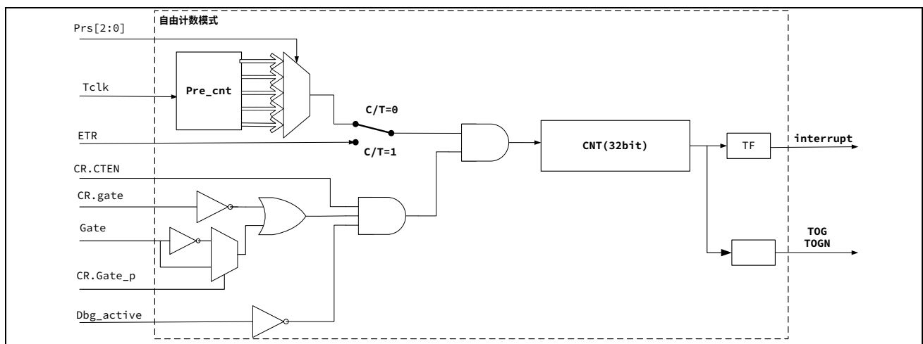
图 13-3 自由计数框图
