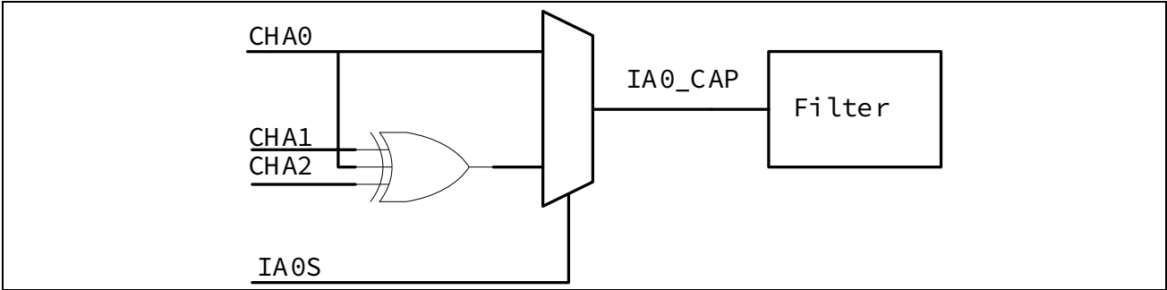
图 13-49 CHA 端口选择
