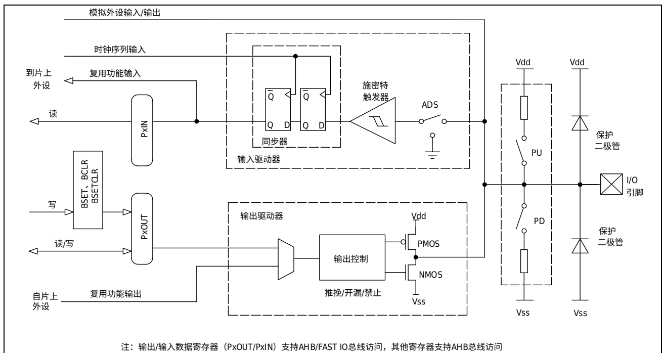
图 6-1 端口电路图
