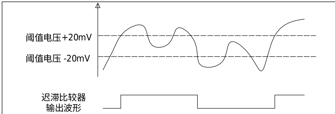
图 29-2 LVD 迟滞响应
