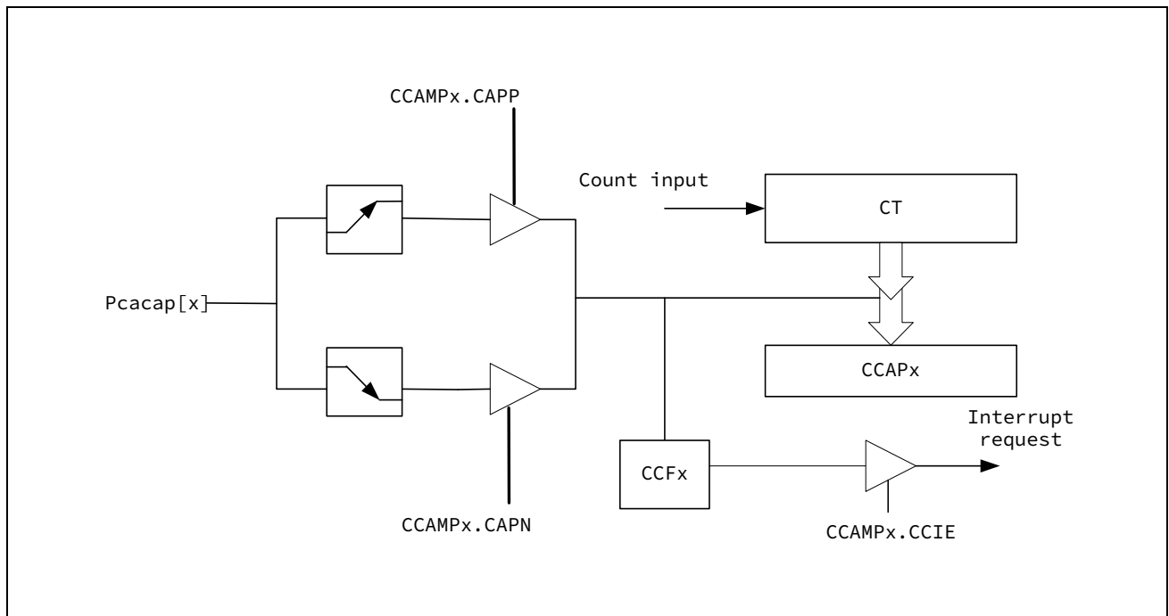
图 15-3 PCA 捕获功能框图
