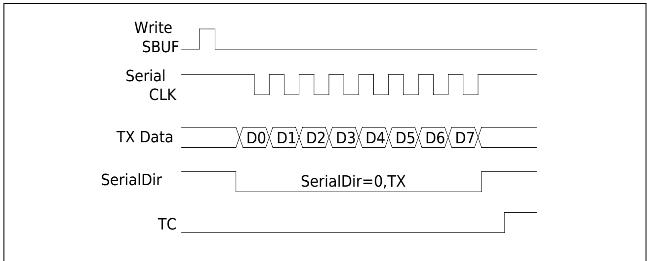
图 21-2 Mode0 发送数据
