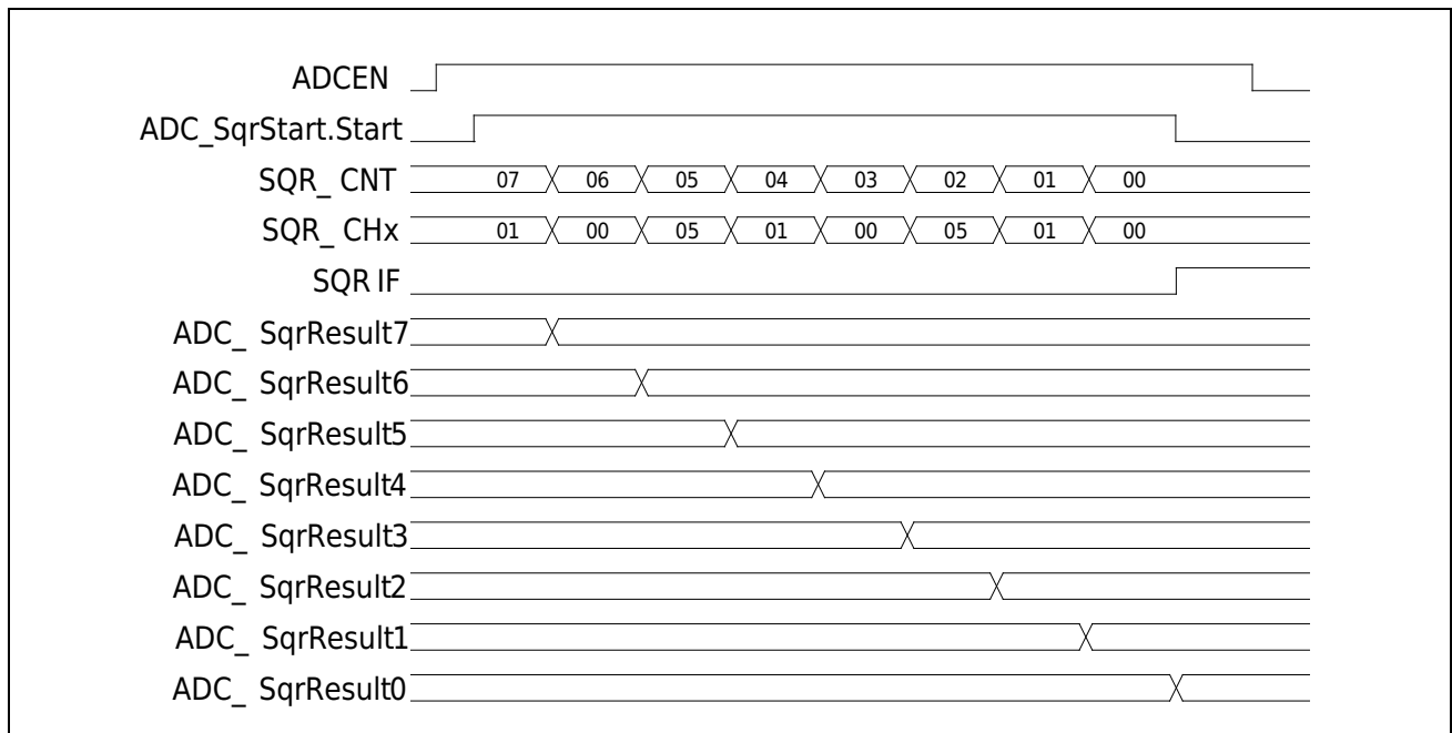
图 26-3 ADC 顺序扫描转换过程示例
