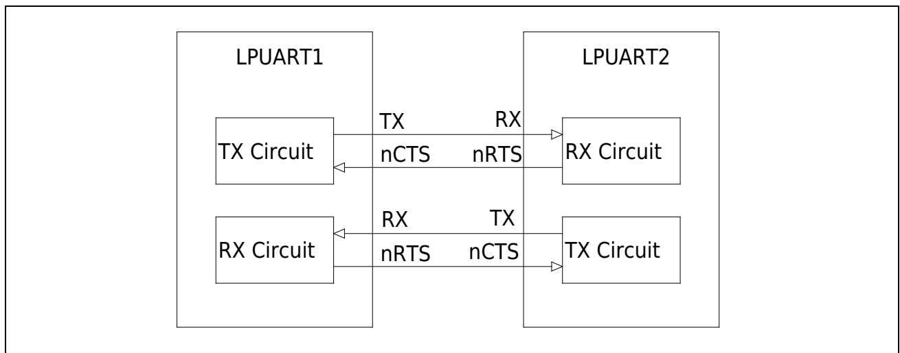
图 21-10 LPUART 硬件流控
