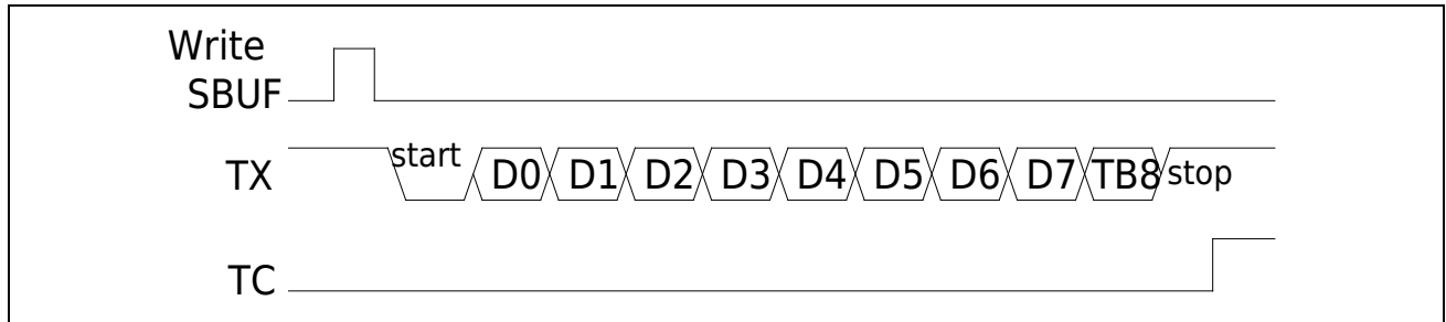
图 20-6 Mode2 发送数据
