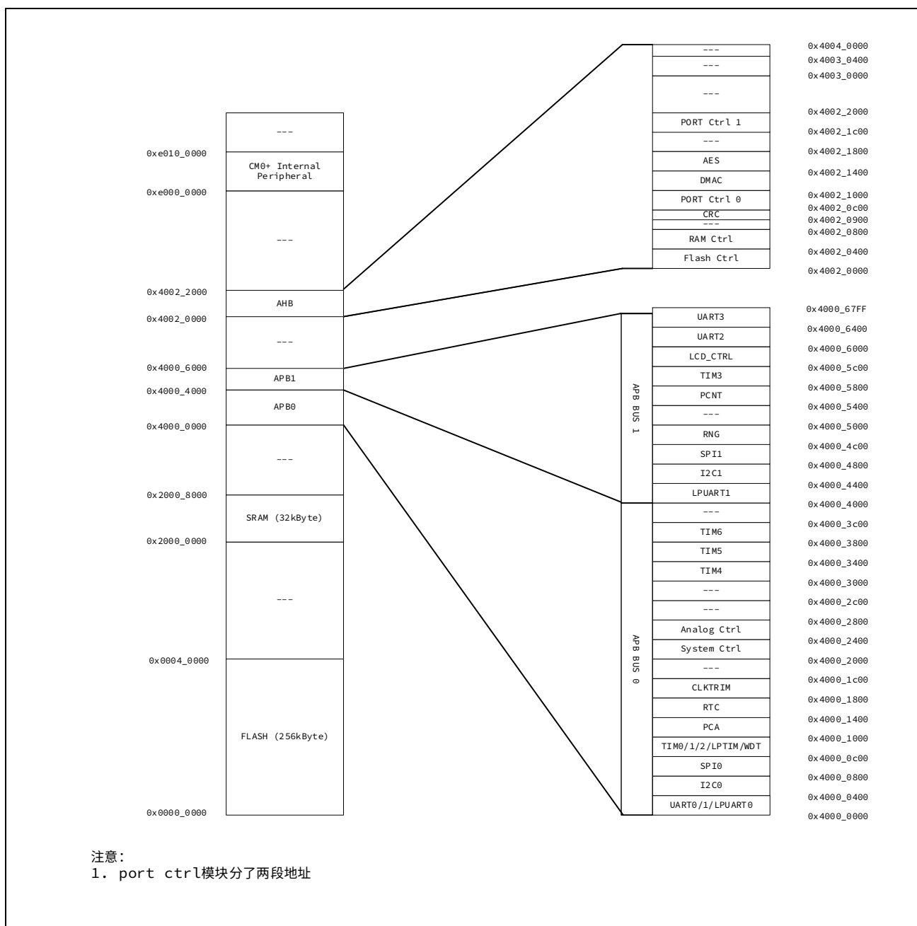
图 1-2 地址区域划分示意图
