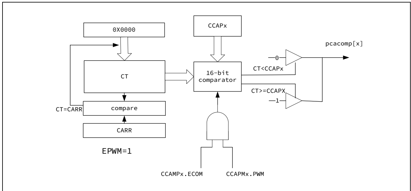
图 15-5 PCA 16 位 PWM 功能框图
