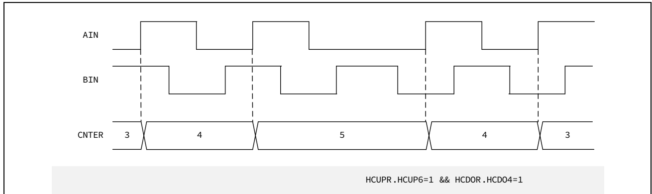
图 16-17 位置模式时相位差计数动作设定 (1 倍)
