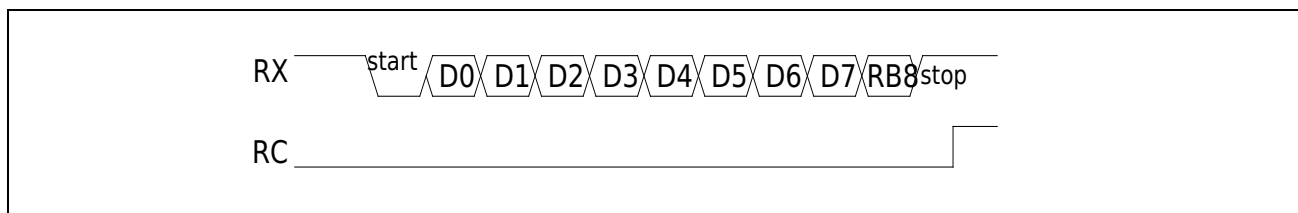
图 21-7 Mode2 接收数据
