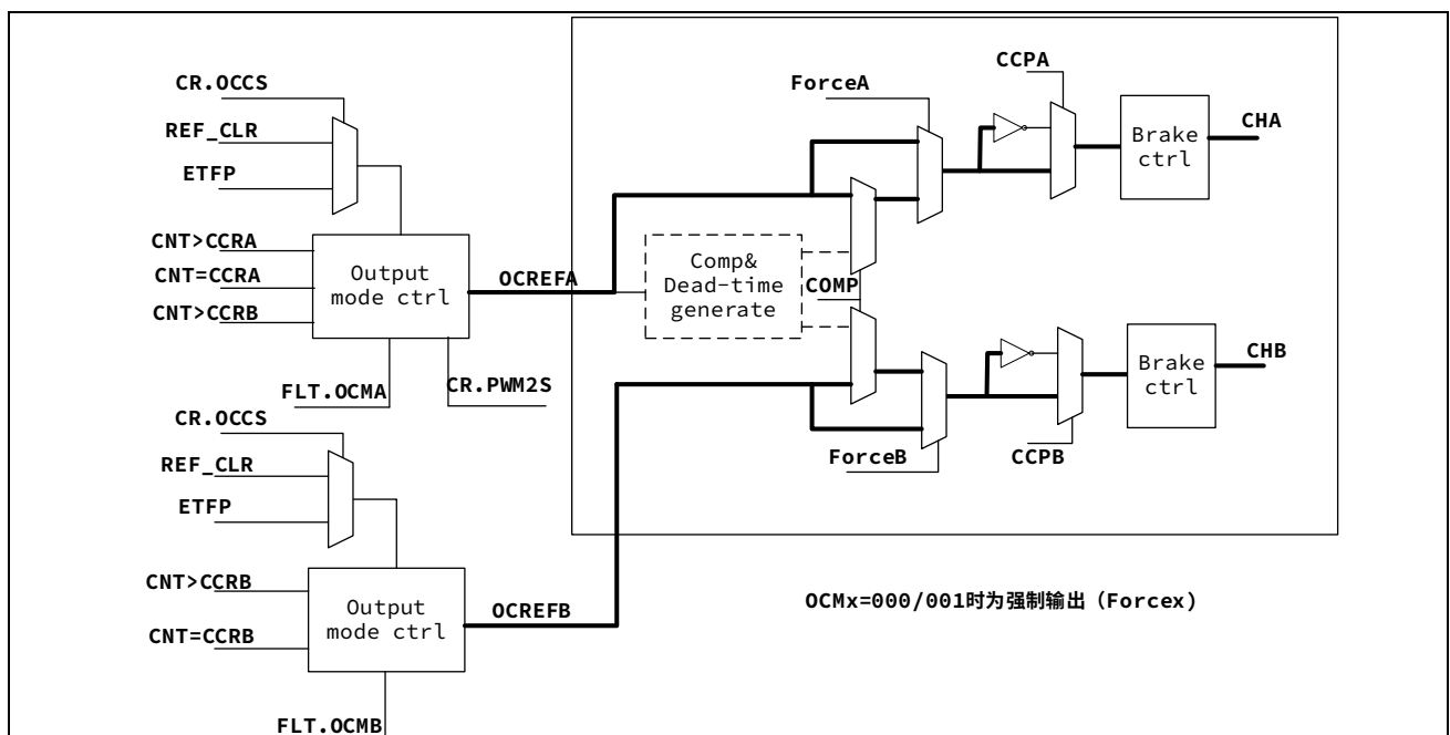
图 13-36 独立 PWM 输出框图
