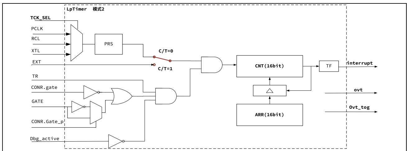
图 14-3 LPTimer 模式 2
