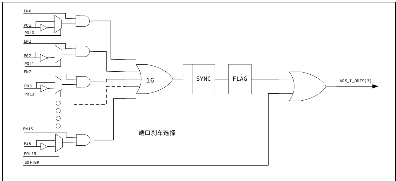
图 16-27 端口刹车与软件刹车示意图
