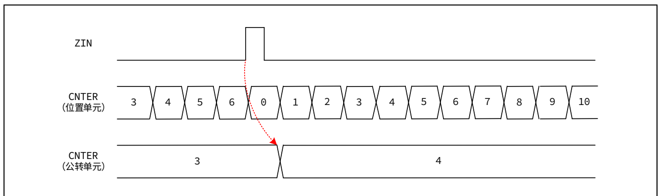
图 16-21 公转模式时 Z 相计数动作
