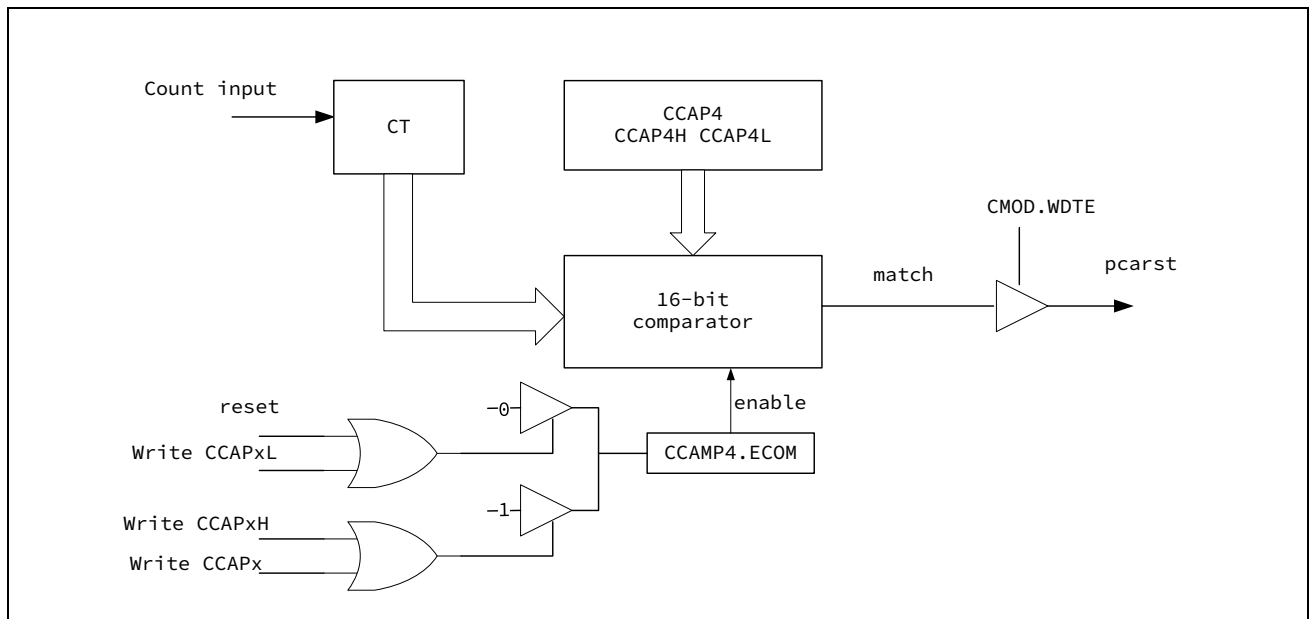
图 15-6 PCA WDT 功能框图
