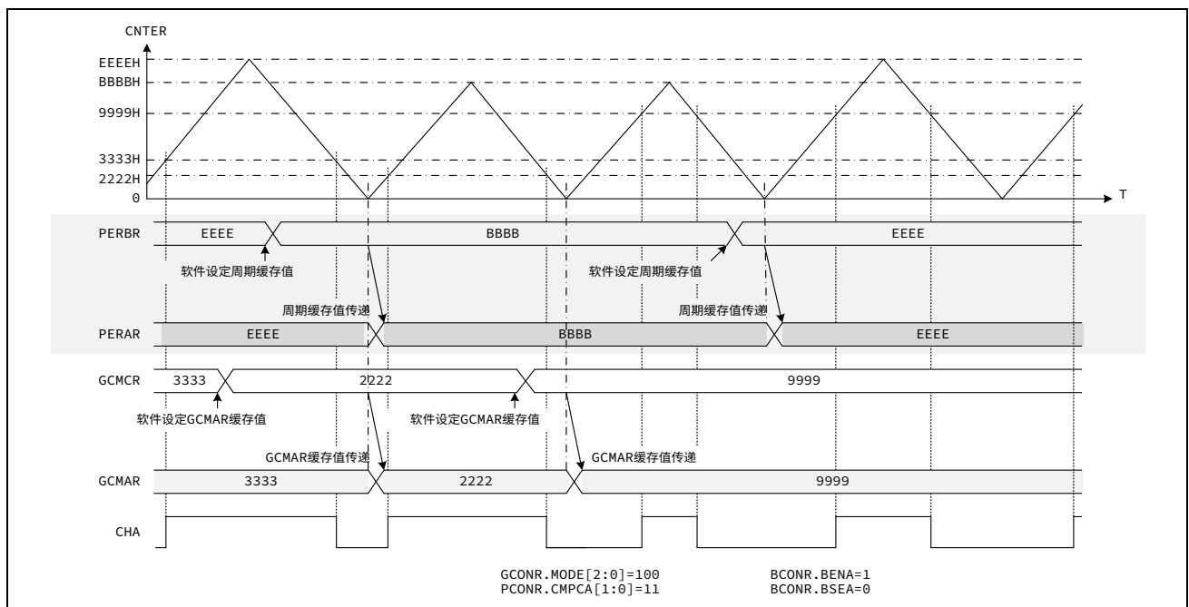
图 16-9 单缓存方式比较输出时序
