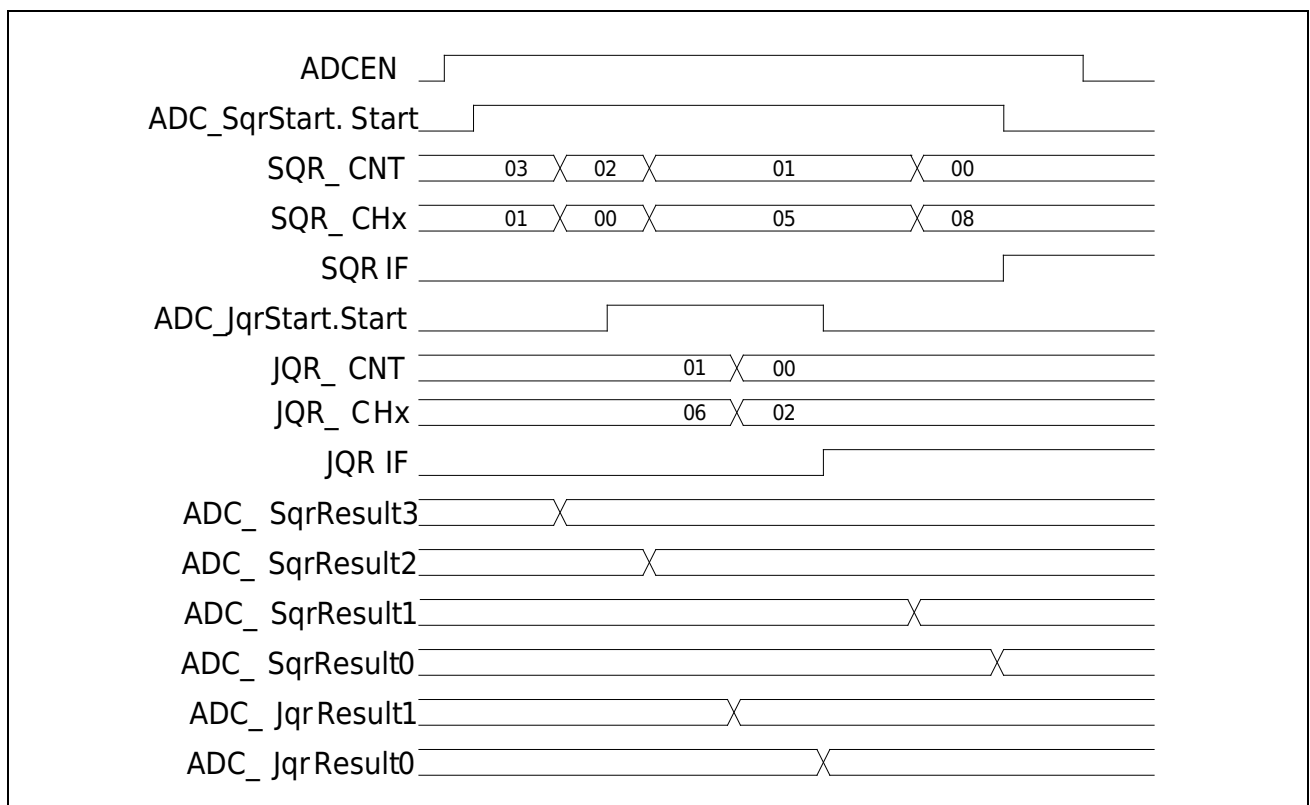
图 26-5 ADC 顺序扫描过程中进行插队扫描示例
