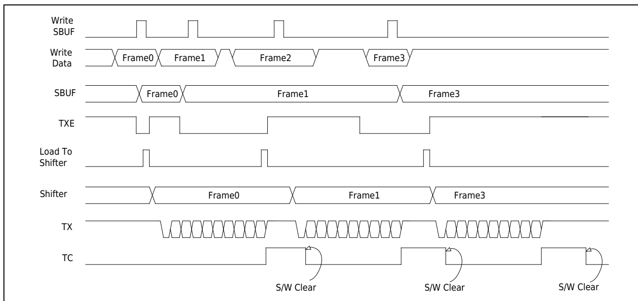
图 20-14 发送缓存
