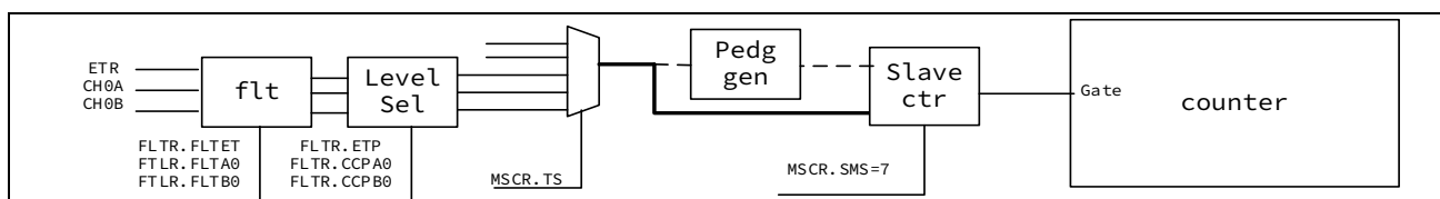
图 13-52 门控功能
