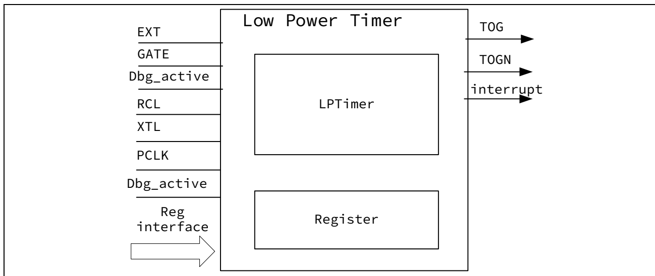
图 14-1 LPTimer 框图
