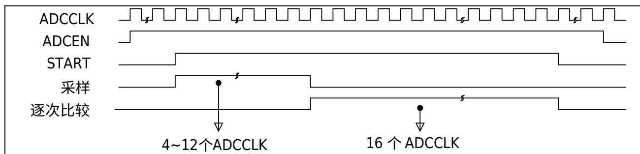
图 26-2 ADC 转换时序图
