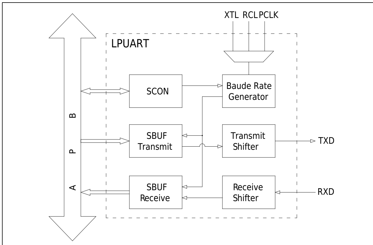
图 21-1 结构框图
