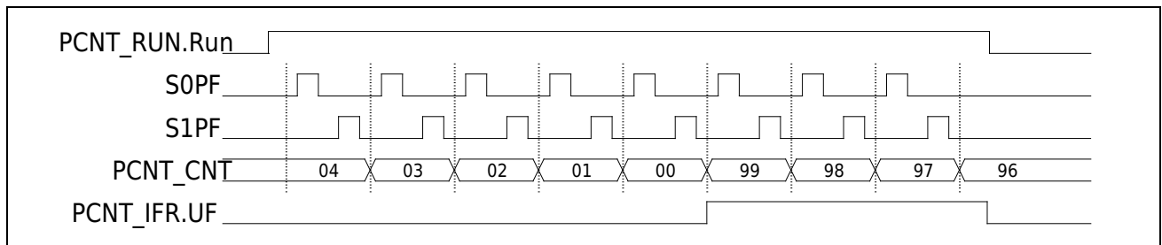
图 19-5 双通道非交脉冲计数模式减计数波形
