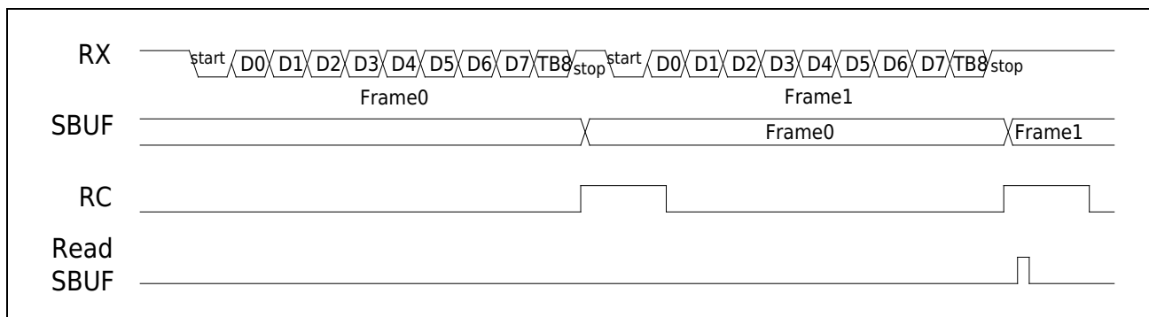
图 20-13 接收缓存
