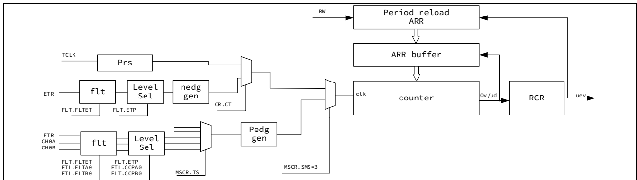
图 13-14 计数器框图
