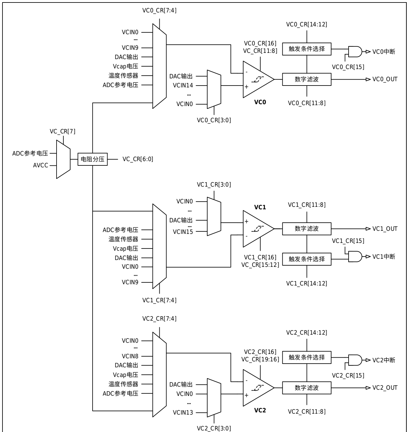
图 28-1 VC 框架图
