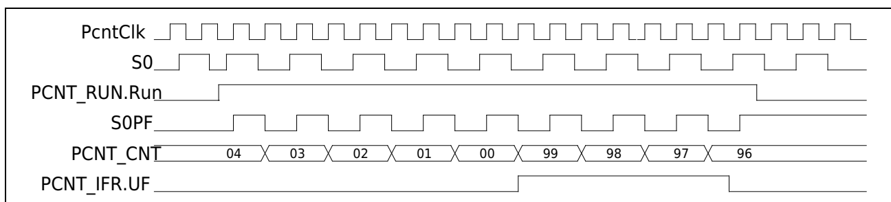
图 19-3 单通道脉冲计数模式减计数波形
