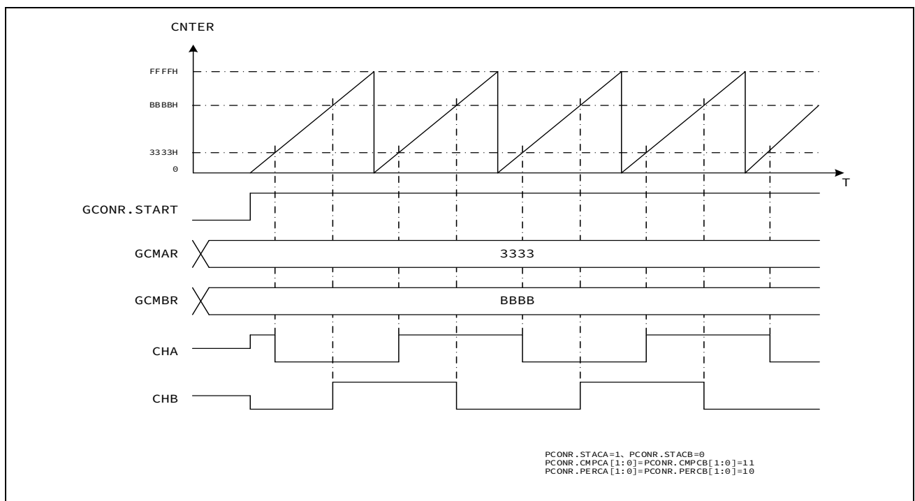
图 16-4 比较输出动作
