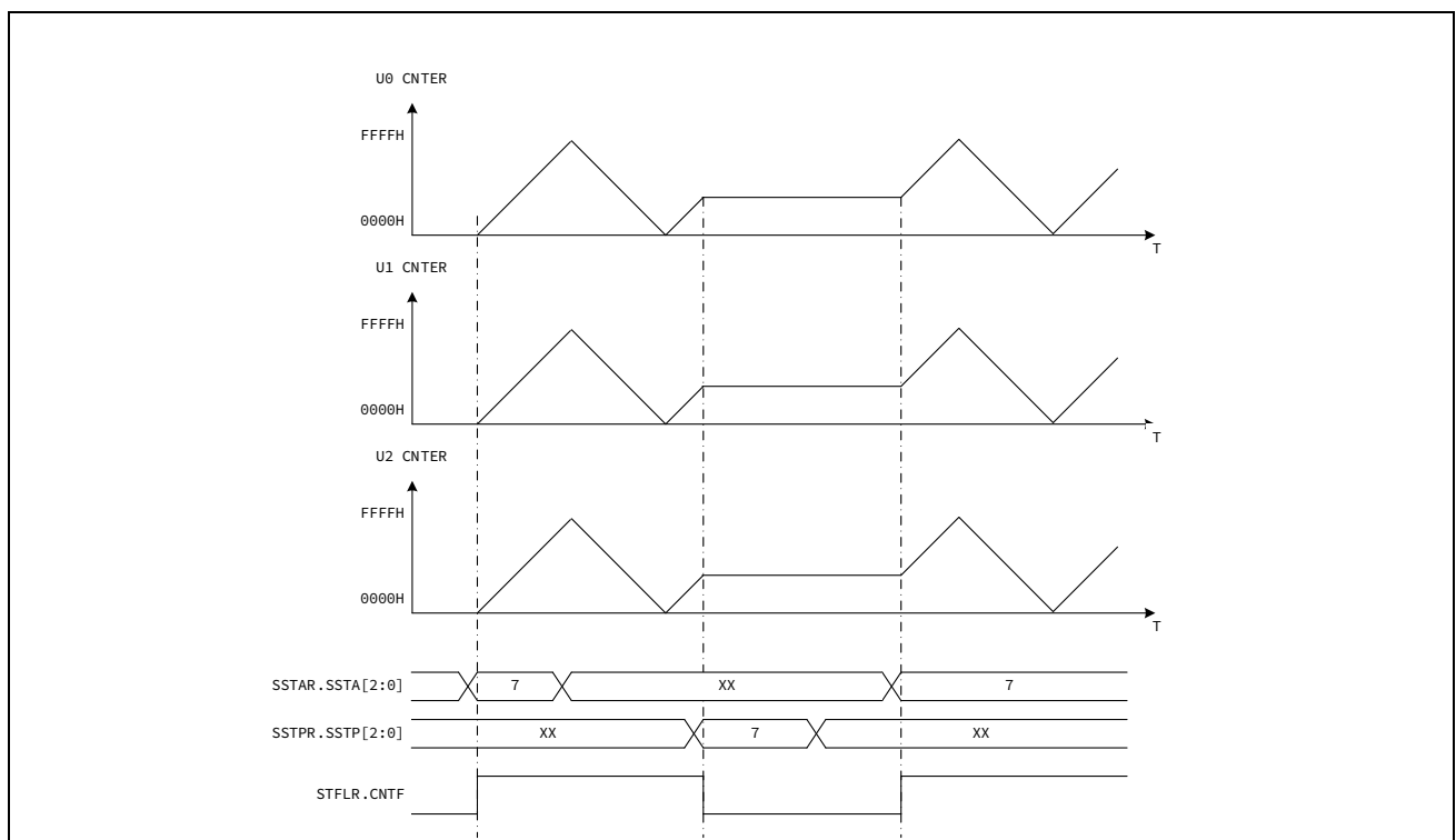
图 16-7 软件同步动作
