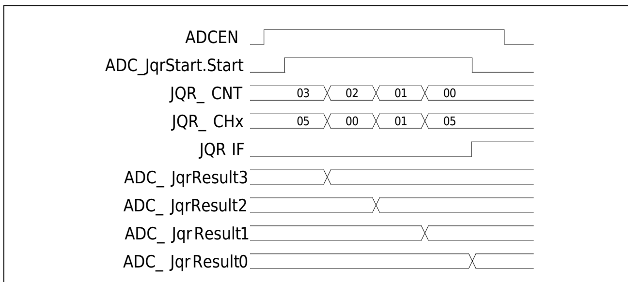
图 26-4 ADC 插队扫描转换过程示例
