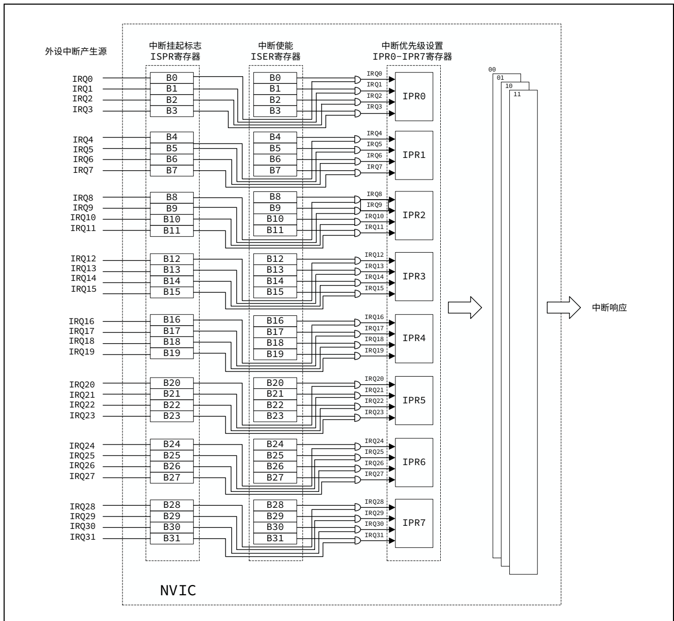
图 5-7 中断结构图
