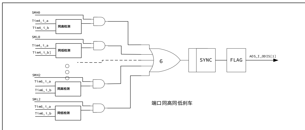
图 16-28 输出同高同低刹车示意图
