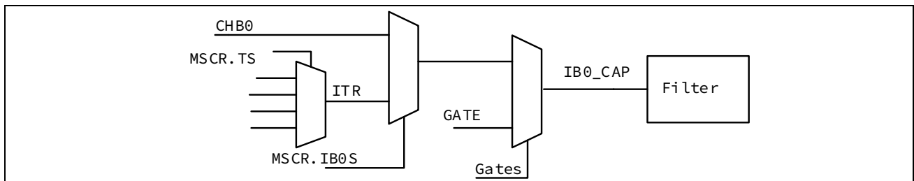
图 13-50 CHB 端口选择
