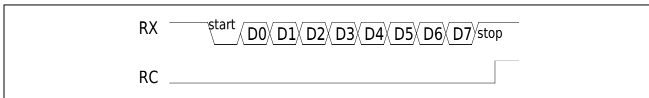
图 21-5 Mode1 接收数据
