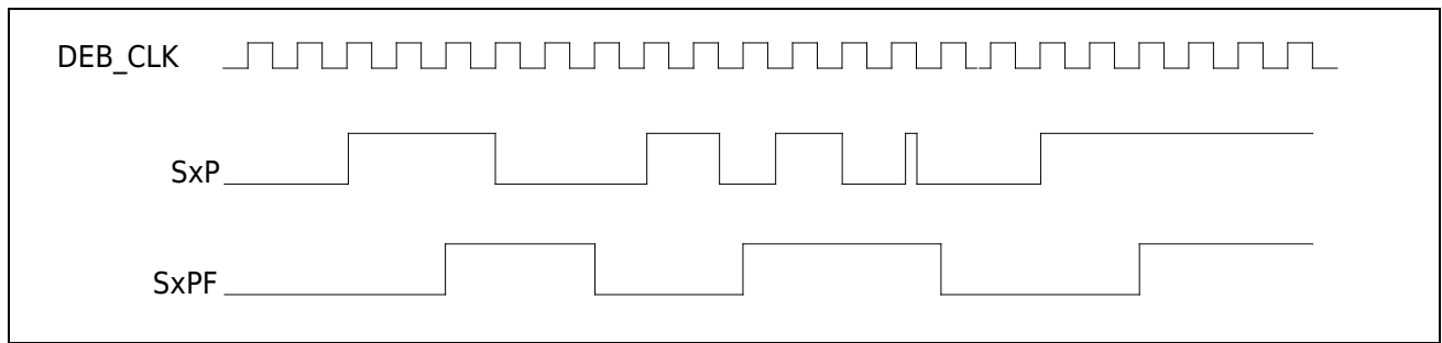
图 19-8 脉冲宽度滤波波形
