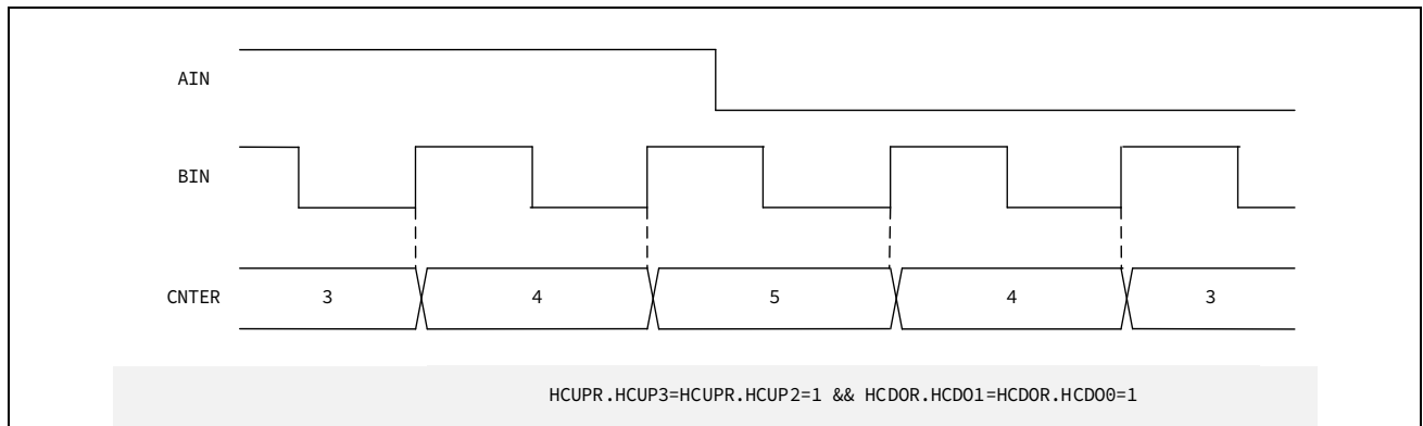
图 16-20 位置模式时方向计数动作
