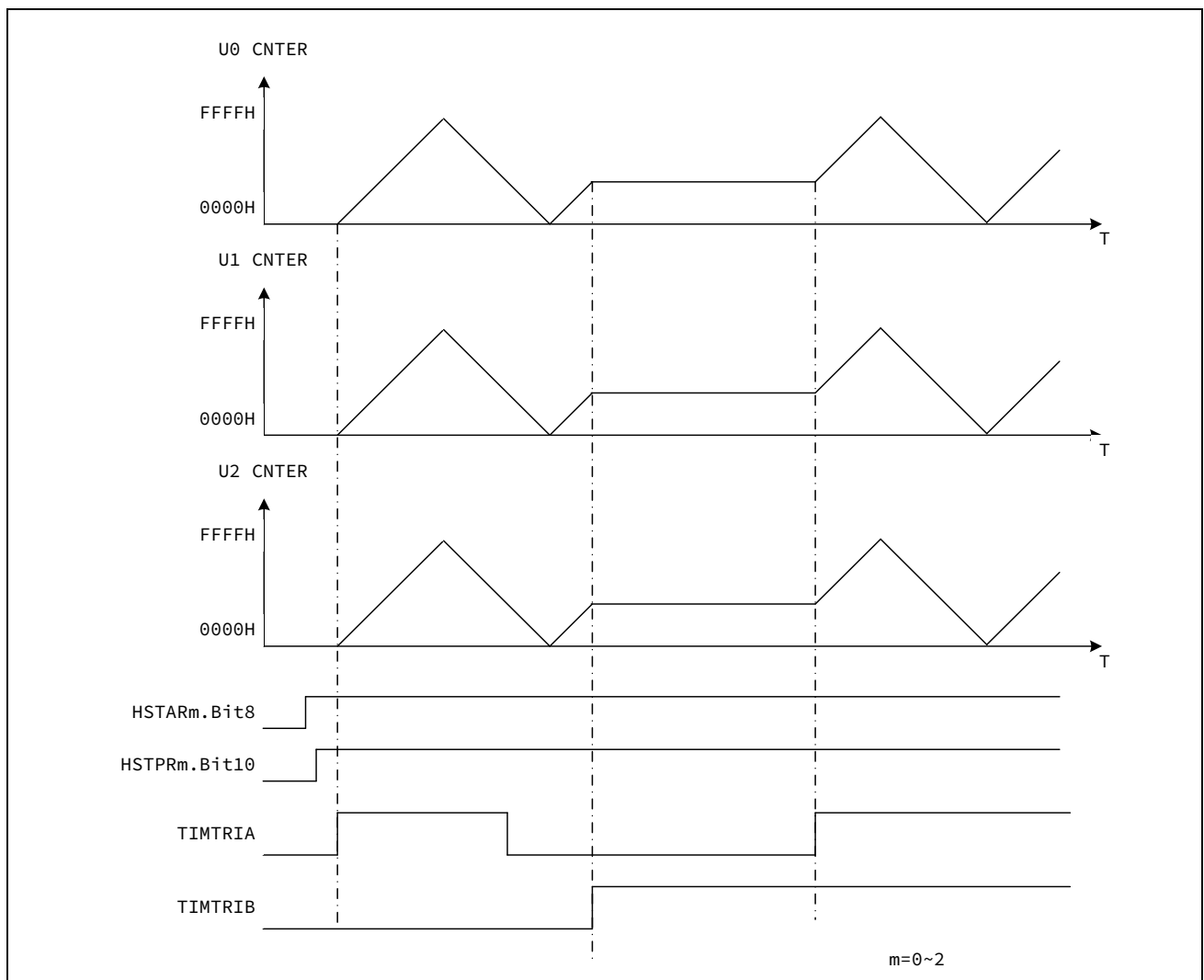
图 16-8 硬件同步动作
