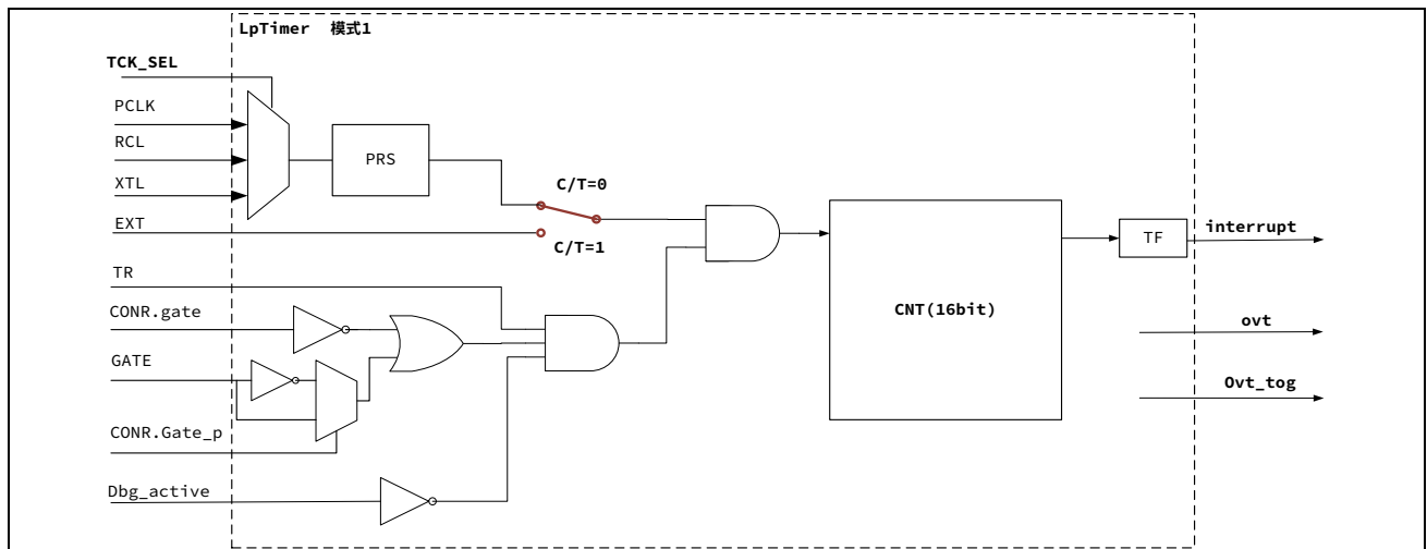
图 14-2 LPTimer 模式 1
