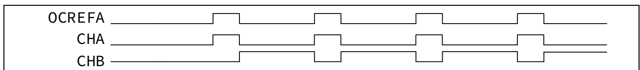
图 13-40 互补 PWM 输出波形图
