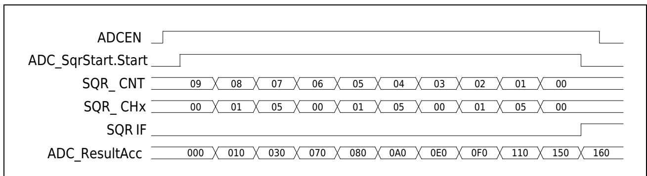
图 26-6 ADC 连续转换累加过程示例
