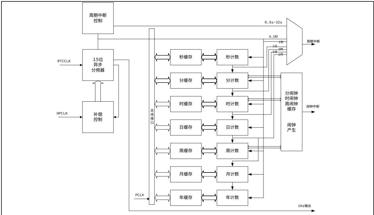
图 17-1 RTC 框图
