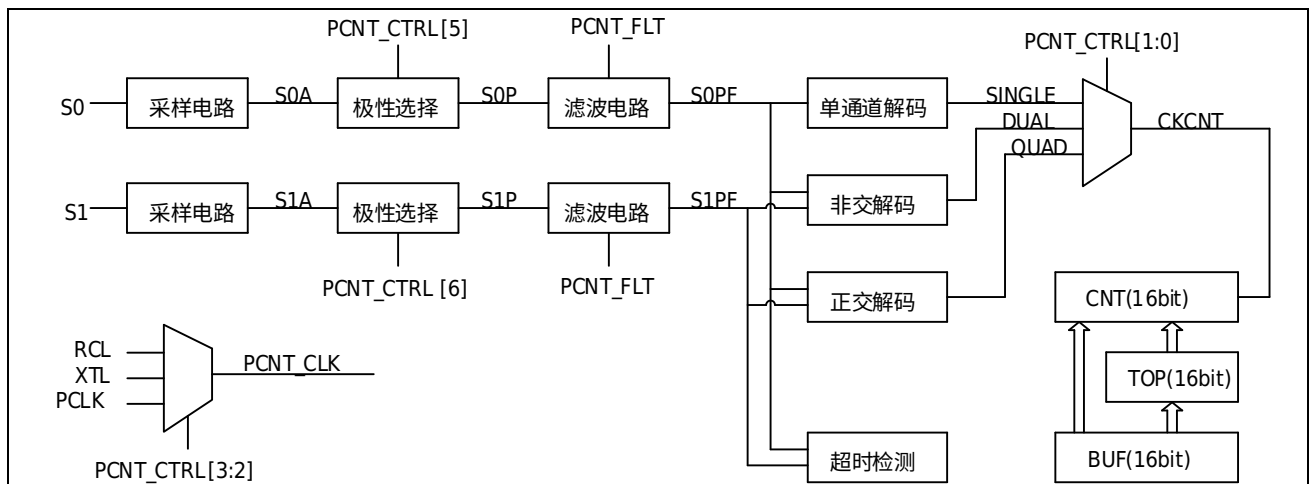
图 19-1 整体框图
