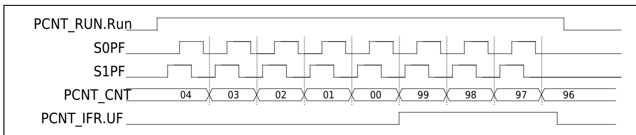
图 19-7 双通道正交脉冲计数模式减计数波形
