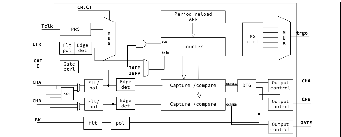
图 13-1 TIM0/1/2 框图
