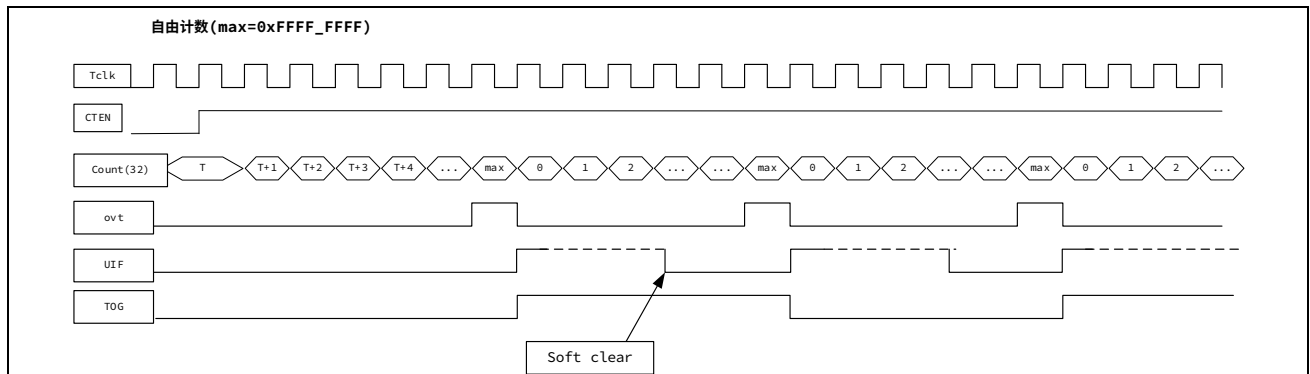
图 13-7 自由计数时序图
