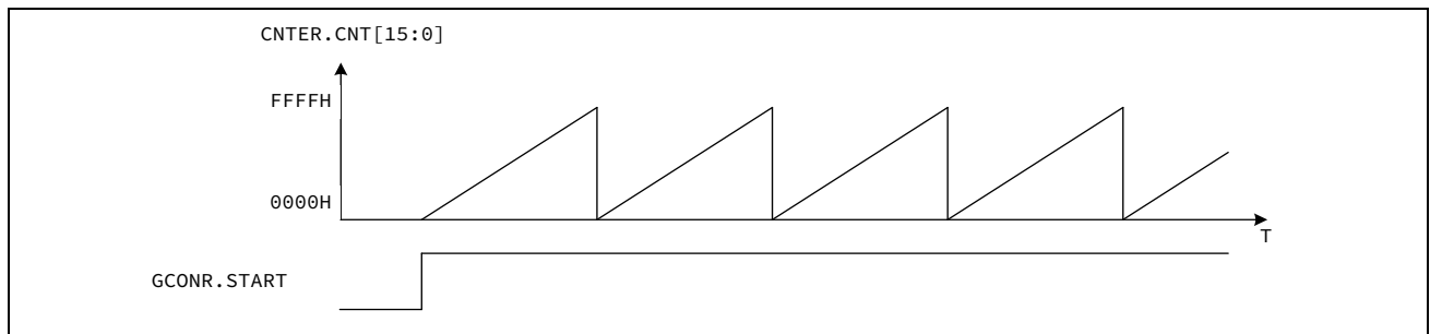
图 16-2 锯齿波波形（递加计数）
