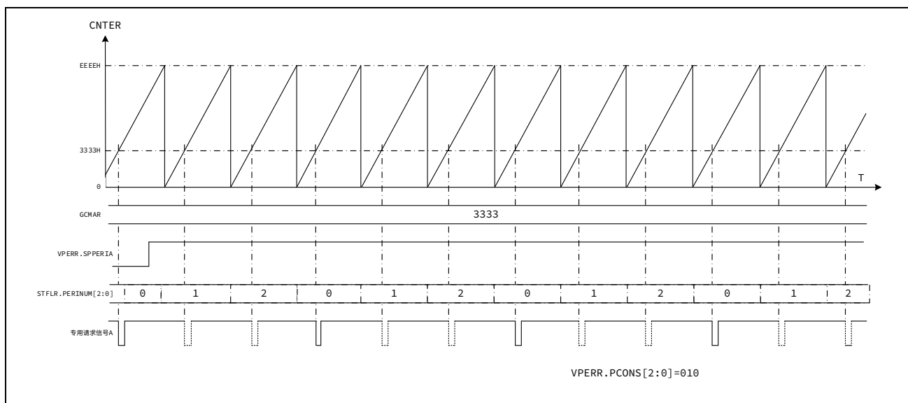
图 16-26 周期间隔有效请求信号动作
