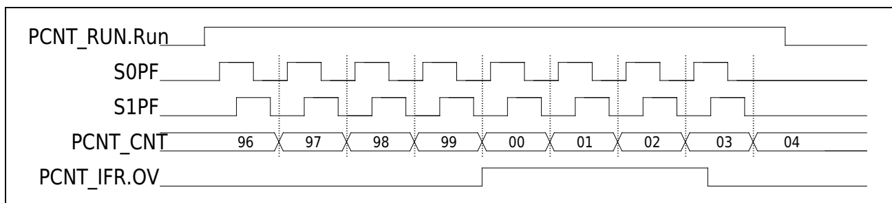
图 19-6 双通道正交脉冲计数模式加计数波形
