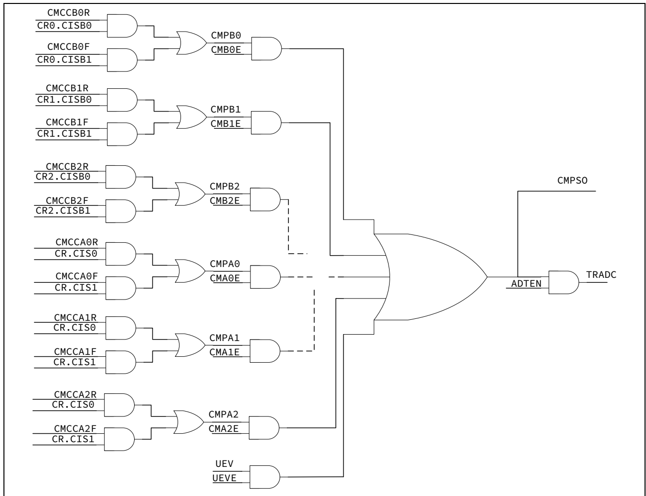
图 13-55 ADC 触发
