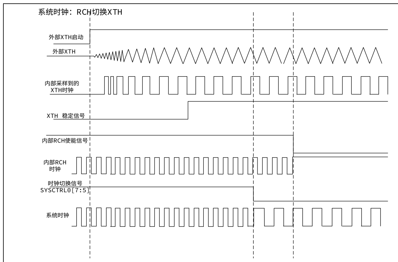
图 3-3 时钟切换示意图
