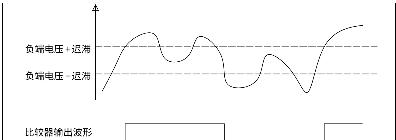
图 28-3 VC 迟滞功能
