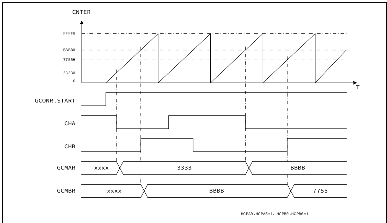
图 16-5 捕获输入动作
