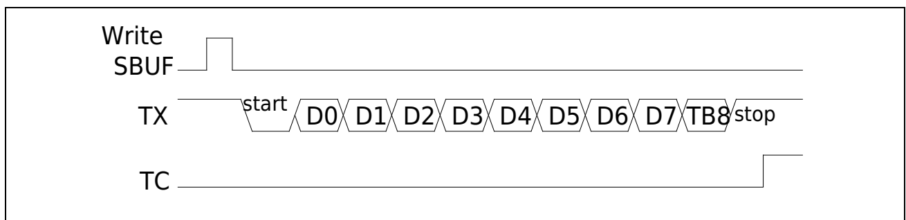
图 20-8 Mode3 发送数据
