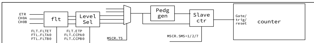
图 13-51 从模式示意图
