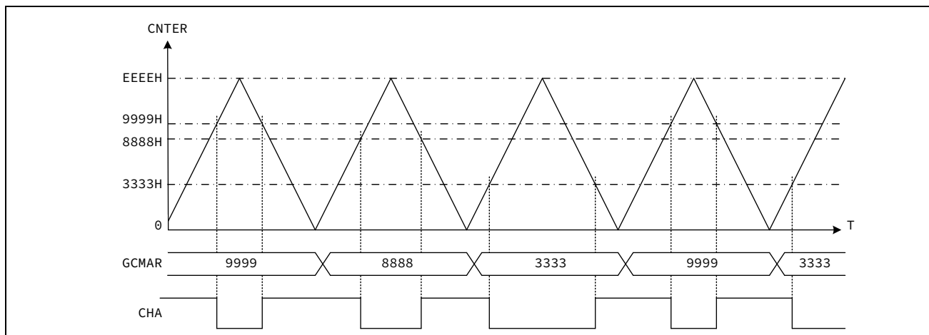
图 16-11 CHA 输出 PWM 波
