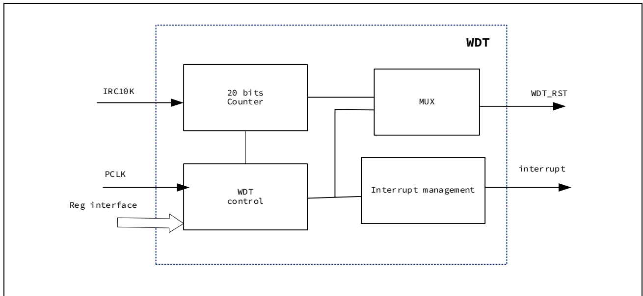
图 18-1 WDT 整体框图
