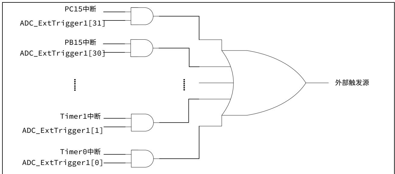
图 26-8 ADC 插队扫描转换外部触发源示意图
