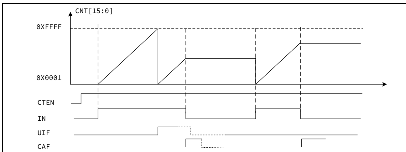
图 13-10 高电平脉冲宽度测量
