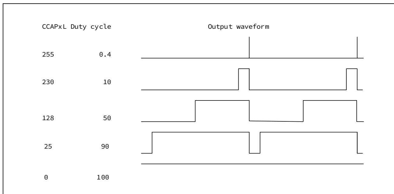
图 15-8 PCA PWM 输出波形
