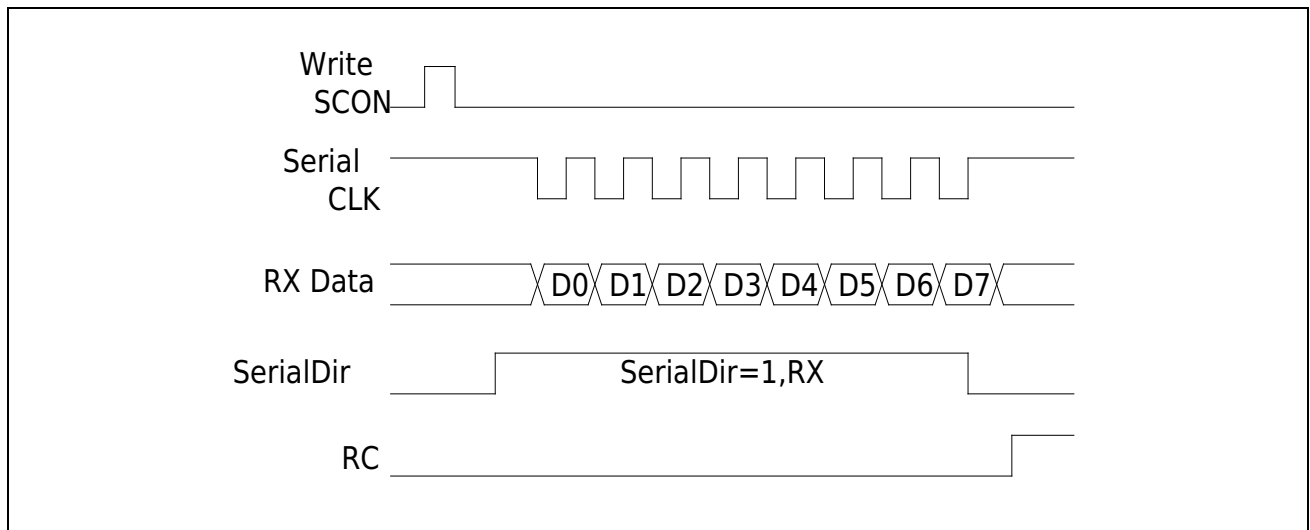
图 21-3 Mode0 接收数据
