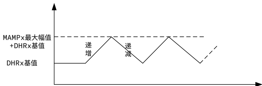
图 27-3 生成 DAC 三角波
