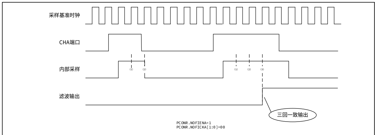
图 16-6 捕获输入端口的滤波功能
