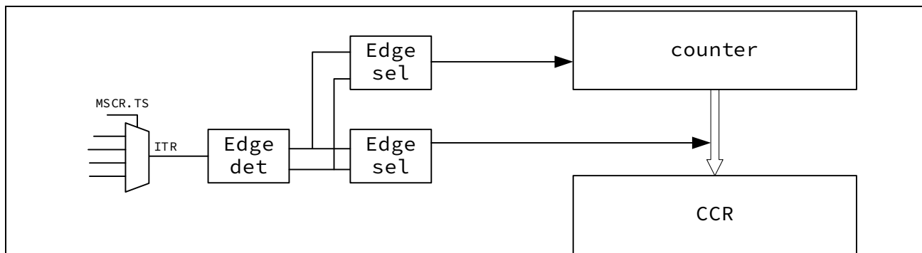
图 13-9 PWC 测量框图
