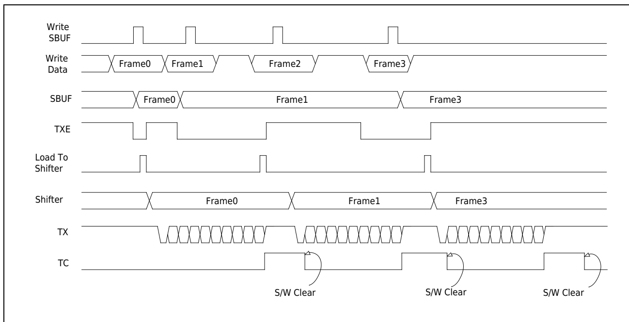
图 21-14 发送缓存
