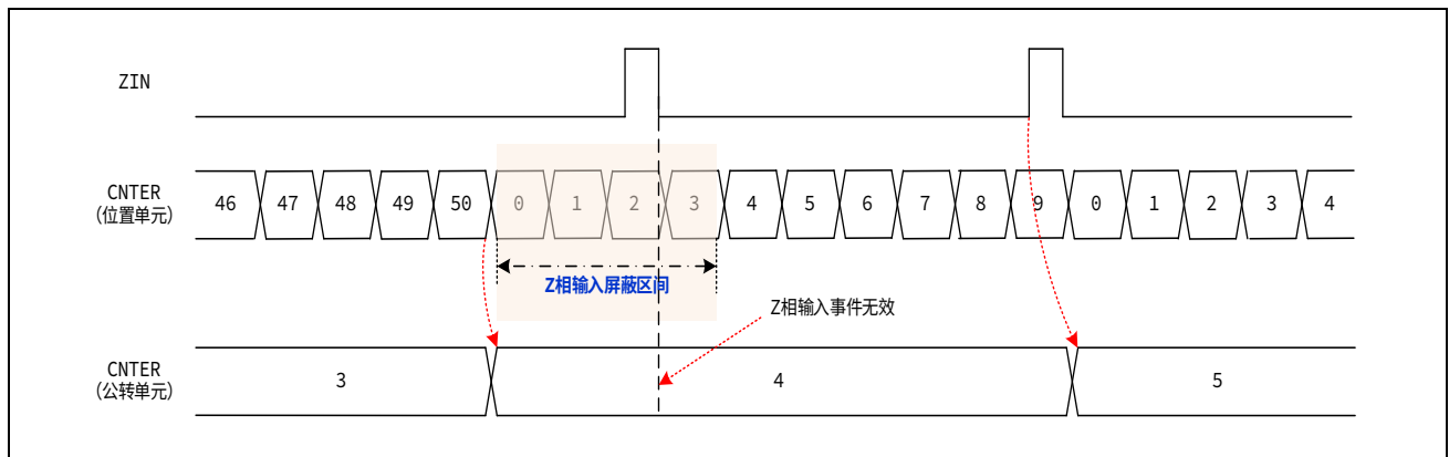
图 16-24 公转计数模式-混合计数 Z 相屏蔽动作例 1
