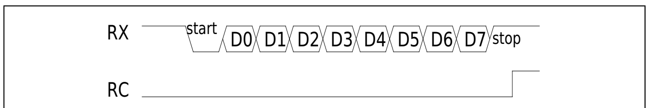
图 20-5 Mode1 接收数据
