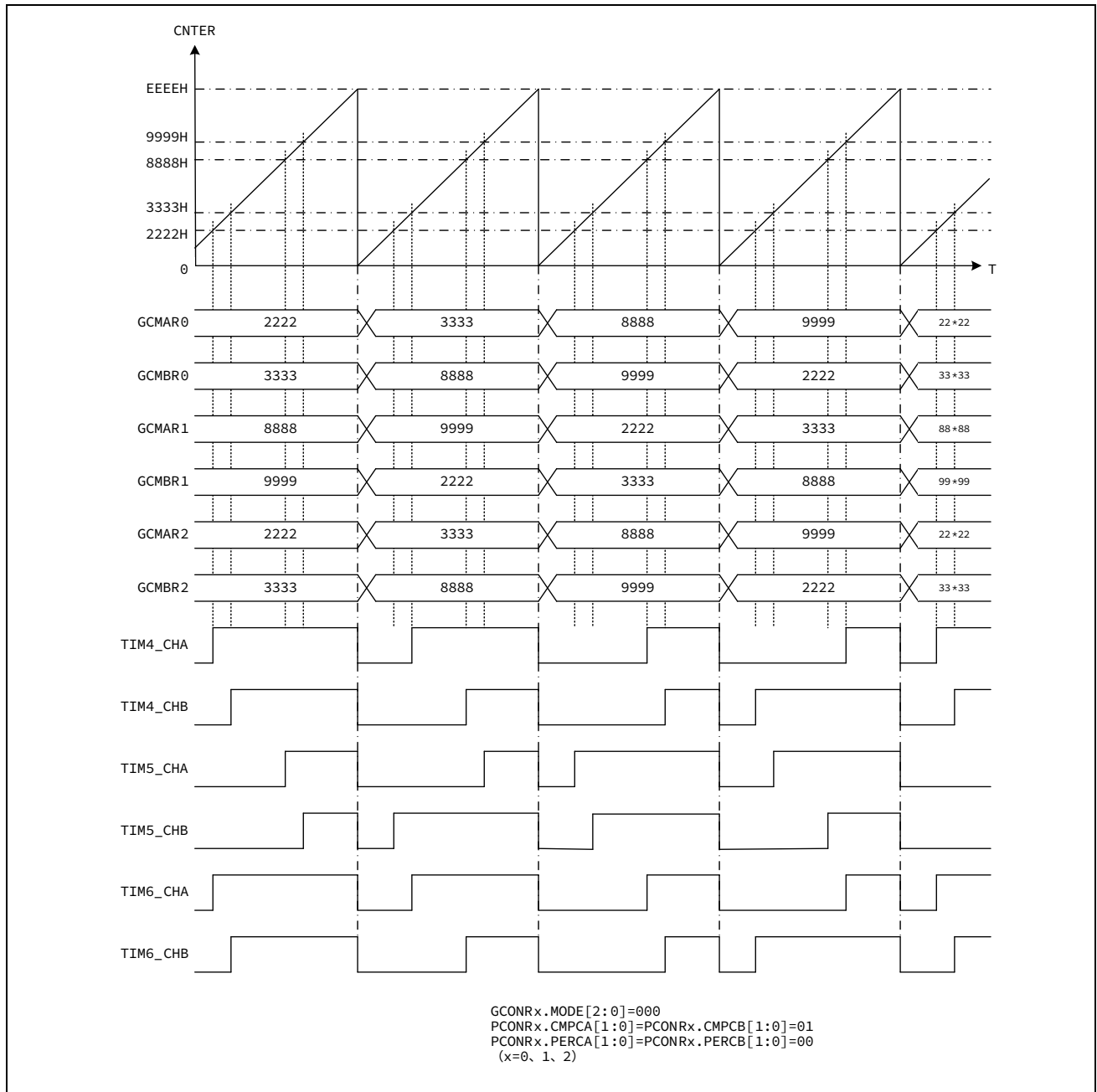
图 16-14 6 相 PWM 波
