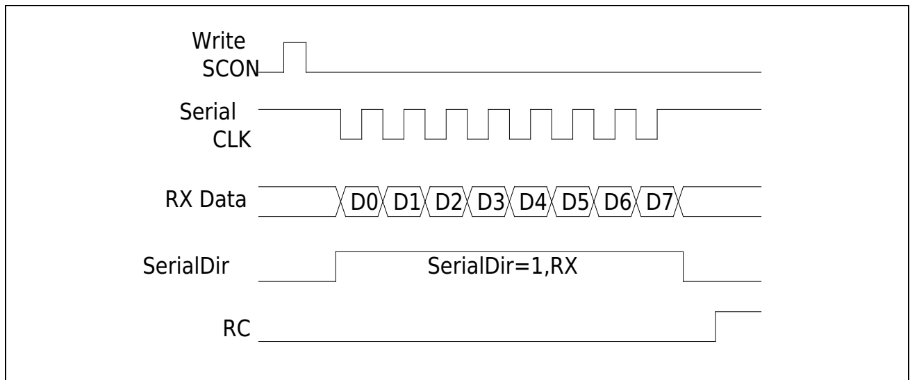
图 20-3 Mode0 接收数据
