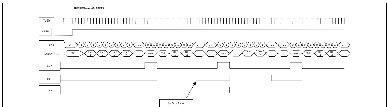
图 13-8 重载计数时序图（预分频设置为 2）
