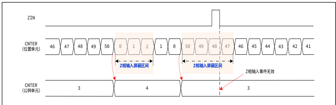
图 16-25 公转计数模式-混合计数 Z 相屏蔽动作例 2
